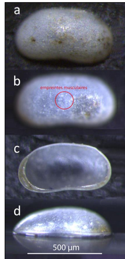
Fig. 74 – Fossiles de Candona neglecta (Sars, 1887). Individus prélevés à 195 cm ( b et d ) et 500 cm ( a et c ) de profondeur dans le sondage LG13T3. Cette espèce vit dans des sédiments vaseux et occupe les étangs d'eau douce, les marais, les fossés et les ruisseaux oligohalines (Henderson, 1990). Avec a : Vue externe d'une valve gauche adulte ; b : Vue externe d'une valve droite adulte ; c : Vue interne d'une valve droite adulte ; d : Profil d'une valve gauche adulte.
