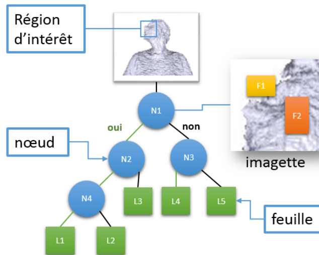
FIGURE 1.3 – Représentation d'un arbre de profondeur d_{RF} = 3 . Les ronds bleus représentent les nœuds. Les carrés verts représentent les feuilles. L'image représente l'extraction des descripteurs (différence d'intensité entre le rectangle F1 et F2) lors du passage dans le premier nœud.
