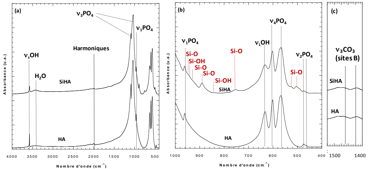
Figure II-7 : Spectres FT-IR dans les intervalles (a) 4000-400 \text{cm}^{-1} , (b) 1000-400 \text{cm}^{-1} et (c) 1500-1400 \text{cm}^{-1} des poudres d'HA et de SiHA calcinées à 1000°C/1 h. Les indexations représentées en noir sont communes aux spectres d'HA et SiHA, les indexations en rouge sont spécifiques aux spectres de SiHA
