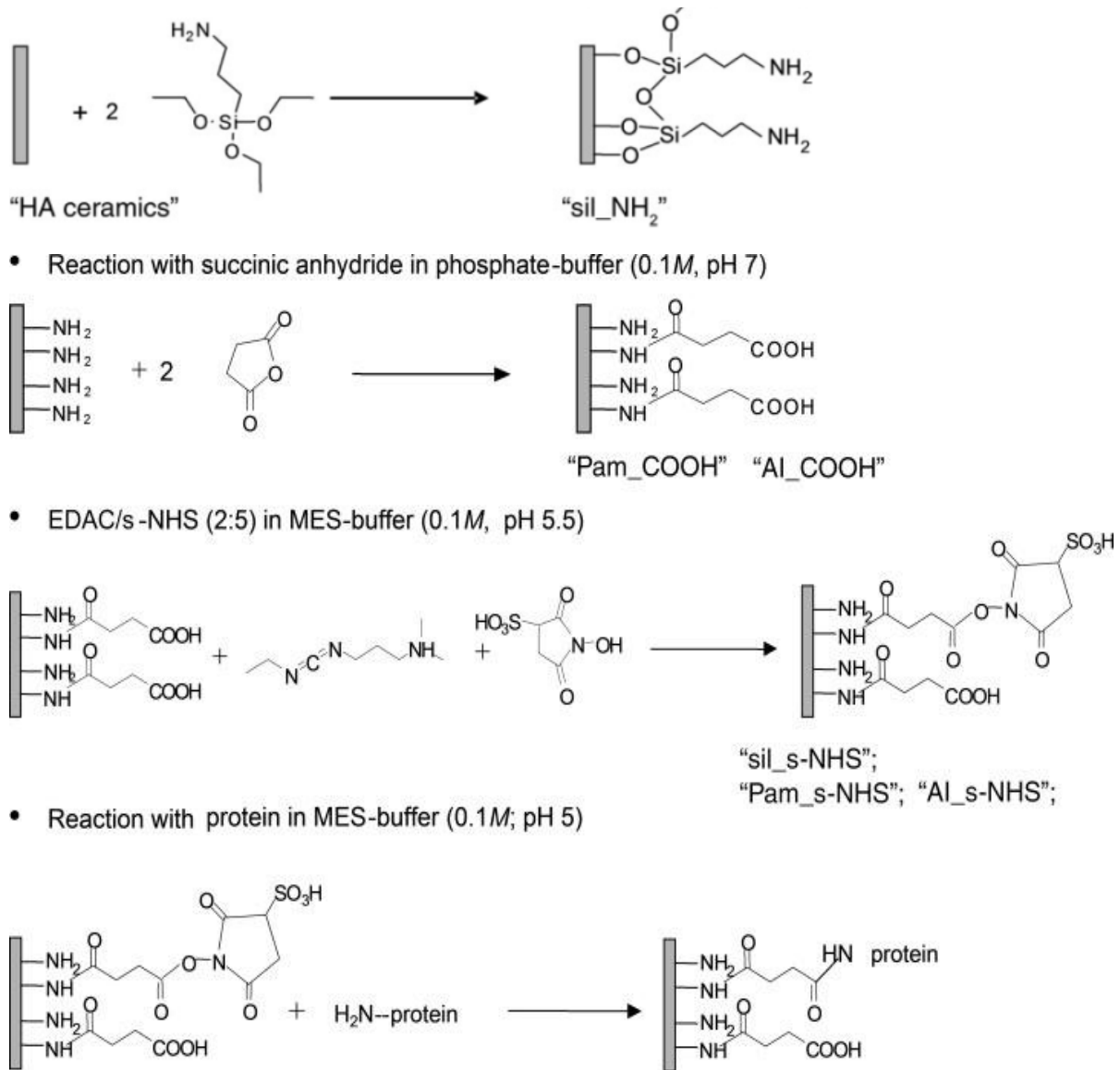
Figure I-29 : Procédé de silanisation d’HA par de l’APTES établi par Schuessele et al. [105]
