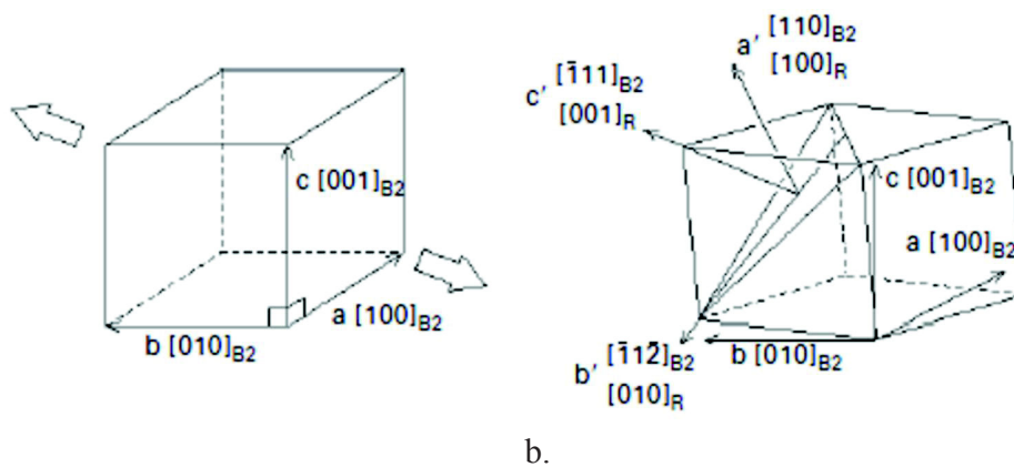
Figure 1.4: a. Structures cristallines austénitique (B2), martensitique (B19') et la correspondance de maille entre ces deux phases (Miyazaki et al. 2009); b. Structure cristalline de la phase R.
