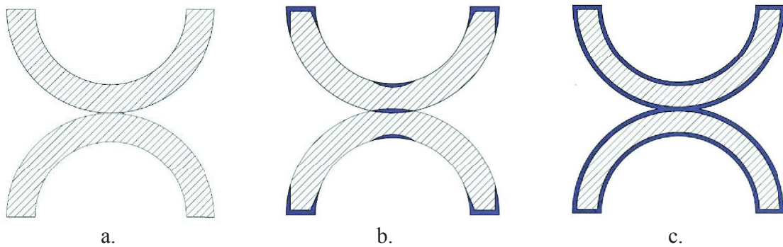
Figure 2.30: Distribution de la phase gris foncé ( Ti_2NiO ) suivant l'augmentation de la durée de frittage; a. Échantillon initial; b. Frittage court; c. Frittage long.
