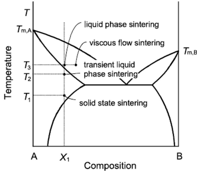
Figure 2.3: Illustration des différents types de frittage.
