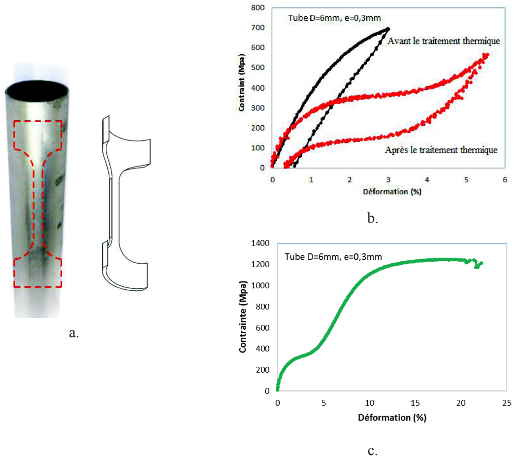
Fig 4.1: Influence du traitement de vieillissement (350°C, 1 heure) sur le comportement mécanique du tube de TiNi (Alonso et al. 2014); a. Epreuve de traction usinée par électroérosion; b: essais de traction à 20°C de type charge-décharge avant (courbe noire) et après traitement (courbe rouge) ; (c) essai de traction à rupture sur épreuve traitée.
