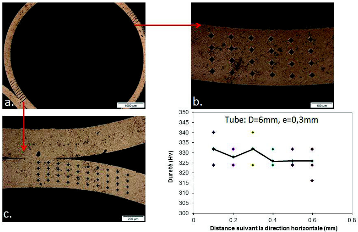
Figure 4.23 : La mesure de dureté du tube D=6\text{mm} , e=0,3\text{mm} .
