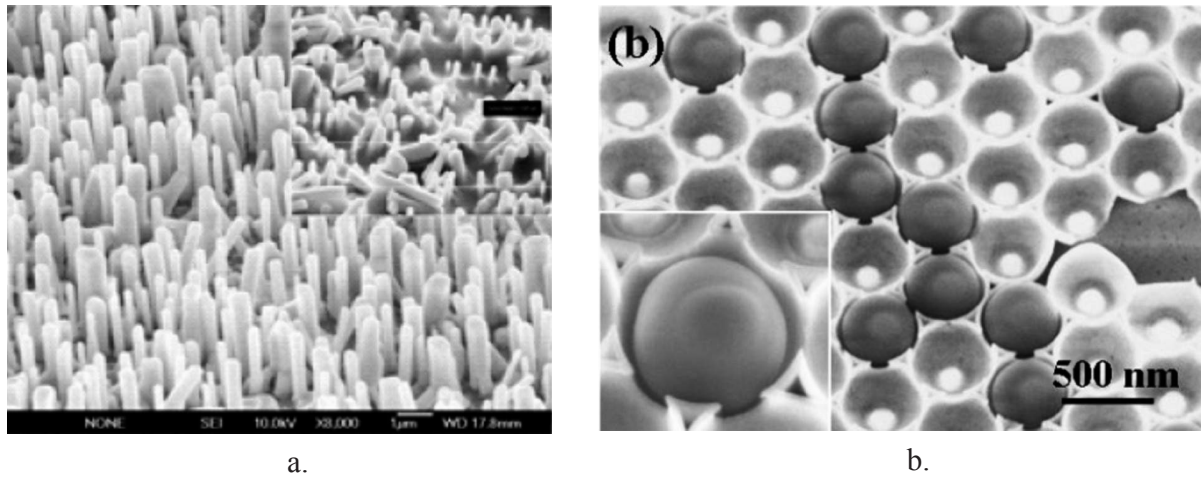
Figure 1.13: Exemples de surfaces architecturées ; a. nano-fils d'oxyde de zinc (Umar et al. 2008); b. tableau de nano-bols ordonné (Xu et al. 2004).
