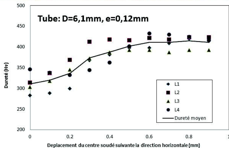
Figure 4.16: Mesure de la liaison soudée- E_{tot}= 160J , E_{puls1}= 15J , E_{puls2}= 145J , F= 100N .
