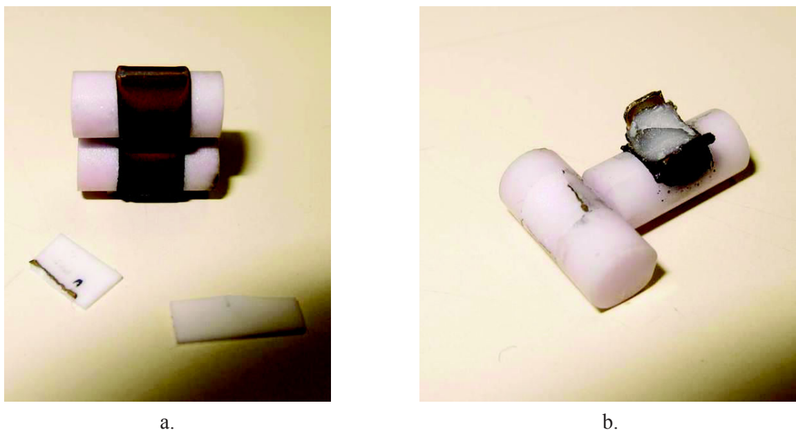
Figure 2.16: Liaison entre TiNi et l'alumine lors du frittage de tubes à 1200°C pendant 2h; a. Deux tubes entiers; b. Deux demi-tubes
