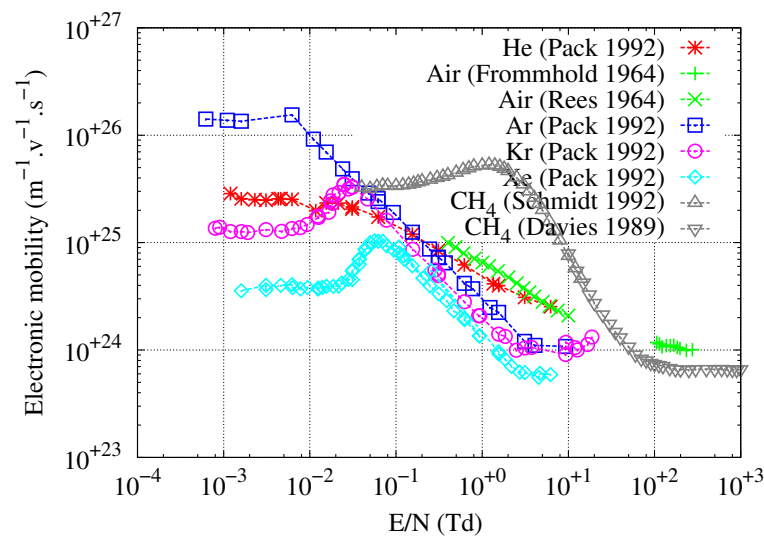
FIGURE 1.9 – Mobilités électroniques pour différents gaz en fonction du champ électrique en Td (pour de l'air à 300 K, 1 \text{ Td} \approx 24,5 \text{ V}\cdot\text{mm}^{-1} ). Ces données sont extraites du site web : http://lxcat.net [18].
