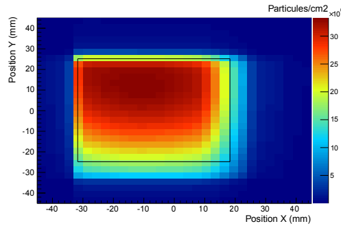
FIGURE 6.19 – Carte de fluence constatée après une panne de quadripoles magnétiques au GANIL en 2014 en faisceau de ^{12}\text{C} à 75 MeV/A.
