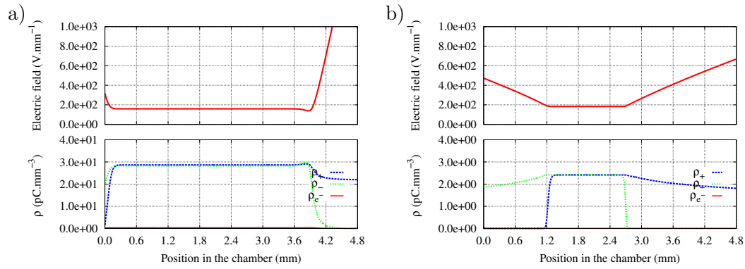
FIGURE 3.10 – Effet de charge d’espace et densités de charges (cations, anions et électrons) dans une chambre à électrodes parallèles de 4,8 mm d’air alimentée à 1600 V pour une ionisation de 100 \text{ pC}\cdot\text{mm}^{-3} délivrée en 10 \mu s . a) À t = 10 \mu s . b) À t = 40 \mu s .
