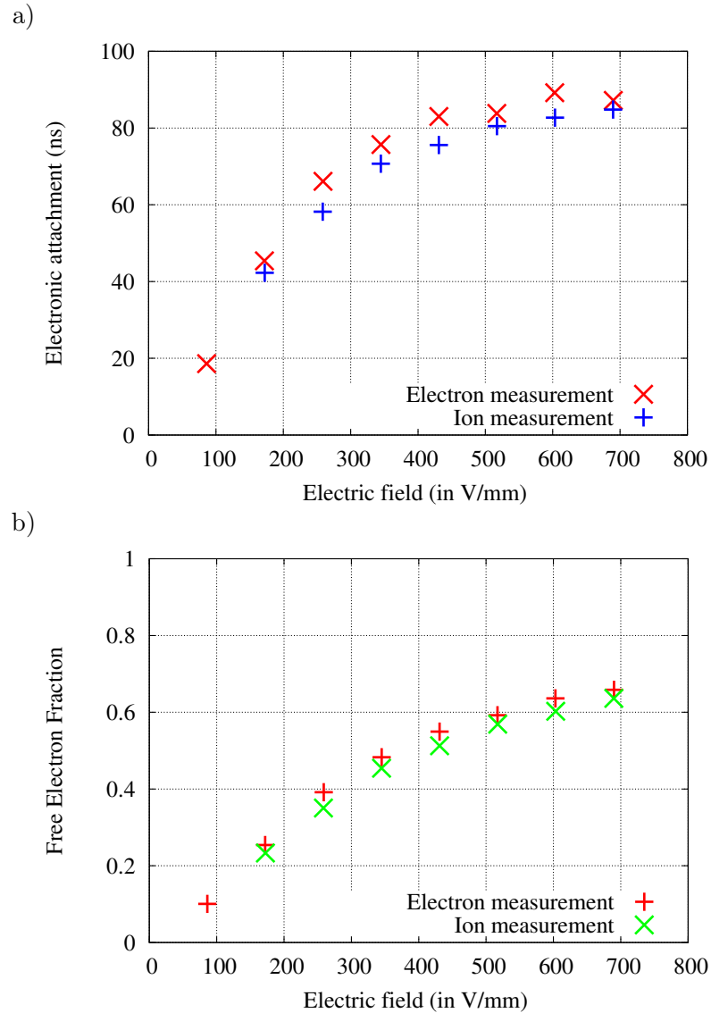
FIGURE 2.15 – Comparaison des résultats de MICMAC pour les deux échantillonnages (2 ns et 0,512 \mu s) dans l'air à 300\text{ K} \pm 2\% et 1,015\text{ hPa} \pm 1\% . a) Constante de temps d'attachement électronique en fonction du champ électrique. b) Fraction d'électrons libres en fonction du champ électrique.
