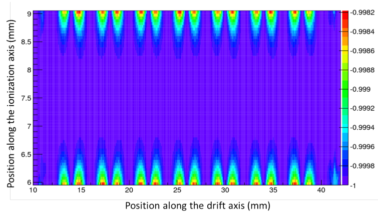
FIGURE 2.17 – Déformation du champ électrique dans la zone de dérive des charges de MAGIC. La déformation (axe Z ) est le rapport entre la composante horizontale du champ E_X et sa norme.
