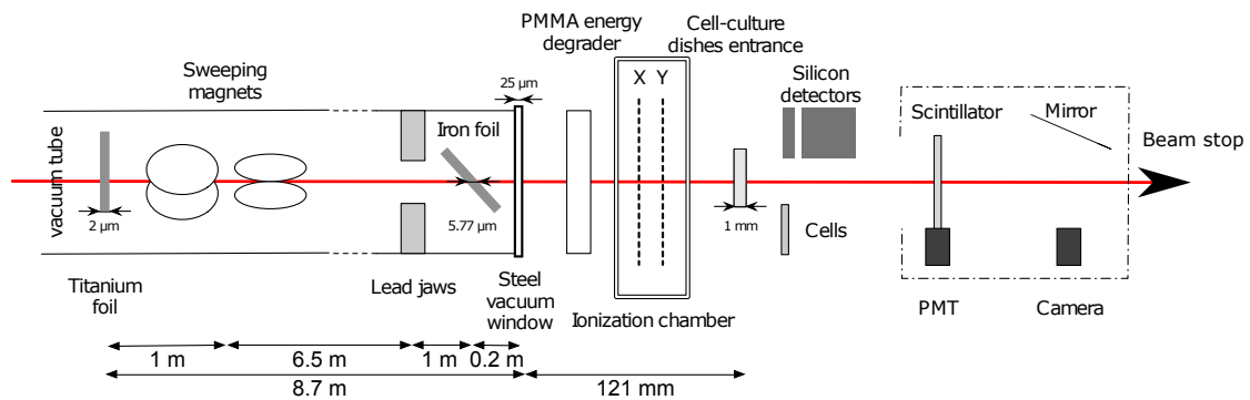
FIGURE 5.3 – La ligne faisceau D1 au GANIL comprend un diffuseur de 2 \mu\text{m} de titane, deux paires d'aimants de balayage, une feuille de 5,77 \mu\text{m} de fer pour la production de rayons X et une feuille de 25 \mu\text{m} d'acier pour la sortie de vide. Avant d'arriver sur les cellules, le faisceau traverse un dégradeur de PMMA, la chambre d'ionisation et le millimètre de polystyrène constituant la fenêtre d'entrée des boîtes de culture. Lors des phases de calibration, les cellules sont remplacées par deux détecteurs silicium à barrière de surface afin de mesurer le TEL des particules et un scintillateur lu par un tube photomultiplicateur qui est placé sur la ligne en aval des boîtes des cultures afin de compter le nombre d'ions. Ce même scintillateur est également observé via un miroir par une caméra afin d'obtenir une visualisation en direct du champ d'irradiation vis-à-vis de la position des boîtes de cultures.
