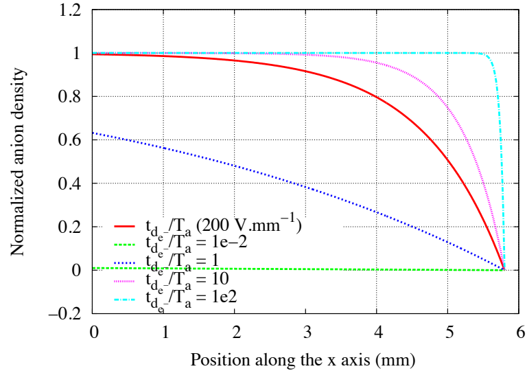
FIGURE 2.3 – Distribution normalisée des anions dans la chambre d’ionisation MICMAC pour différentes valeurs du rapport entre le temps de dérive t_{d_{e^-}} et le temps d’attachement électronique T_a dans le cas où les charges négatives sont collectées en x = 0 et les cations en x = 5,8 mm.
