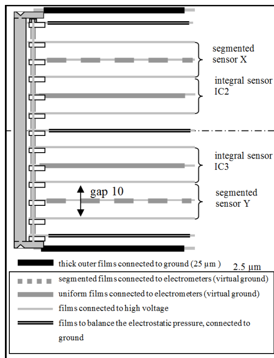
FIGURE 4.7 – Schéma d'IC2/3 comportant les deux électrodes intégrales de mesure d'intensité faisceau et les deux plans de mesure segmentés pour la mesure de la position. Figure extraite de l'article de thèse de Charlotte Courtois [44].
