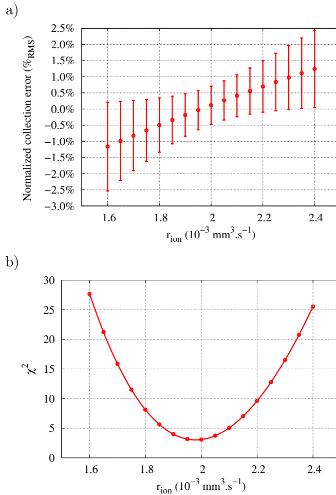
FIGURE 3.2 – Comparaison des données TRAgIC avec les simulations en fonction de r_{ion} sous la forme d'écart moyen (a) (avec les écarts-types correspondants) et de \chi^2 (b) pour l'ensemble des six conditions expérimentales présentées en Tableau 2.1.
