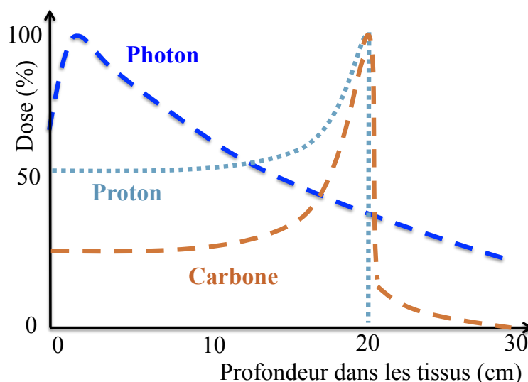
FIGURE 1.2 – Schéma du dépôt de dose de protons et d’ions carbone pour un parcours de 20 cm dans l’eau (en regard de photons mégavolts) en fonction de l’épaisseur d’eau traversée.
