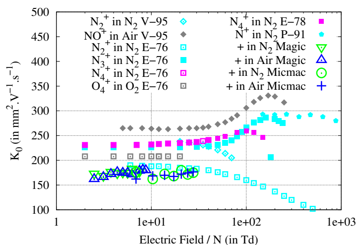
FIGURE 2.23 – Mesures et comparaisons des vitesses de dérive des cations avec la littérature en fonction du champ électrique. Les données de MICMAC et MAGIC sont présentées dans l'air et l'azote en comparaison avec la littérature : GT-70 [40], V-95 [32], E-76 [29], E-78 [30] et P-91 [41].
