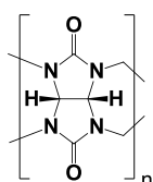
Figure 1. Structure chimique des composés de la famille des cucurbit[n]urils CB[n] .
