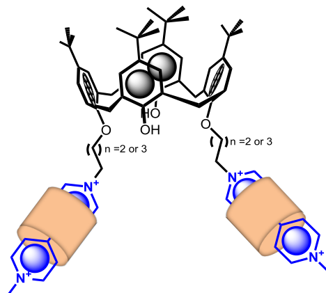
Figure 20. Représentation schématique des [3]pseudorotaxanes C23 4+ · CB[7] 2 et C24 4+ · CB[7] 2 (la cavité hydrophobe du CB[7] interagit avec les groupements bipyridiniums).
