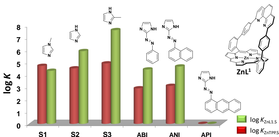
Figure 29. Représentation schématique des valeurs de \log K_{ZnTPP.S} et \log K_{ZnL1.S} qui montre l'importance des liaisons hydrogène avec l'anse phénanthroline sur la stabilisation des complexes pentacoordinés indépendamment du volume d'encombrement de l'azo-chromophore.
