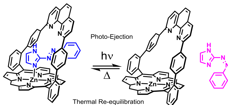
Figure 26. Représentation schématique du principe de photo-éjection d'un azo-aryl-imidazole de son complexe pentacoordiné avec \text{ZnL}^1 .
