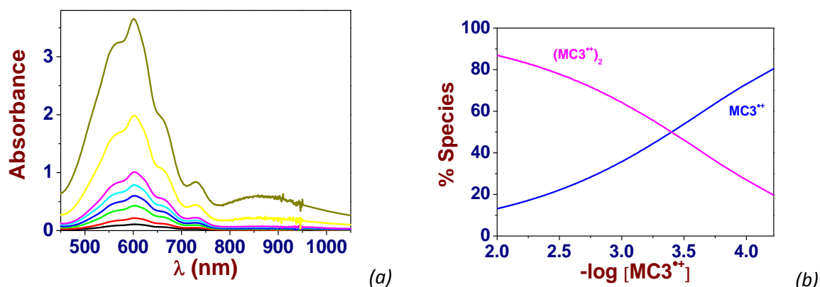
Figure 21. (a) Titrage spectrophotométrique d'absorption UV-Vis.-PIR de MC3^{2+} en solution aqueuse.
