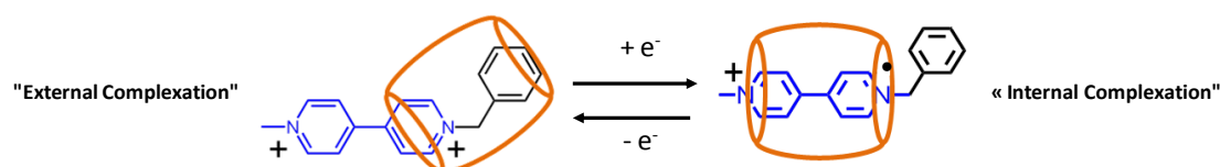
Figure 9. Translocation de \text{CB}[7] contrôlée électrochimiquement pour les complexes avec \text{BMV}^{2+} .
