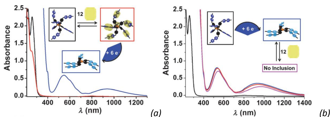
Figure 10. (a) Spectres d'absorption de \text{HV}^{12+} et de \text{HV}^{12+} \subset (\text{CB}[7])_6 . L'addition de \text{Na}_2\text{S}_2\text{O}_4 à \text{HV}^{12+} \subset (\text{CB}[7])_6 induit la dissociation des macrocycles CB[7] comme en témoigne la signature spectroscopique caractéristique (absorption dans le PIR) de l'espèce entièrement dimérisée \text{HV}_D^{6(\bullet+)} . (b) Spectres d'absorption de \text{HV}^{12+} et de son produit de réduction \text{HV}_D^{6(\bullet+)} . L'addition d'excès de CB[7] n'a aucun effet apparent sur le spectre d'absorption de \text{HV}_D^{6(\bullet+)} .
