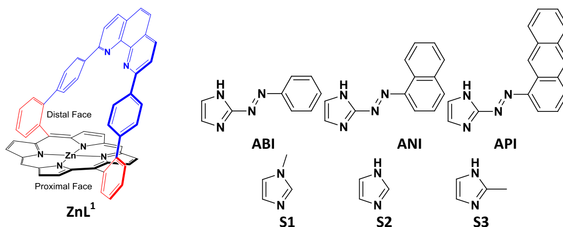
Figure 25. Structures chimiques d'un récepteur à anse phénanthroline ( \text{ZnL}^1 ) et des substrats imidazole ( \text{S1-S3} ) et azo-aryl-imidazole ( \text{ABI} , \text{ANI} et \text{API} ) examinés au cours de ce travail.
