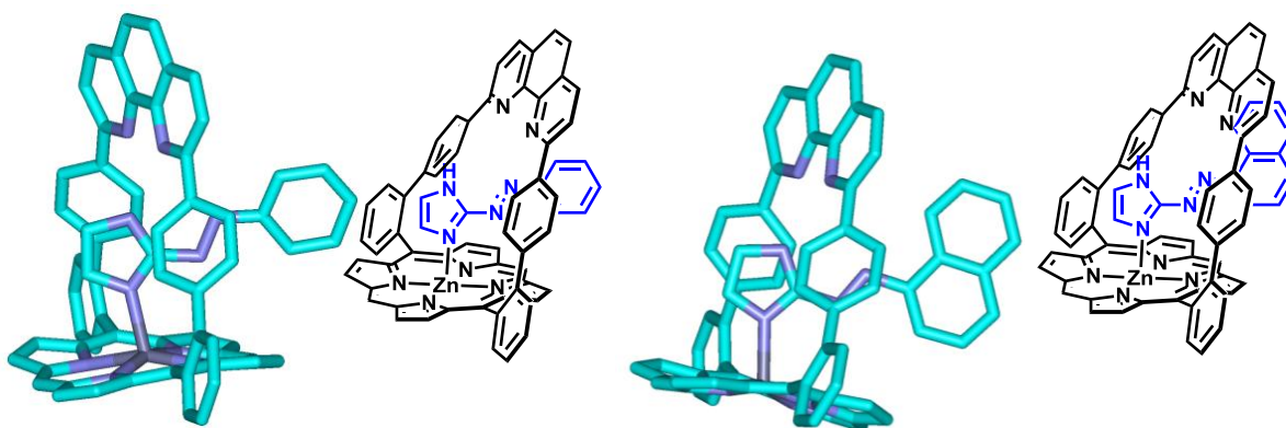
Figure 27. Représentation schématique des structures RX des complexes \text{ZnL}^1\cdot\text{ABI} et \text{ZnL}^1\cdot\text{ANI} .
