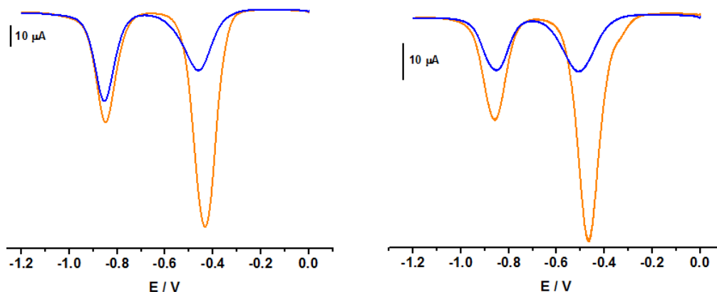
Figure 24. Voltampérogrammes à ondes carrées de C23 4+ , [ C23 4+ ] = 0,05 mM (gauche) et de C24 4+ , [ C24 4+ ] = 0,05 mM (droite) en absence (orange) et en présence de CB[7] (bleu, 3 et 4 équivalents de CB[7] ont été respectivement ajoutés). Tous les voltampérogrammes ont été mesurés sur des solutions aqueuses dégazées et tamponnées à pH 7,0 (0,1 M Na 2 HPO 4 /NaH 2 PO 4 ) à 25°C ( E versus Ag/AgCl).
