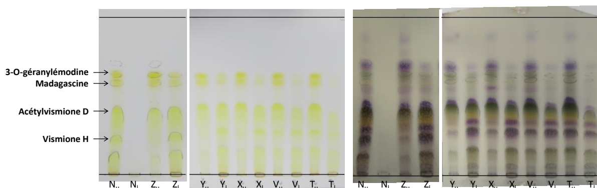
Figure 70 : Evaluation des coefficients de partage par CCM avec la Gamme ARIZONA 257 .
