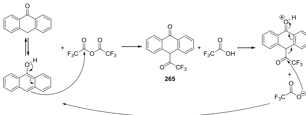
Figure 123 : Mécanisme de formation de l'adduit trifluoroacétique.
