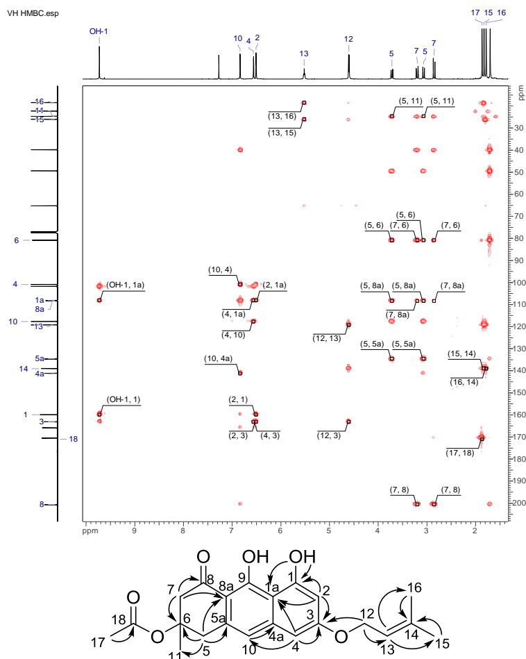
Figure 60 : Principales corrélations HMBC de la molécule A.
