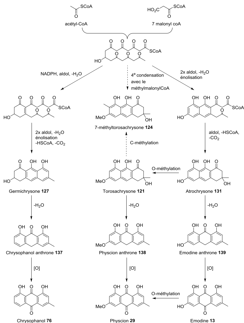
Figure 26 : Voies de biosynthèse des dihydroanthracénones de Senna bicapsularis 151 .
