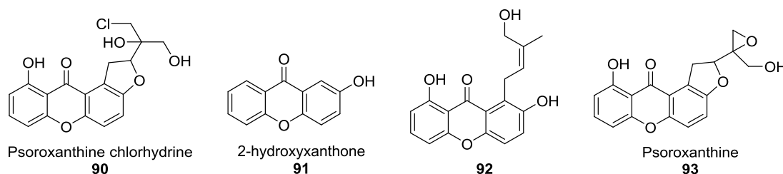
Figure 18 : Molécules isolées de P. molluscum .
