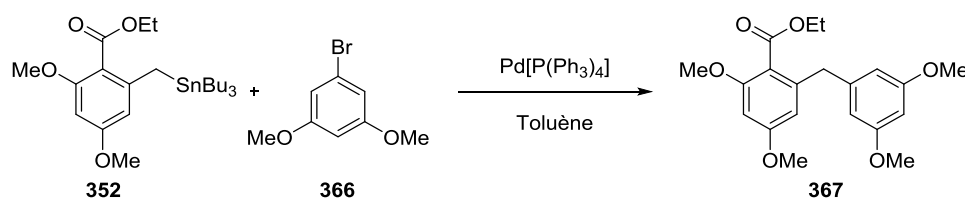
Schéma 56 : Réaction de Stille.
