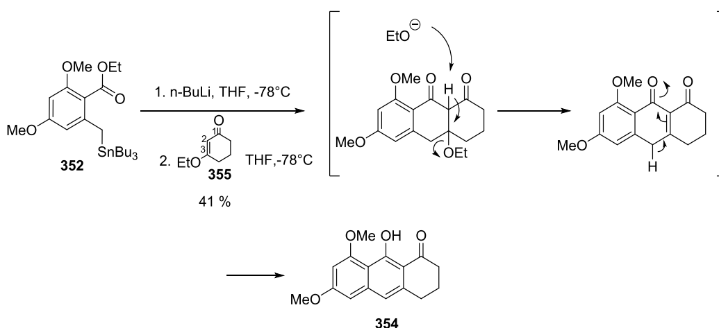
Schéma 50 : Synthèse de la dihydroanthracénone 354 via la \beta -alkoxycyclohexénone 355 .
