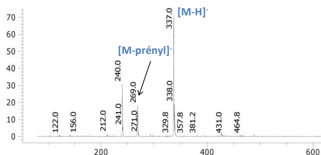
Figure 63 : Spectre de masse basse résolution de la molécule C . APCI mode négatif.
