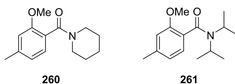
Figure 122 : Dérivés N-pipéridyl- et N,N-diisopropyl-2-méthoxy-4-méthylbenzamide.
