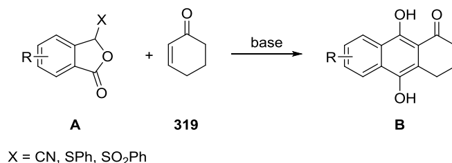
Schéma 36 : Réaction d'annélation de Hauser.
