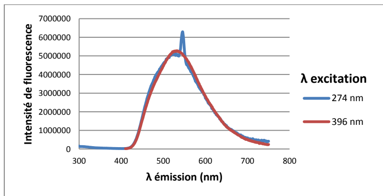
Figure 113 : Spectre de fluorescence de l'acétylvismione D.
