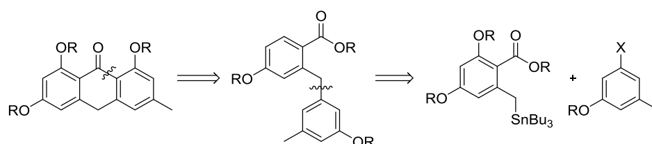
Figure 129 : Rétrosynthèse de l'anthrone par couplage de Stille.
