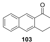
Figure 20 : Structure de base des dihydroanthracénones.
