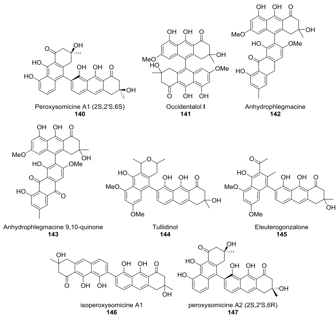
Figure 27 : Aperçu de la diversité des dihydroanthracénones dimériques.
