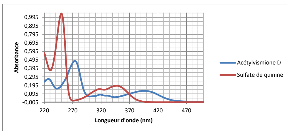
Figure 114 : Spectre d'absorption de l'acétylvismione D et du sulfate de quinine.
