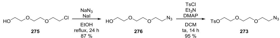
Schéma 24 : Synthèse du dérivé 2-(2-(2-azidoéthoxy)éthoxy)éthyle tosylé 273 .
