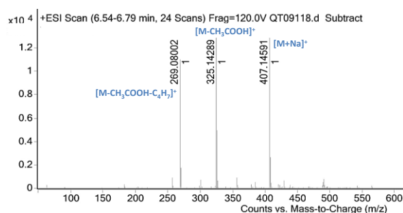
Figure 74 : Spectre HRMS de la molécule E.
