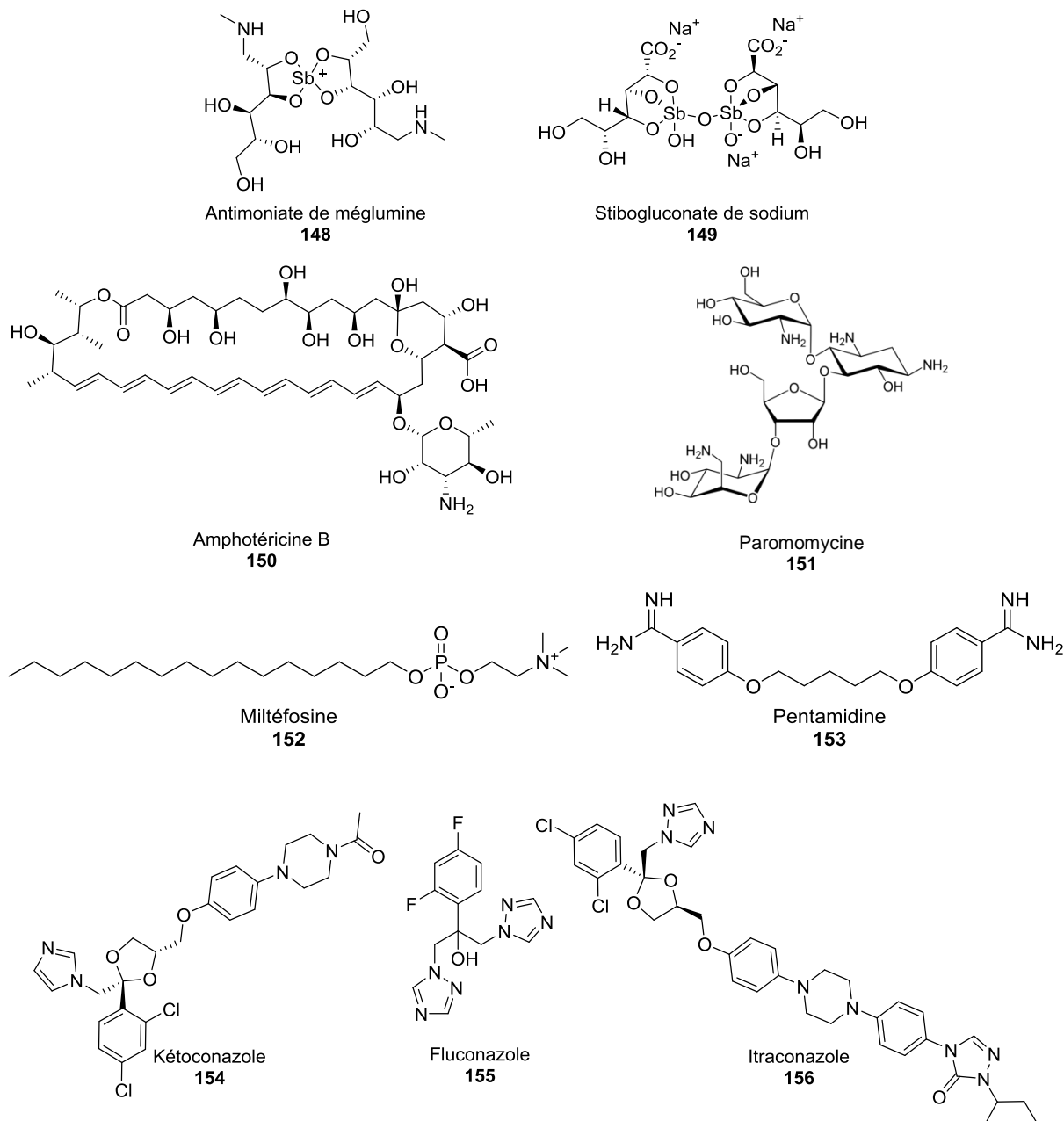
Figure 34 : Molécules utilisées dans le traitement des leishmanioses.
