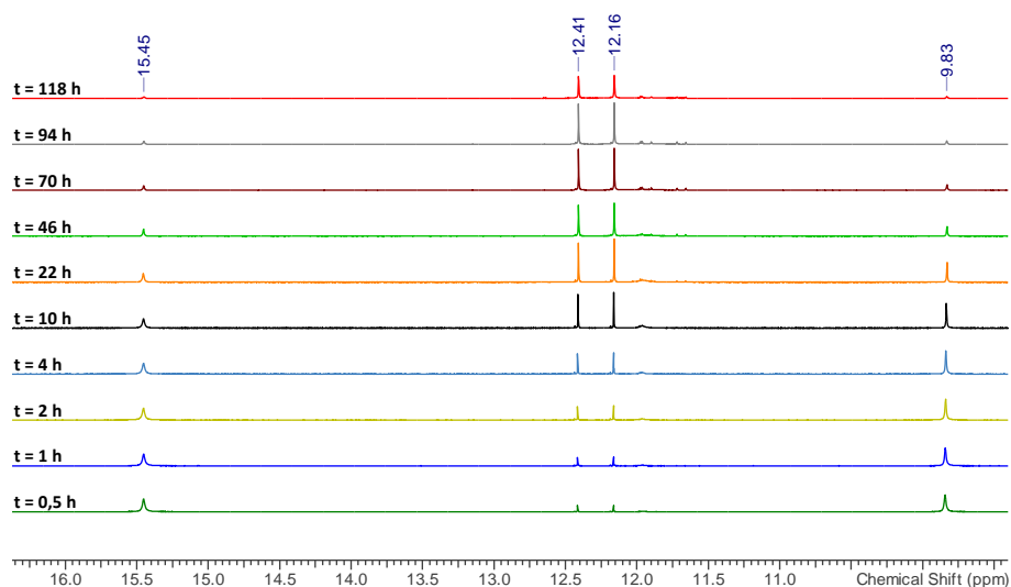
Figure 102 : Suivi RMN ^1\text{H} de la dégradation de l'acétylvismione D dans le DMSO.
