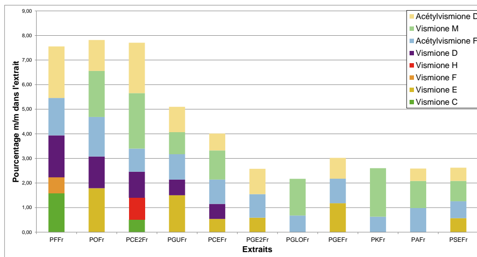
Figure 99 : Teneurs en vismiones des extraits de fruits.
