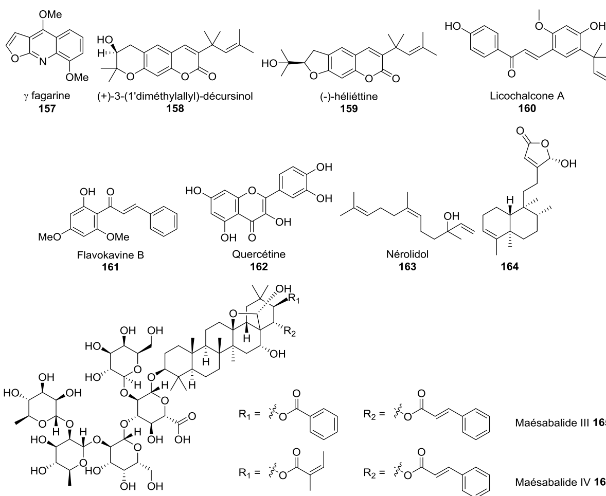
Figure 36 : Exemples de molécules naturelles ayant montré une activité significative sur plusieurs modèles animaux de leishmanioses cutanées et viscérales.
