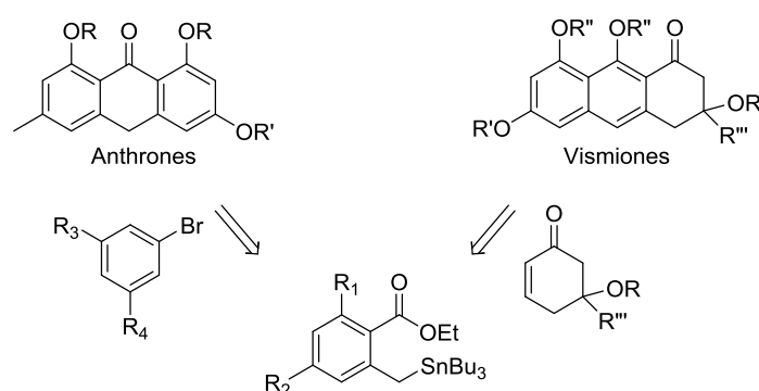
Figure 128 : Synthèse de vismiones et d'anthrones via un dérivé stannylé.
