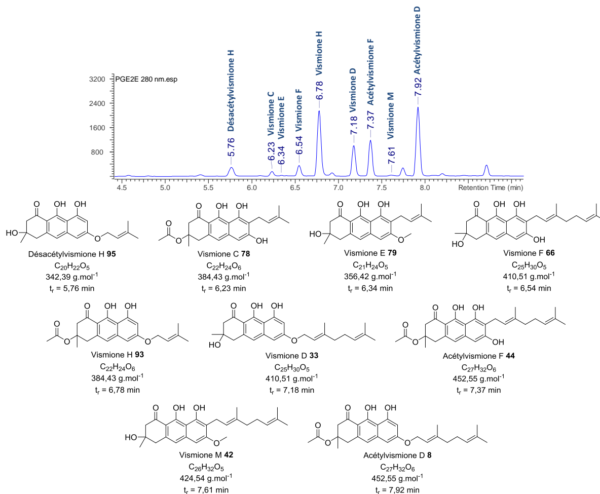
Figure 84 : Bilan du fractionnement de PGPAF en polarité de phase inverse.
