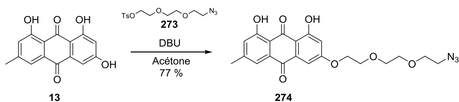
Schéma 23 : Synthèse de l'anthraquinone PEGylée 274 .
