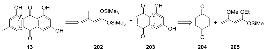
Figure 118 : Rétrosynthèse de l'émodyne par double réaction de Diels-Alder sur une benzoquinone.
