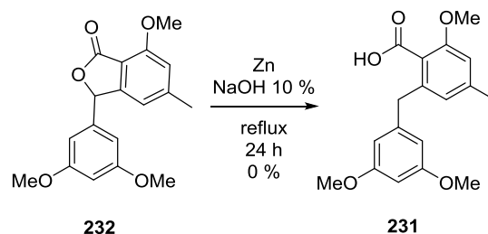
Schéma 13 : Tentative de réduction de la lactone au zinc.
