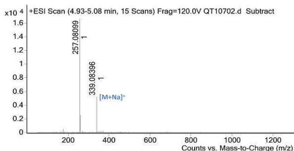
Figure 89 : Spectre HRMS de la molécule L.
