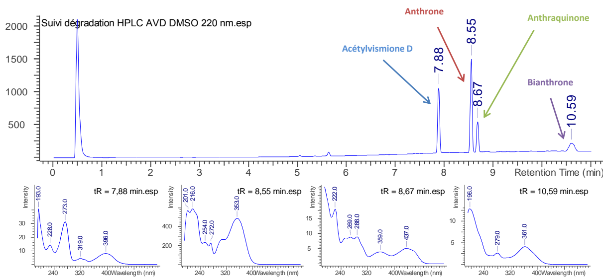
Figure 104 : Chromatogramme du suivi HPLC de la dégradation de l'acétylvismione D sous atmosphère contrôlée.
