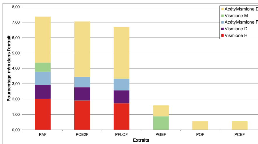
Figure 100 : Teneurs en vismiones des extraits de feuilles.
