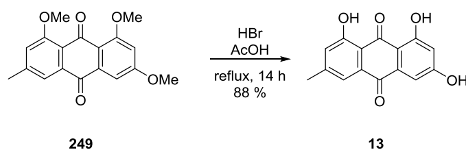
Schéma 19 : Déprotection de la triméthoxyémodine ( 249 ).
