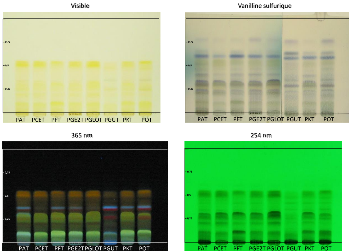
Figure 94 : Profils CCM des extraits DCM de tiges de Psorospermum .
