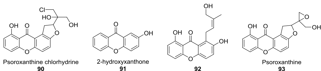
Figure 18 : Molécules isolées de P. molluscum .
