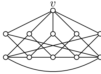
Figure 7.7 – the Mycielski-Grötzsch graph
