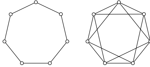
FIGURE 2.2 – un trou impair de longueur 7 et l'anti-trou impair correspondant
