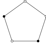
FIGURE 2.1 – le circuit de longueur 5 et un stable de cardinal maximum (en noir). Ce graphe ne peut pas être couvert par 2 cliques
