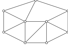
FIGURE 2.3 – un graphe proche-parfait qui n'est ni parfait ni minimalement imparfait
