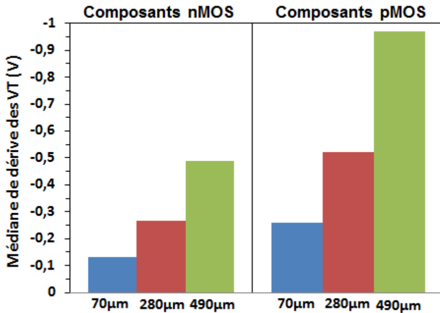
Figure III-22: Médiane de dérive de la tension de seuil des structures de test nMOS et pMOS en fonction de l'espaceur entre les antennes grille et drain après exposition au procédé de gravure métal non-uniforme.
