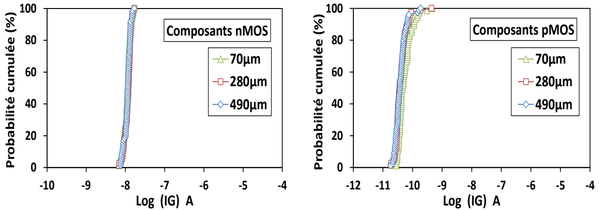
Figure III-21: Evolution de la fuite de grille des composants nMOS et pMOS en fonction de l'espaceur entre les antennes grille et drain.
