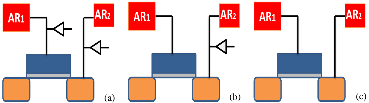
Figure IV-9: Structures de test (a, b et c) avec différentes configurations d'antennes et de protection par diodes.
