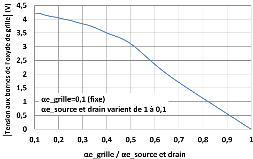
Figure IV-17: Evolution de la contrainte électrique en fonction du rapport entre les facteurs d'ombrage électronique des antennes grille et source/drain, simulée à l'aide du circuit-modèle. \alpha_e\text{ grille}=0,1 et \alpha_e\text{ source et drain} varient de 1 à 0,1. La structure d'antenne considérée est un composant pMOS munie d'un oxyde de grille high-k de 2,3nm d'épaisseur avec des antennes connectées aux nœuds grille et source/drain de rapport d'antenne via AR_{\text{via}}=100 .
