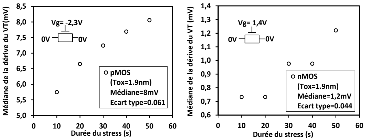
Figure IV-13: Médiane de la dérive de la tension de seuil durant la contrainte électrique de l'ensemble des 70 composants nMOS et pMOS avec un oxyde de grille d'épaisseur de 1.9nm.
