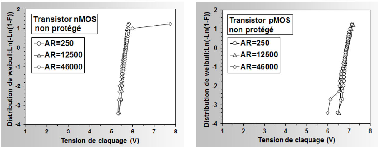
Figure III-9: Probabilité cumulée en échelle de Weibull des tensions de claquage obtenues avec les structure de test nMOS et pMOS non protégées.
