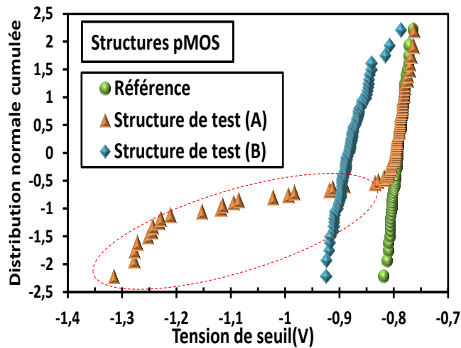
Figure III.18-a: Distributions cumulées des tensions de seuil des structures de test en configuration (A) et (B) après exposition au procédé de gravure métal non-uniforme .
