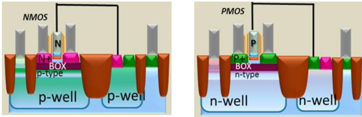
Figure III-4: Modes d'utilisation des diodes de protection : diode n+/pwell pour protéger un transistor nMOS et diode p+/nwell pour protéger un transistor pMOS.
