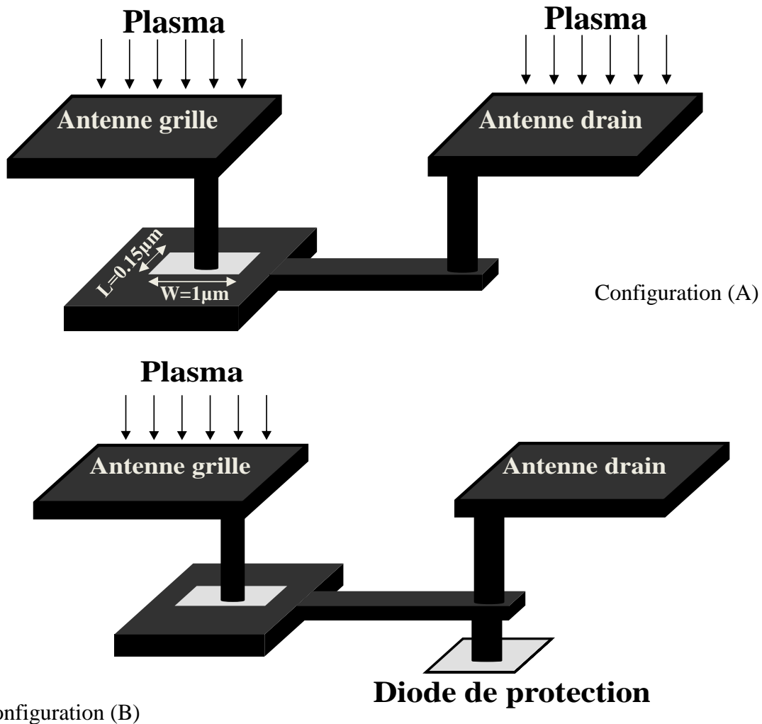
Figure III-17: Configuration (A) : structure définie pour détecter les variations locales du potentiel plasma entre les nœuds du transistor. Configuration (B) : permet de reproduire le comportement des dégradations par non-uniformité du plasma dans un composant standard.
