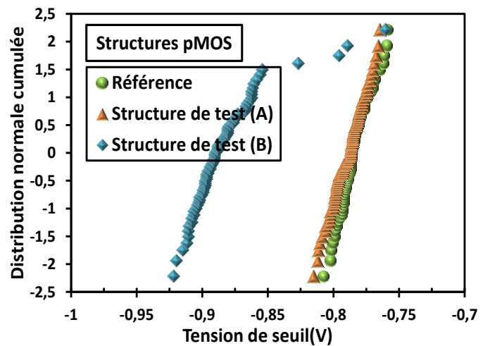
Figure III.18-b: Distributions cumulées des tensions de seuil des structures de test en configuration (A) et (B) après exposition au procédé de gravure métal uniforme .
