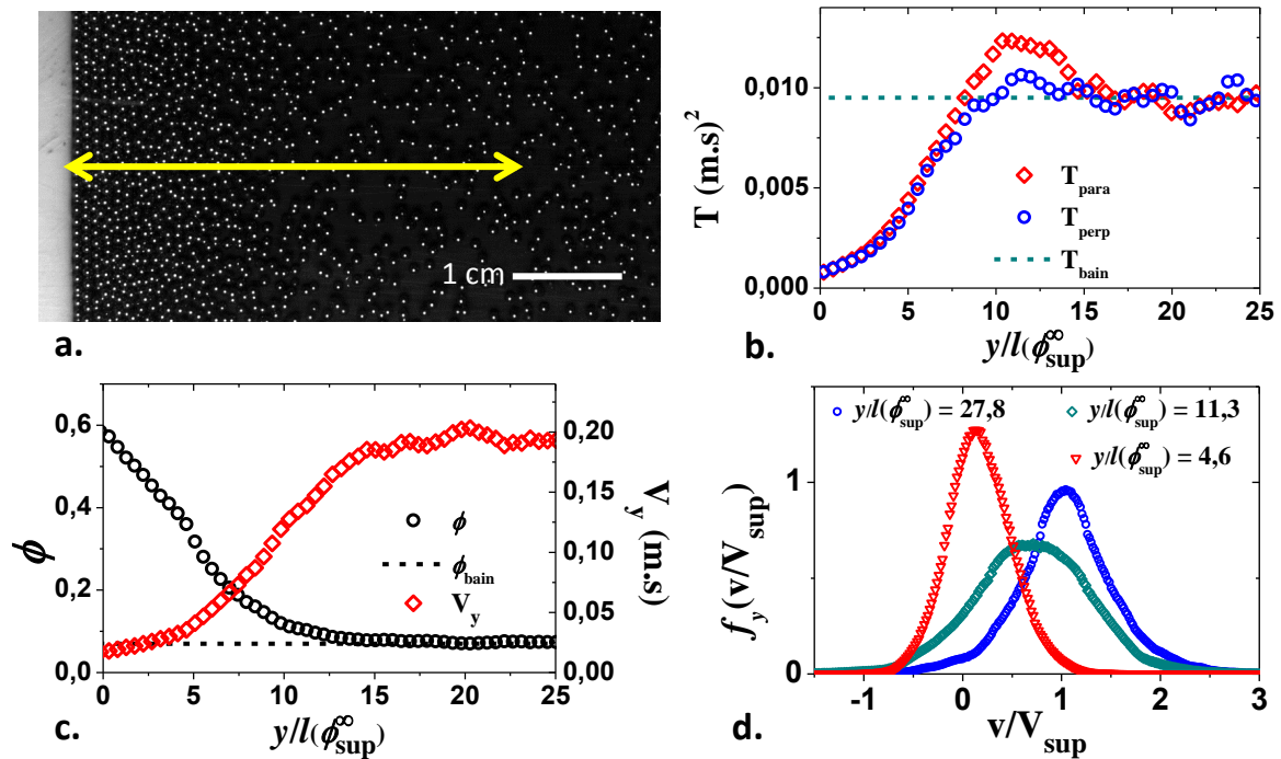
FIGURE 3.15 – a. Photographie du front d’onde généré par un obstacle dans un gaz granulaire ( \phi_{sup}^{\infty} = 0,07 , e = 3 mm, V_{sup} = 0,019 m/s, vibreur : \Gamma = 3,0 g, f = 40,0 Hz, A = 1 mm) filmée en réflexion. b. Températures granulaires longitudinale T_{para} et transverse T_{perp} en fonction de y . La ligne hachurée indique la température initiale du bain vibré. c. Fraction volumique \phi et vitesse moyenne longitudinale V_y mesurées en fonction de y . La ligne hachurée indique la fraction volumique du bain vibré. d. Distributions normalisées f_y(v/V_{sup}) des vitesses longitudinales normalisées V_{sup} pour trois positions différentes dans l’écoulement.
