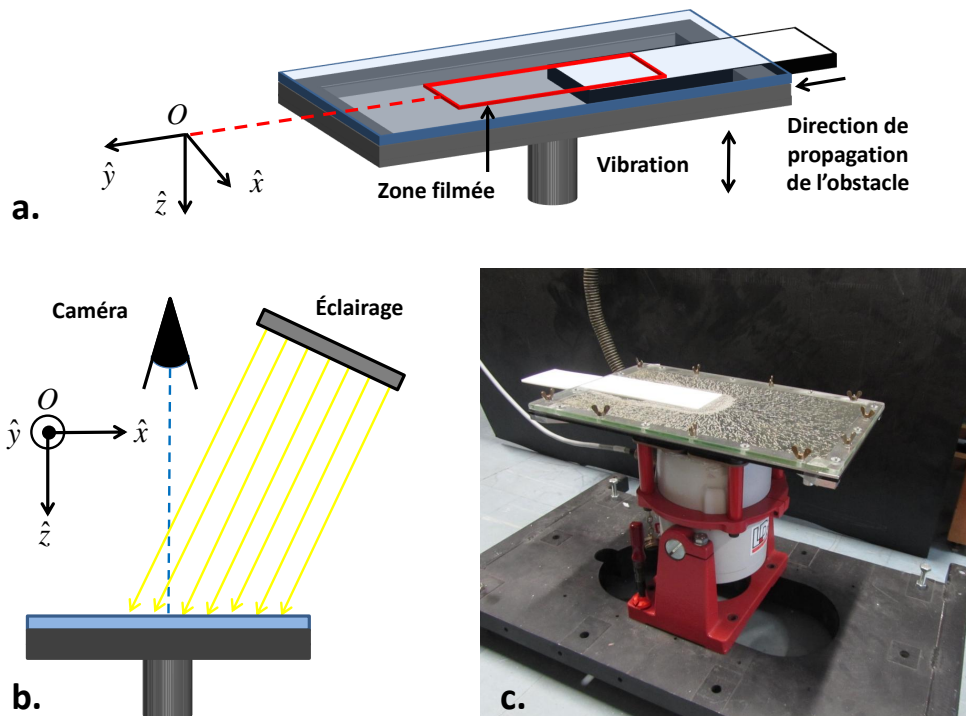
FIGURE 2.9 – Schémas (en perspective a. et de côté b. ) et photographie ( c. ) du montage permettant de générer des ondes de choc dans un gaz granulaire vibré.
