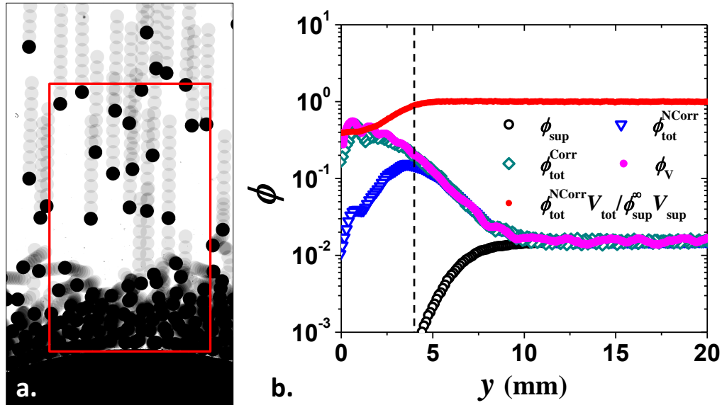
FIGURE 2.15 – a. Chronophotographie d'une onde de choc filmée en réflexion ( \phi_{sup}^{\infty} = 0,017 , V_{sup} = 1,5 m/s, e = 2 mm). Le temps entre 2 positions successives est 0,5 ms. Le cadre rouge représente la zone d'étude où sont mesurées les fractions volumiques. b. Mesure de la fraction volumique \phi_{sup} des particules supersoniques, \phi_{tot}^{NCorr} pour les particules totales détectées par suivi de particules sans correction. \phi_{tot}^{NCorr} V_{tot} / \phi_{sup}^{\infty} V_{sup} = f est le flux de masse mesuré et normalisé. \phi_{tot}^{Corr} est la fraction volumique des particules totales après correction par la procédure décrite. \phi_v est la fraction volumique mesurée en transmission.
