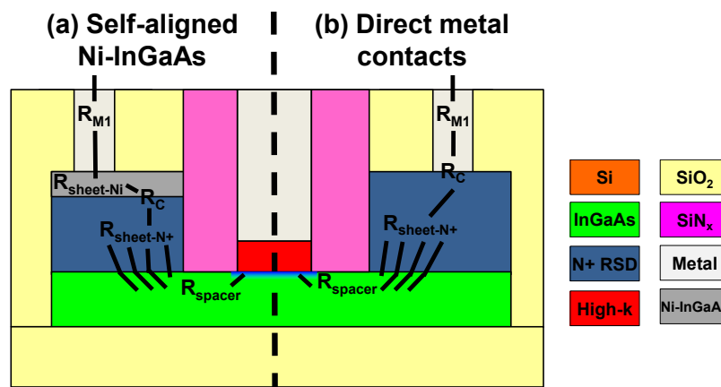
Figure D.4: Schéma d'un gate-first (GF) metal-oxide-semiconductor field-effect transistor (MOSFET) avec raised S/D (RSD) et (a) nickel-indium-galium-arsénide (Ni-InGaAs) ou (b) contacts métalliques directs avec la description des différentes contributions à la résistance série extrinsèque.
