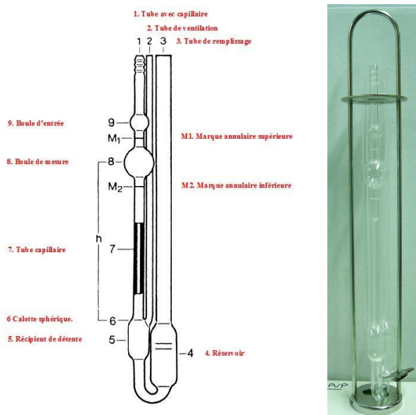
Figure 56: Viscosimètre d'Ubbelhode.
