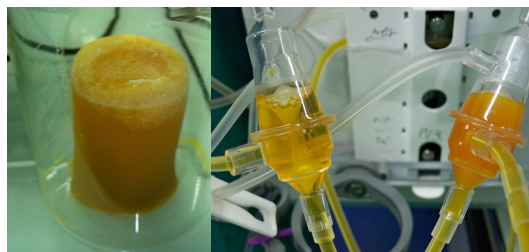
Figure 179: A gauche: Démoulage de la cartouche IE250. A droite : Pièges à bulles en amont et en aval de la cartouche IE250 (le piège à bulle en aval contient du plasma qui totalement figé).
