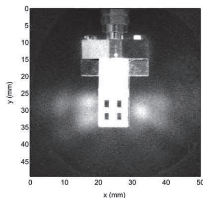
Figure I.14 - Distribution expérimentale à la surface d'un fantôme équivalent de la peau exposé à un réseau d'antennes à 60 GHz [50].
