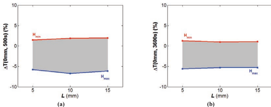
Figure V.9 - Impact de l'incertitude de positionnement du guide d'onde ouvert WR-15 sur l'élévation de température maximale en z = 0 \text{ mm} après (a) 500 sec d'exposition et (b) 1 h d'exposition.
