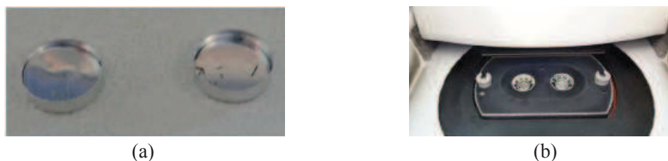
Figure IV.12 - Illustration des capsules dans lesquelles sont placées des échantillons. (a) Exemples de capsules, et (b) capsules positionnées dans la DSC.
