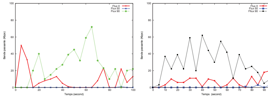
FIG. 4.4 – Débits des flux avec 802.11 (à gauche) et oCSMA (à droite) dans la topologie 50/97
