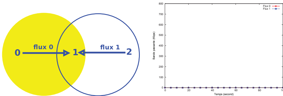
FIG. 1.6 – Collision symétrique
