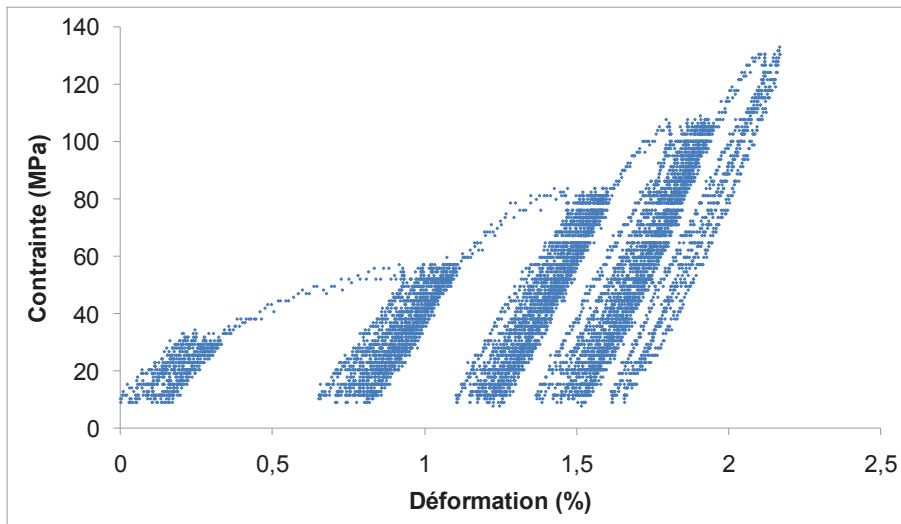
Figure 2-14 : Diagramme Contrainde/Déformation sous l'effet de charges cycliques répétées progressives (T=23°C ; HR=25%)
