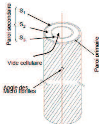
Figure 1-15 : Illustration des différentes parois cellulaires d'une fibre
