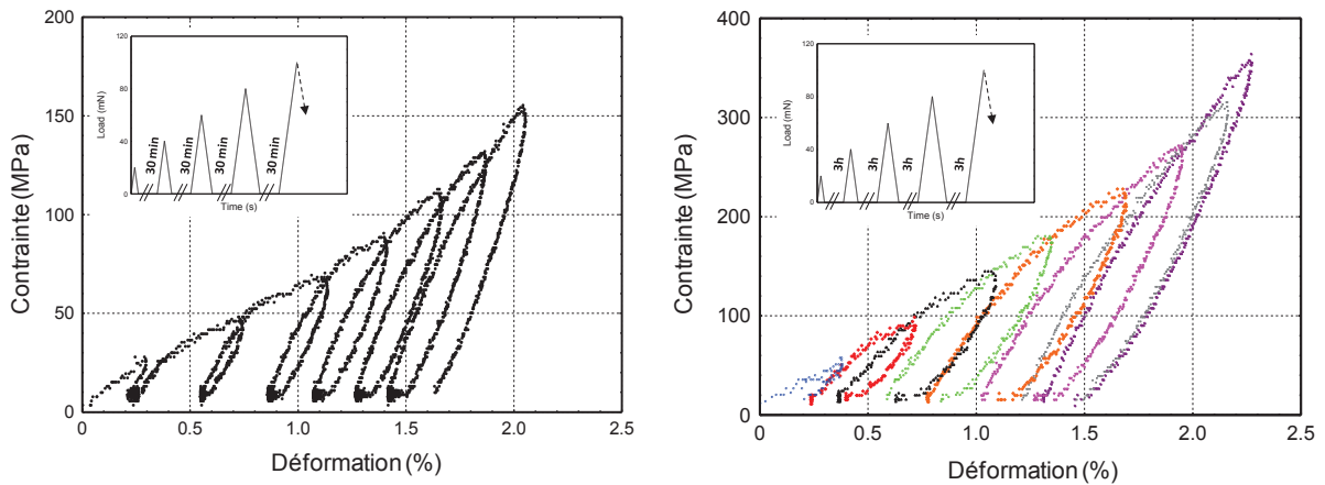
Figure 2-12 : Diagramme Contrainte/Déformation sous charges progressives (T=23°C ; HR=25%)
