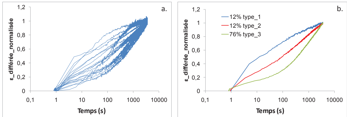
Figure 4-8 : (a) Evolution des déformations différées en fonction du logarithme du temps, (b) Mise en évidence de 3 types de réponses
