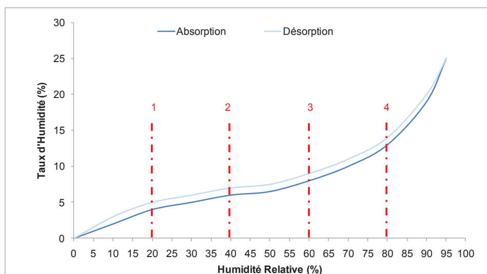
Figure 5-3 : Isotherme de sorption d'eau d'une fibre élémentaire de chanvre d'après (Hill et al., 2009)
