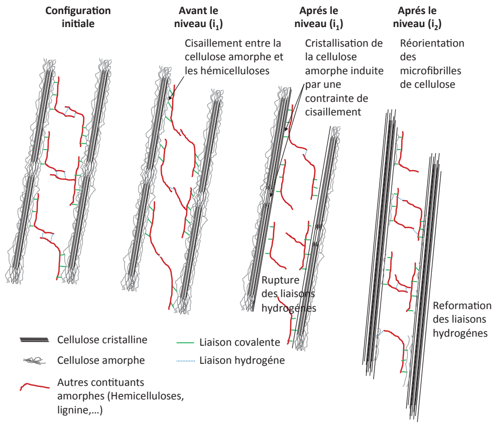
Figure 2-19 : Illustration de l'origine possible du comportement non-linéaire de la fibre en traction quasi-statique
