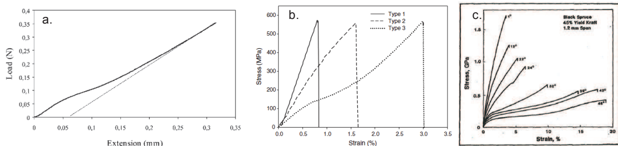
Figure 1-29 : Synthèse des types de comportement observés sur des fibres végétales. Selon les auteurs (Baley, 2002; Duval et al., 2011; Page and El-Hosseiny, 1971)
