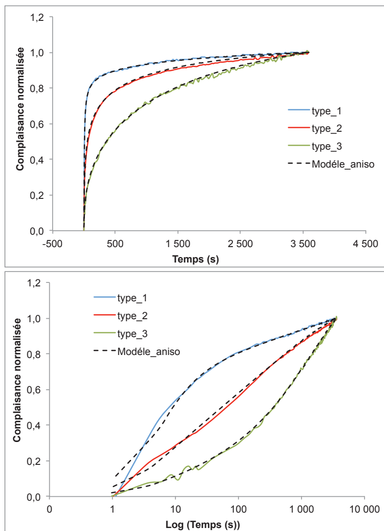
Figure 4-23 : Résultats du modèle anisotrope sur les trois types de comportement
