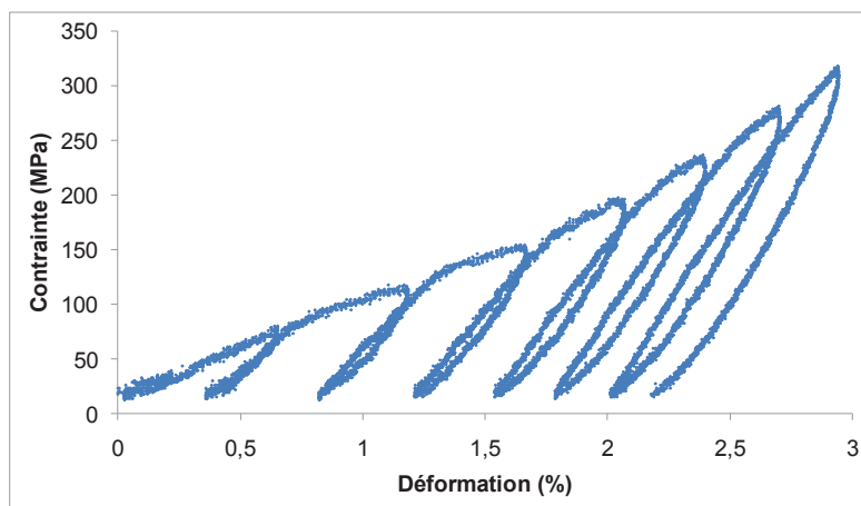
Figure 2-9 : Diagramme Contraincte/Déformation d'une fibre élémentaire sous charges progressives (T=23°C ; HR=25%)
