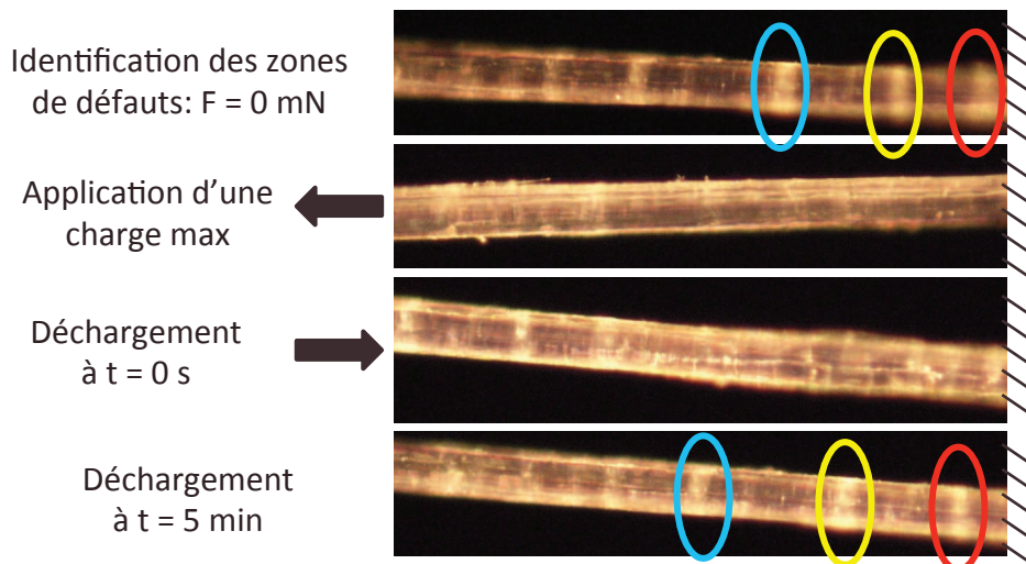
Figure 2-17 : Disparition et réapparition des zones de dislocations
