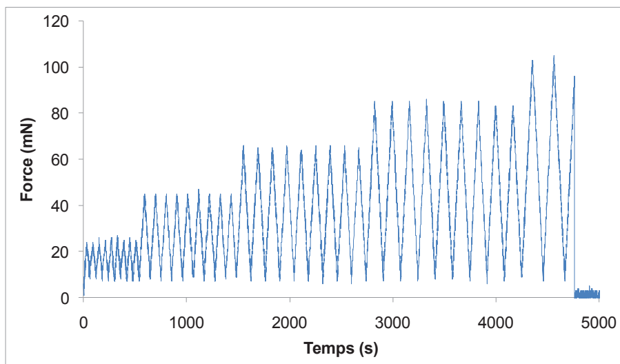
Figure 2-13 : Chargements cycliques répétés progressifs appliqués à une fibre élémentaire (T=23°C ; HR=25%)
