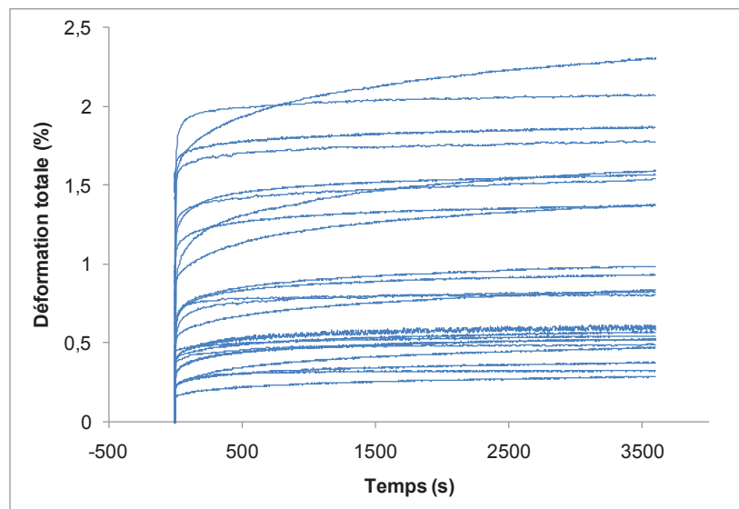
Figure 4-6 : Evolution de la déformation totale au cours du temps pour une campagne de mesures en fluage sur fibres élémentaires de chanvre ( T = 23^{\circ}\text{C} \pm 1.5 , \text{HR} = 50\% \pm 2.5 , \sigma = 50 \text{ MPa} \pm 2 )
