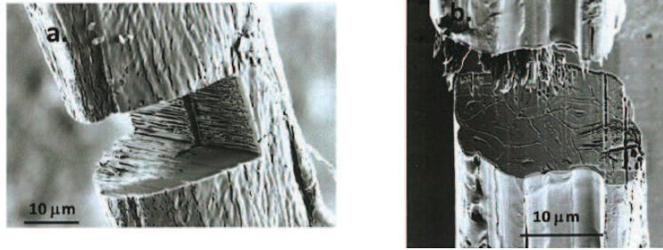
Figure 1-19 : Mise en évidence de la structure interne de deux fibres de chanvre d’une trentaine de microns de diamètre extérieur. a. : fibre élémentaire ; b. : faisceau d’une douzaine de fibres élémentaires. Extrait des travaux de Placet (Placet, 2013)
