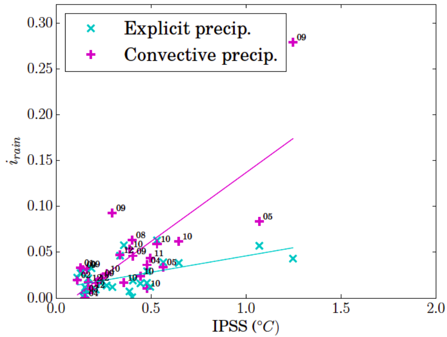
Fig. 6.8 i_{rain} (% du maximum de précipitations totales) en fonction de IPSS ( ^{\circ}C ) calculés comme dans la partie précédente (Eq. (5.4.1) et Eq. (5.4.2)) pour les précipitations explicites (bleu clair) et convectives (rose) dans les zones présentées dans la figure 6.1.
