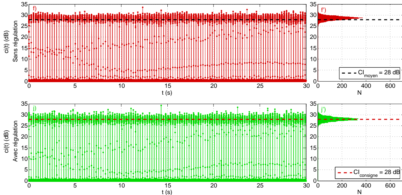
FIGURE 2.12 – Exemple d'évolution temporelle et de distribution du ci(t) durant 30 s à 550 kHz et 7 mgO 2 /L : f ) et f' ) en régime non régulé (courbe rouge et histogramme rouge) pour un ci(t) moyen de 28 dB (lignes en pointillés noires) et j ) et j' ) en régime régulé (courbe verte et histogramme vert) pour un CI_{consigne} de 28 dB (lignes en pointillés rouges).
