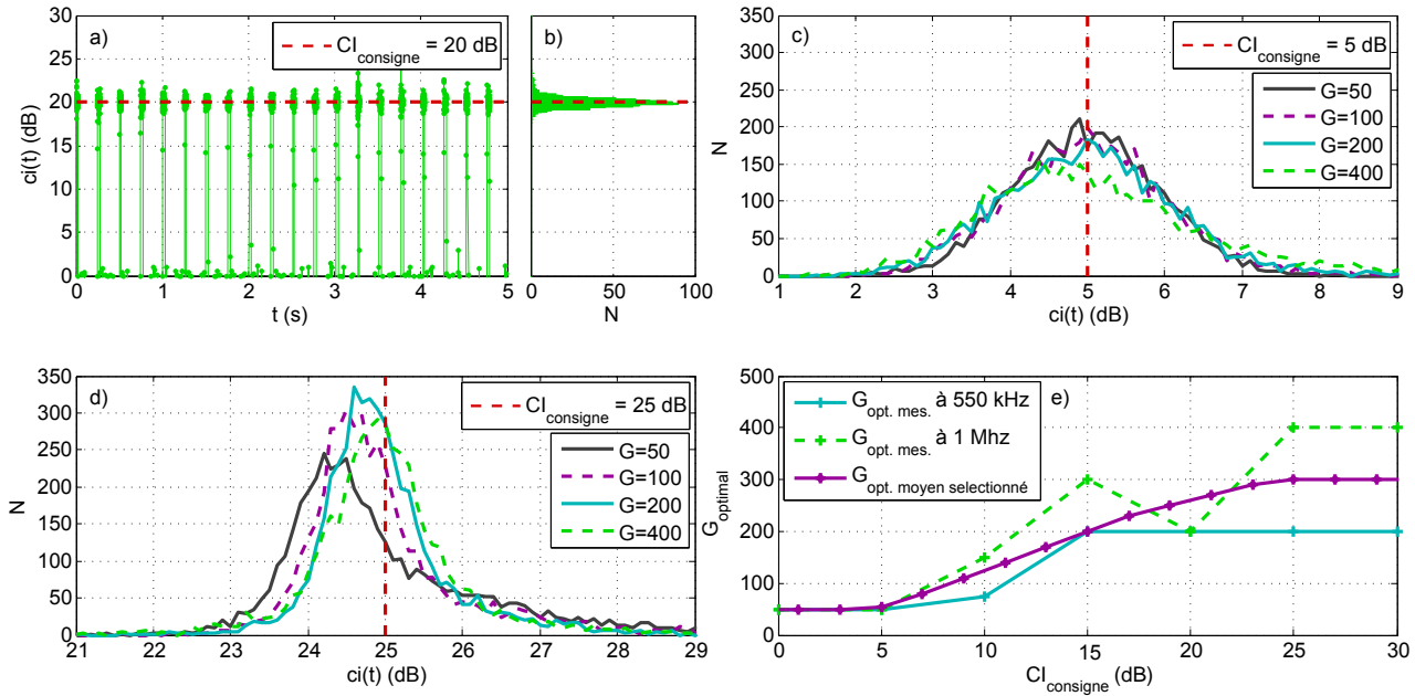
FIGURE 2.8 – a) Évolution temporelle en régime pulsé de l’indice de cavitation ci(t) avec régulation (ligne verte) pour un CI_{consigne} = 20\text{ dB} (ligne rouge), à 550\text{ kHz} et 7\text{ mgO}_2/\text{L} et un gain G = 200\text{ Vpp/dB} . b) Histogramme de la distribution correspondante des ci(t) pendant les temps ON durant 5\text{ s} . Histogramme de la distribution des ci(t) pendant les temps ON durant 20\text{ s} pour différents gains G , à 550\text{ kHz} et 7\text{ mgO}_2/\text{L} , c) pour un CI_{consigne} = 5\text{ dB} (ligne verticale) et d) pour un CI_{consigne} = 25\text{ dB} (ligne verticale). e) Gain optimal mesuré pour différents CI_{consigne} à 550\text{ kHz} (ligne bleue), à 1\text{ MHz} (ligne verte) et gain optimal moyen choisi (ligne violette) à 7\text{ mgO}_2/\text{L} .
