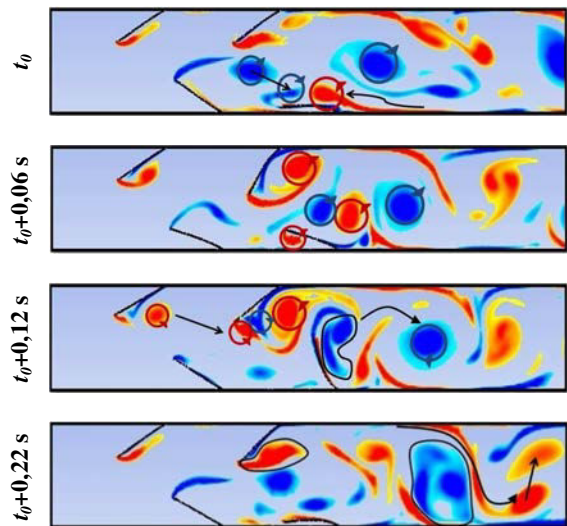
Figure 3: Visualisations instantan es du champ de vorticit  pour la configuration 4FVG
