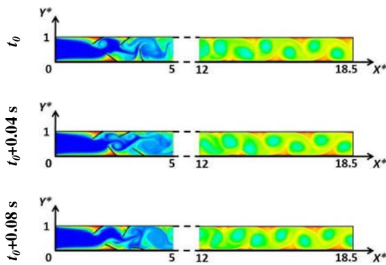
Figure 4: Champ instantan s de temp rature pour la configuration 4FVG. Une partie du champ a  t  volontairement tronqu e de fa on   mettre en  vidence les zones importantes de l' coulement
