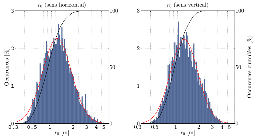
FIGURE 3.65 – Histogrammes des r_0 obtenus dans les deux sens à partir de l'ensemble des mesures différentielles dans la coupole du Mont-Gros. Une fonction log-normale ajustant les données est tracée en rouge tandis que la fonction de répartition est tracée en noir.
