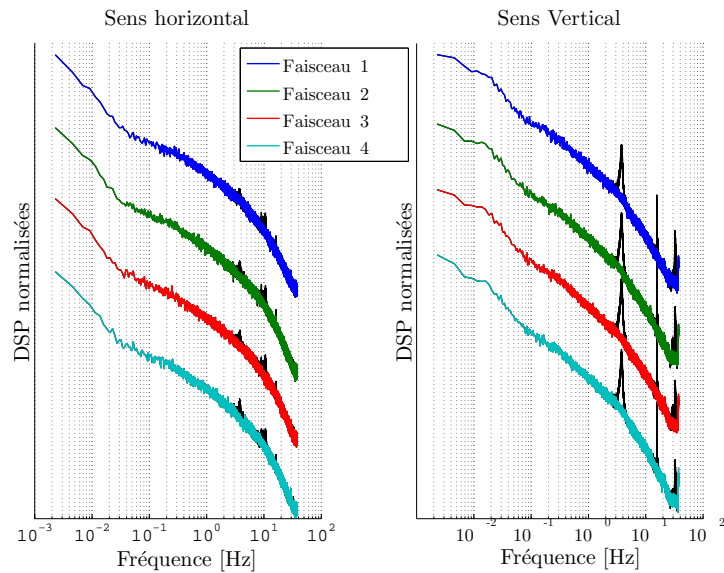
FIGURE 3.7 – DSP des AA pour les différents faisceaux après filtrage. Les DSP sont tracées avec un décalage entre elles pour plus de visibilité. Pour comparaison, les courbes obtenues avant filtrage sont tracées simultanément en noir.
