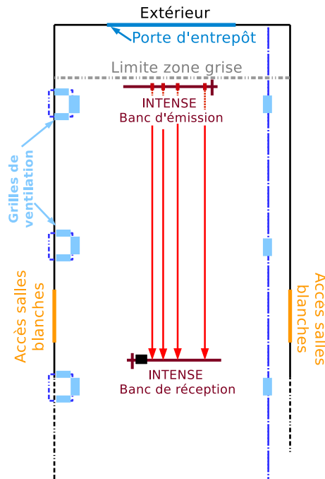
FIGURE 3.2 – Schéma représentatif de l'installation de l'instrument INTENSE dans le SAS matériel pour les mesures en configuration horizontale.
