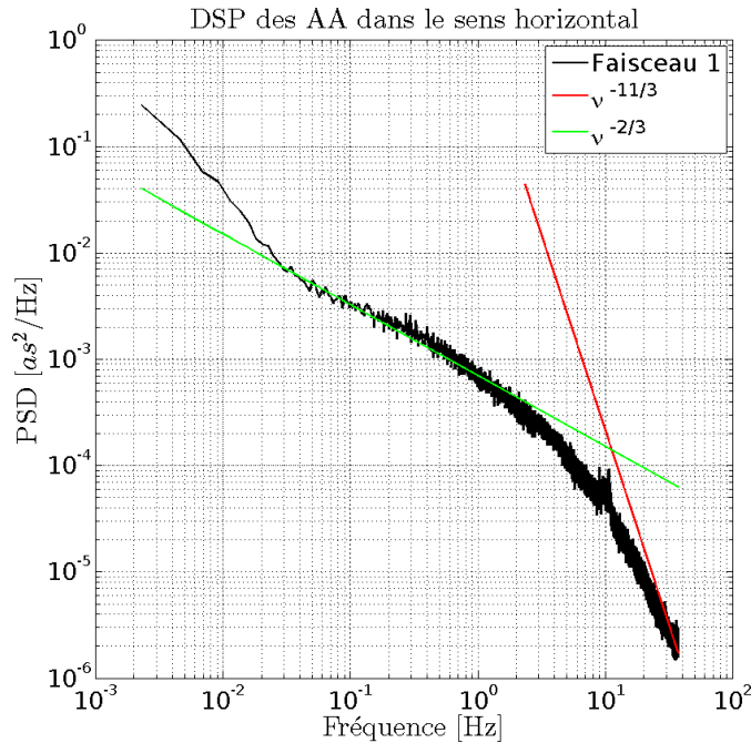
FIGURE 3.13 – DSP des fluctuations des AA dans le sens horizontal. Les tendances en -2/3 et -11/3 sont tracées sur la même figure.
