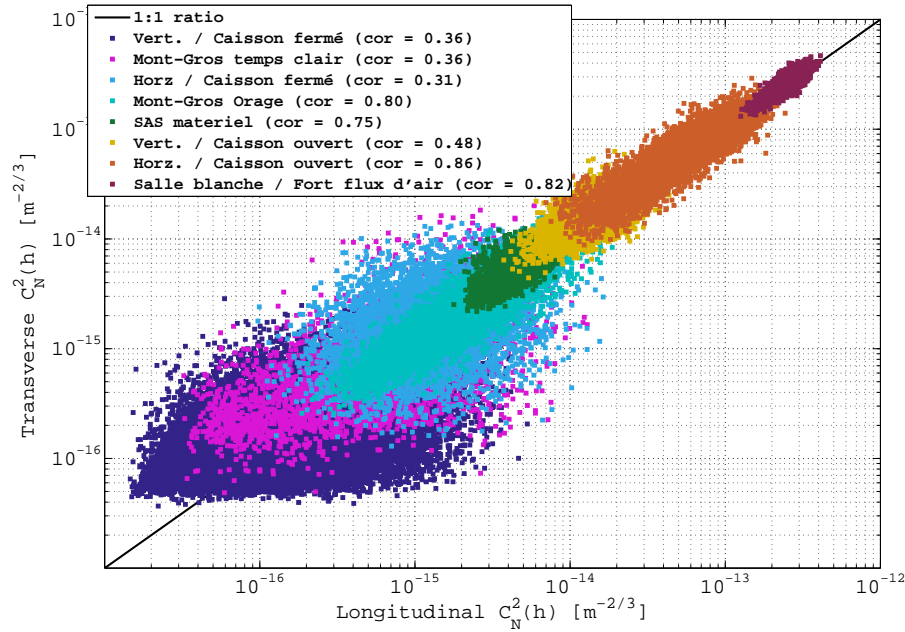
FIGURE 3.69 – Récapitulatif des mesures du C_n^2(h) pour l'ensemble des analyses réalisées durant la période 2013-2014
