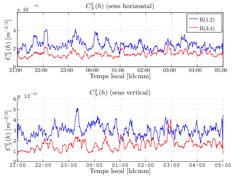
FIGURE 3.38 – Évolution du C_N^2(h) pendant la période de mesure. La base (1;2) est située à l'extrémité Ouest de l'instrument (vers l'intérieur du bâtiment) tandis que la base (3;4) longe le mur Est directement connecté à l'extérieur. Les bases représentées correspondent à des faisceaux voisins entre eux.
