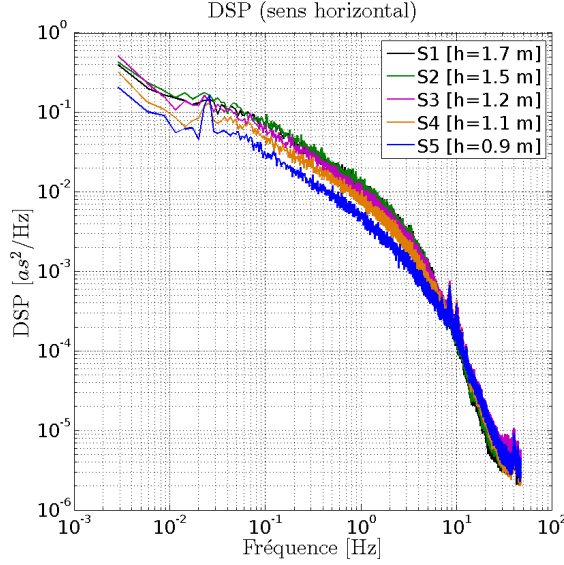
FIGURE 3.55 – DSP des fluctuations des AA issues des mesures de décembre 2014 dans la direction horizontale. Les résultats obtenus pour l'ensemble des faisceaux sont tracés sur cette figure.
