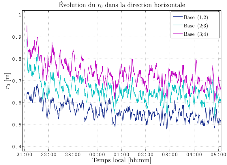
FIGURE 3.10 – Évolution des r_0 pendant la nuit du 08 au 09 Octobre 2013 pour différentes bases. Seuls des r_0 obtenus à partir des variances différentielles des AA dans le sens horizontal sont tracés.
