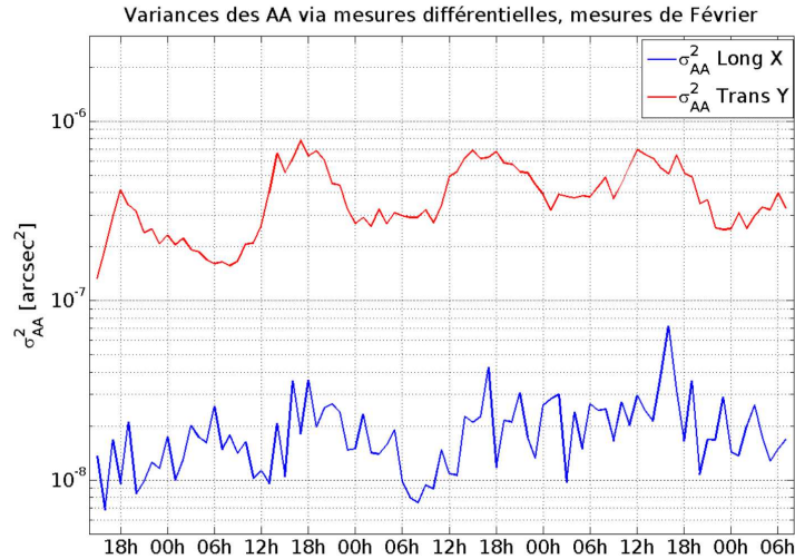
FIGURE 11 – Variance différentielle, base longitudinale en x/y , des fluctuations d'AA ,mois de Février,
