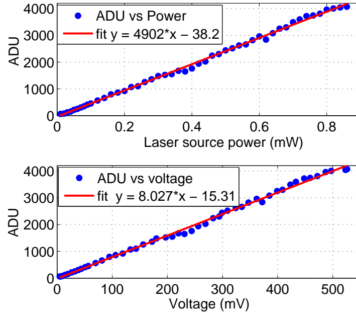
FIGURE 2.12 – Mesure de la linéarité du capteur CCD. En haut, l’amplitude reçue par le capteur CCD comparée avec la puissance affichée sur la source laser. En bas, l’amplitude reçue sur le capteur comparée à celle de la photo-diode.
