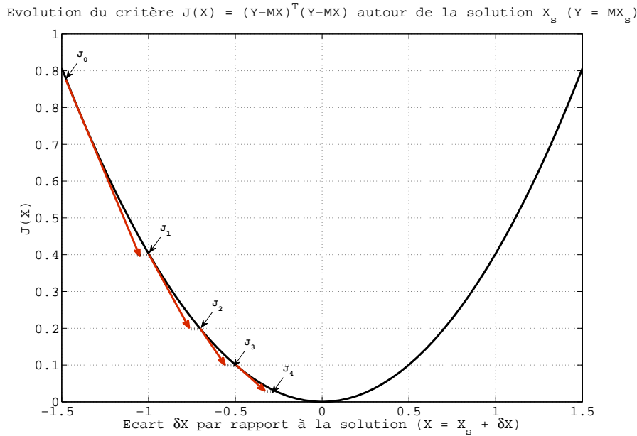
FIGURE 4.20 – Schéma représentatif de la méthode de descente de gradient.
