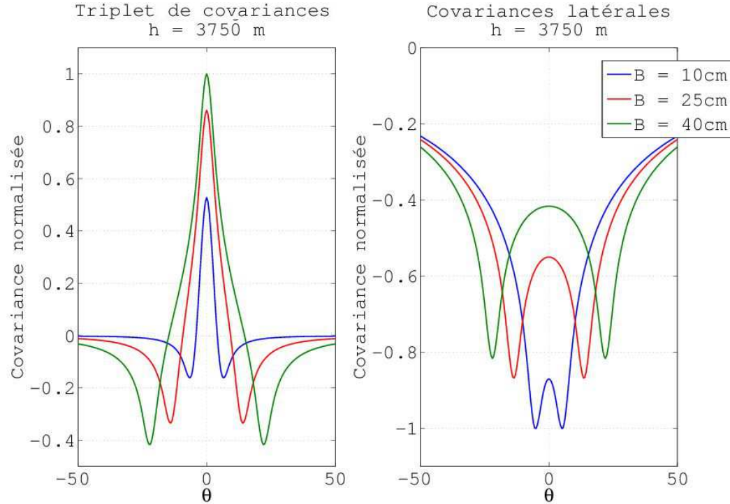
FIGURE 4.4 – Influence de la base B entre les sous-pupilles sur les covariances théoriques. A gauche le triplet de covariances pour une altitude h=3750\text{m} , à droite les covariances latérales pour la même altitude.
