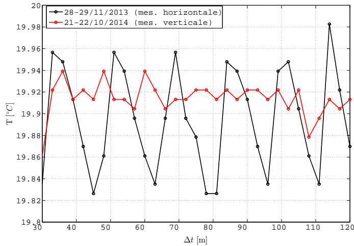
FIGURE 3.50 – Relevés de température dans la salle située au Sud du caisson pour les périodes de mesures de novembre 2013 et d’octobre 2014. Les mesures sont tracées à partir d’une acquisition de référence.
