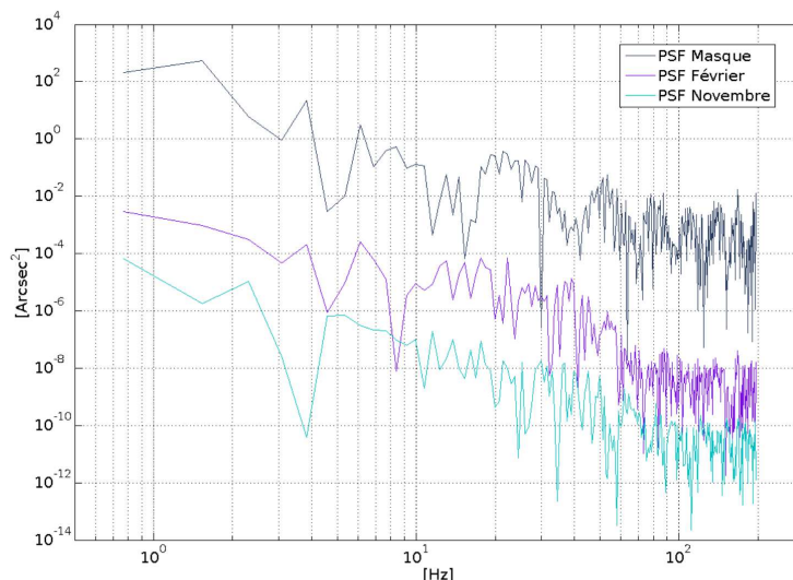
FIGURE 4 – Spectre du masque et des mesures obtenues pour les deux séries
