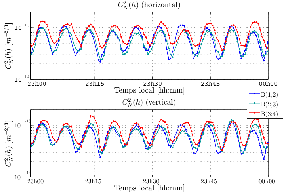
FIGURE 3.31 – Évolution du C_N^2(h) pour la période de mesure dans le caisson en situation portes ouvertes. Les bases présentées correspondent à des faisceaux voisins.
