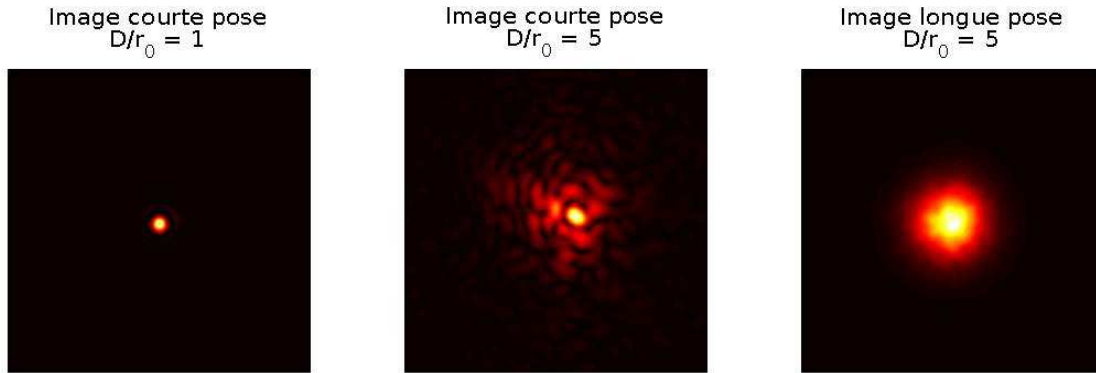
FIGURE 1.4 – Simulation d’images courtes-poses et longues-poses dégradées par la turbulence atmosphérique via le modèle de Kolmogorov. La dégradation de l’image augmente en fonction du rapport D/r_0 où r_0 est le paramètre de Fried défini par l’équation 1.27
