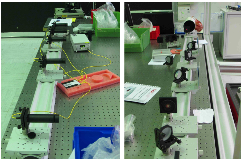
FIGURE 2.1 – Photographies des profilés supportant les éléments optiques d’émission (à gauche) et de réception (à droite) de l’instrument INTENSE.
