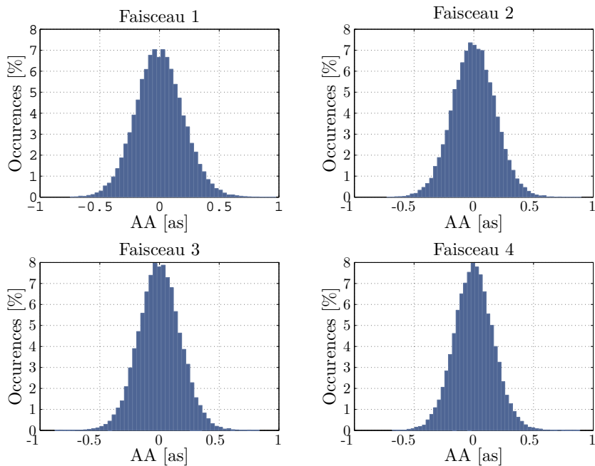
FIGURE 3.5 – Histogrammes individuels des AA dans le sens horizontal pour les quatre faisceaux.
