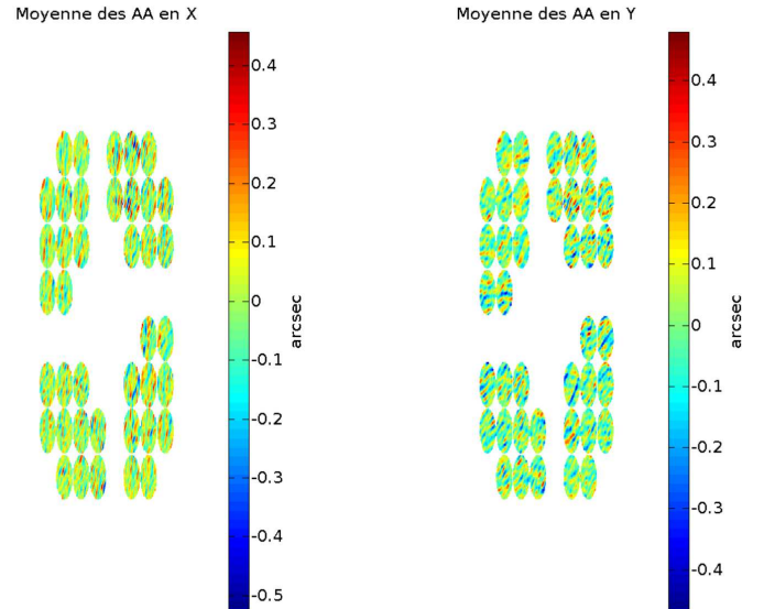
FIGURE 6 – Angles d’arrivée en x/y pour les mesures de Février en arc-secondes
