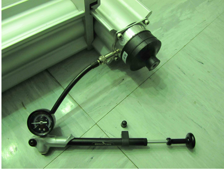
FIGURE 2.9 – Isolateur SLM fixé aux pieds de l'instrument INTENSE dans le but de limiter l'impact des vibrations sur les mesures.
