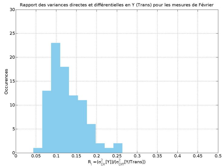
FIGURE 16 – Histogramme du rapport R en y avec une base transversale pour les mesures de Février L_0(t) médian égale à 0.0742 mètre
