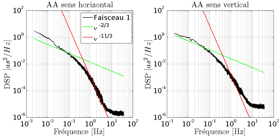
FIGURE 3.41 – DSP des fluctuations des AA dans les deux directions. Les tendances en -2/3 et -11/3 sont tracées sur la même figure.
