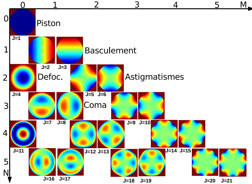
FIGURE 1.8 – Représentation des premiers modes des polynômes de Zernike permettant de décomposer spatialement les déformations de la phase de l’onde incidente.
