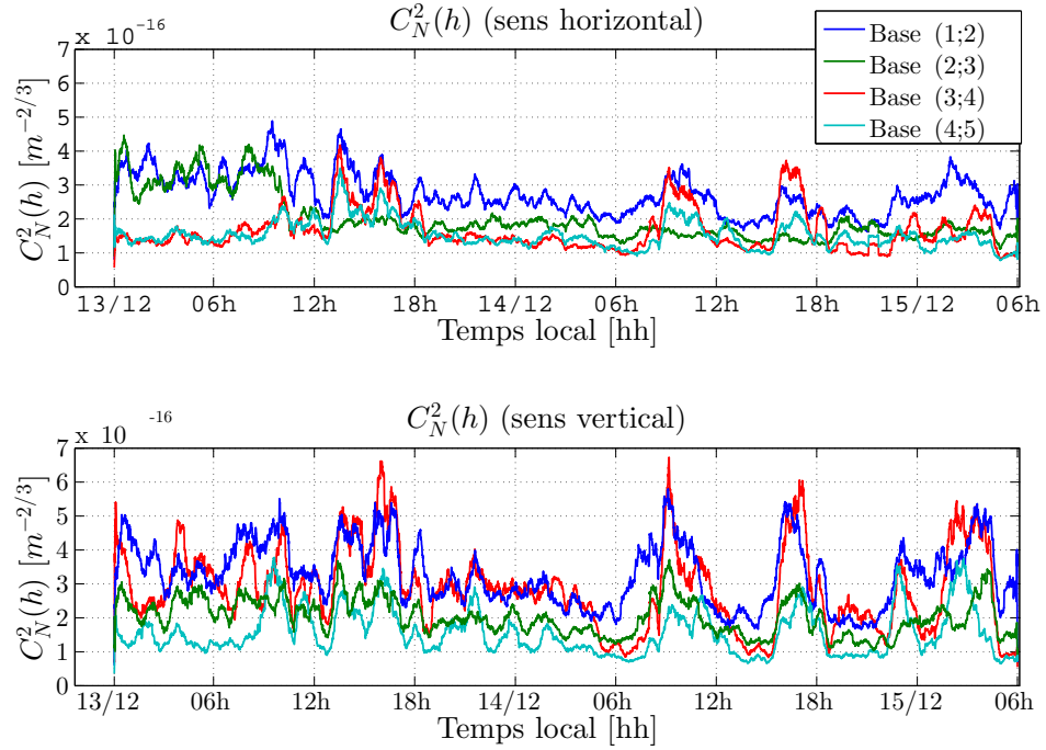
FIGURE 3.57 – Évolution des mesures du C_n^2(h) obtenu à partir des variances différentielles des AA pour différentes bases. Le C_n^2(h) est calculé dans les deux directions.
