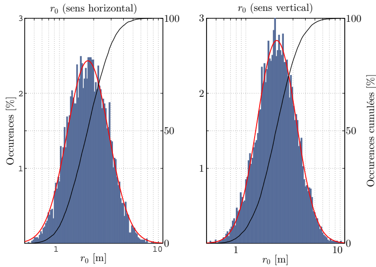
FIGURE 3.37 – Histogrammes des r_0 obtenus dans les deux sens à partir de l'ensemble des mesures différentielles. L'ajustement des histogrammes par une fonction gaussienne est tracé en rouge tandis que la fonction de répartition est tracée en noir.
