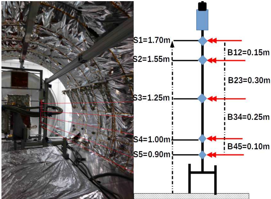
FIGURE 3.44 – Photographies et schéma de l'instrument INTENSE en configuration verticale à l'intérieur du caisson.
