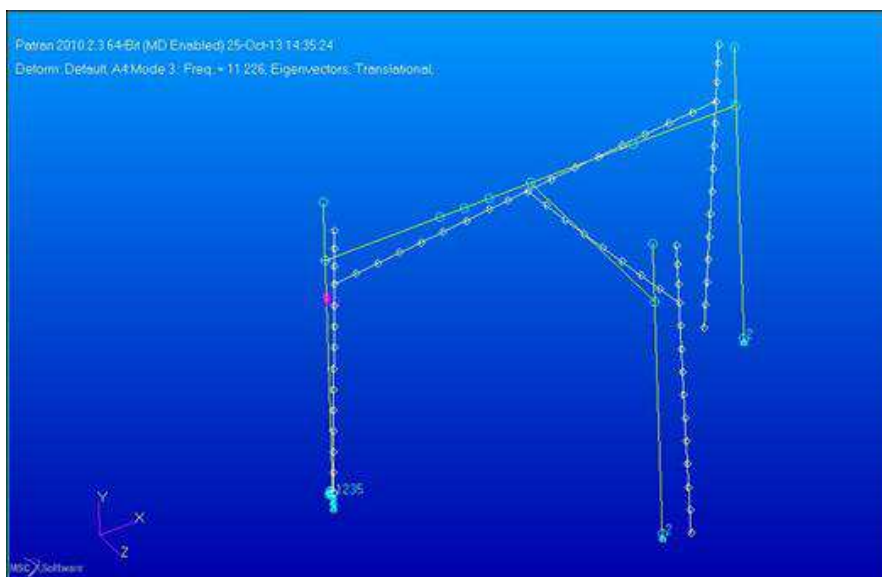
FIGURE 2.5 – Simulation des contraintes et déformations de la structure des bancs initialement employée par l'instrument INTENSE.
