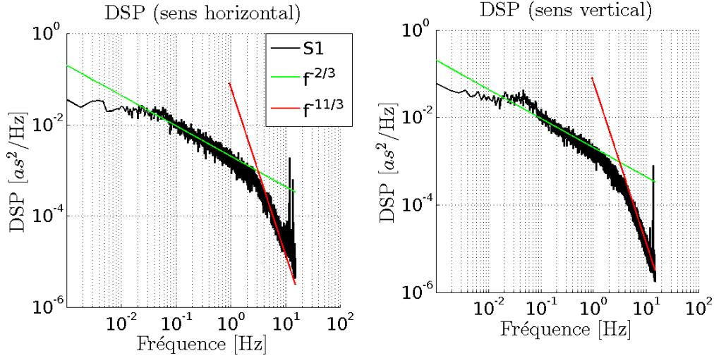
FIGURE 3.53 – DSP des fluctuations des AA issues des mesures d’octobre 2014 dans les deux directions. Les tendances en -2/3 et -11/3 sont tracées sur la même figure.
