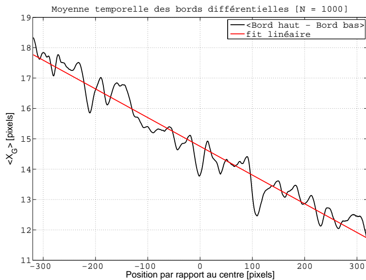
FIGURE 4.17 – Impact du positionnement du prisme de Dove sur les mesures barycentriques. La moyenne du bord différentiel obtenue pour une série de 1000 images est tracée. Le mauvais positionnement du prisme peut induire une différence d'angle entre les bords obtenus pour chacune des sous-pupilles.
