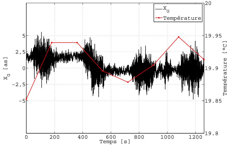
FIGURE 3.29 – Évolution des fluctuations des AA dans la direction longitudinale (horizontale) et de la température dans le caisson. Les températures sont obtenues à partir de relevés dans les pièces adjacentes au caisson.
