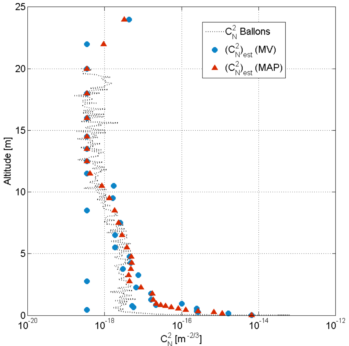
FIGURE 4.24 – Profil estimé pour les mesures P.M.L. du 25/01/2011 à 16h45minUT au Dôme C
