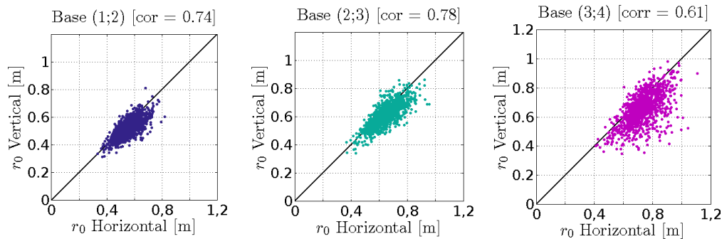
FIGURE 3.9 – Comparaison des r_0 obtenus à partir des variances différentielles des AA dans le sens horizontal et dans le sens vertical pour trois bases. Les bases utilisées exploitent des faisceaux voisins entre eux.
