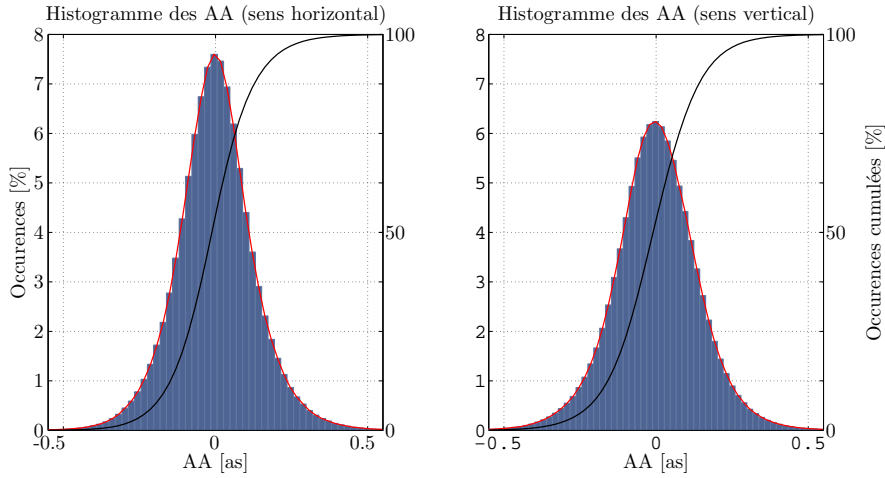
FIGURE 3.62 – Histogrammes des AA dans les deux directions pour l’ensemble des faisceaux pour les mesures dans la grande coupole du Mont Gros.
