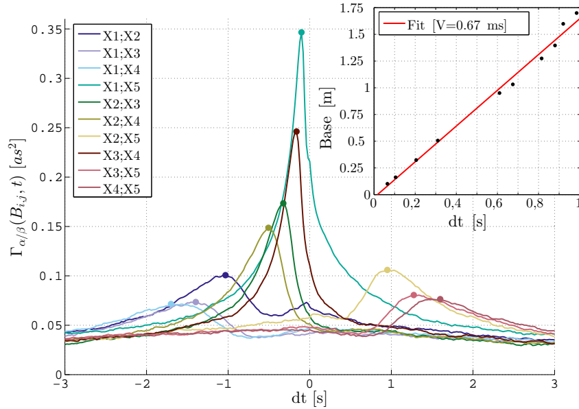
FIGURE 3.26 – Corrélations croisées des AA entre les différents faisceaux. La vitesse du vent est calculée à partir de la relation entre la base et la position du pic pour les différentes corrélations.
