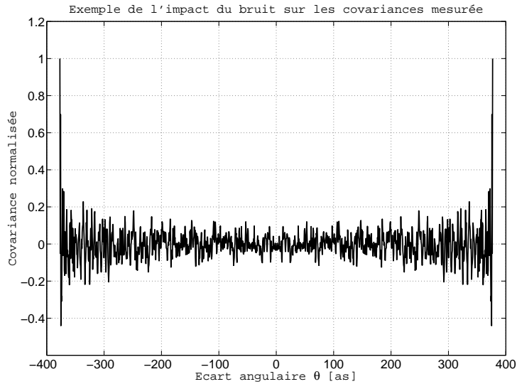
FIGURE 4.12 – Exemple de l’impact du bruit de photons sur une covariance moyenne obtenue via une dégradation par un bruit de Poisson d’une série de 1000 images artificielles.
