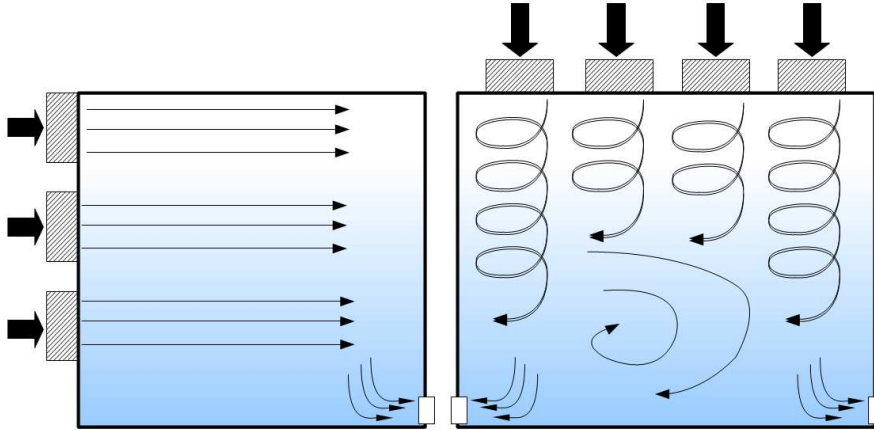
FIGURE 3.1 – Illustration des types de ventilations rencontrés dans les salles blanches étudiées. Le système le plus connu envoie un flux d'air laminaire comme illustré sur le schéma de gauche. Un flux d'air dit turbulent a aussi été rencontré et procède comme illustré sur la figure de droite.
