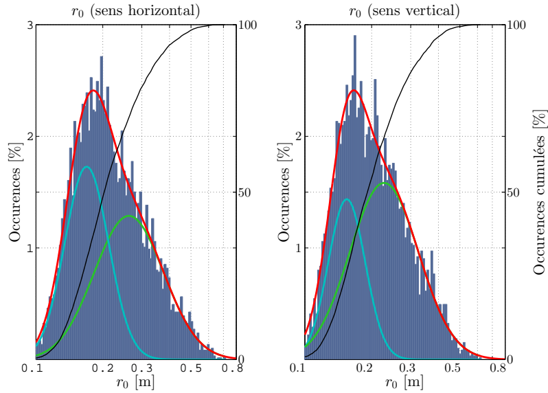
FIGURE 3.30 – Histogrammes des r_0 obtenus dans les deux directions (horizontale et verticale) à partir de l’ensemble des mesures différentielles. L’enveloppe tracée en rouge est obtenue par la combinaison des deux distributions log-normales tracées en bleu et en vert permettant l’ajustement des histogrammes.
