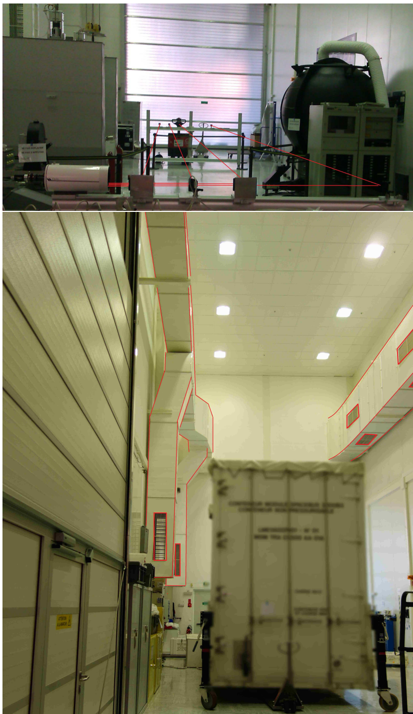
FIGURE 3.3 – Photographies du SAS matériel et du système de ventilation installé à l'intérieur. L'instrument INTENSE est visible sur la photographie du haut tandis que les conduits et grilles du système de ventilation sont surlignés en rouge sur la photographie du bas.
