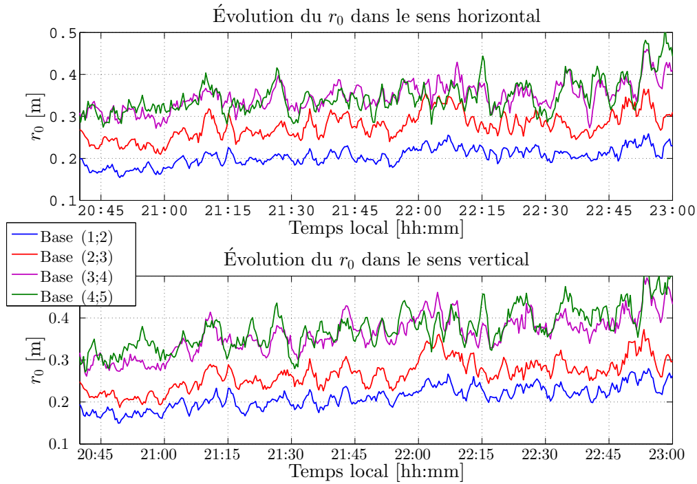
FIGURE 3.16 – Évolution du r_0 pendant la nuit du 19 au 20 juin 2014 pour différentes bases.
