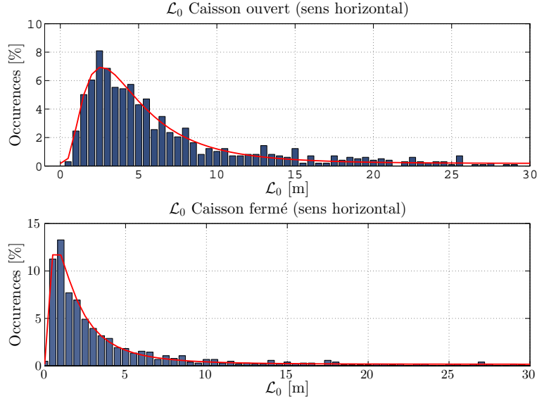
FIGURE 3.42 – Histogrammes des \mathcal{L}_0 obtenues à partir des AA dans la direction horizontale pour les situations caisson ouvert et fermé.
