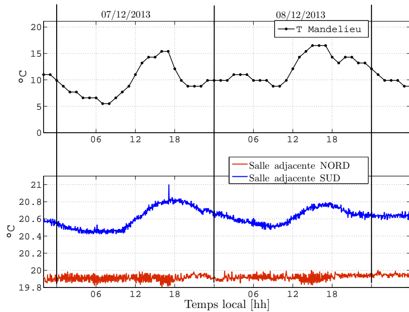
FIGURE 3.39 – Comparaison entre la température extérieure et celles obtenues dans les salles adjacentes au caisson.
