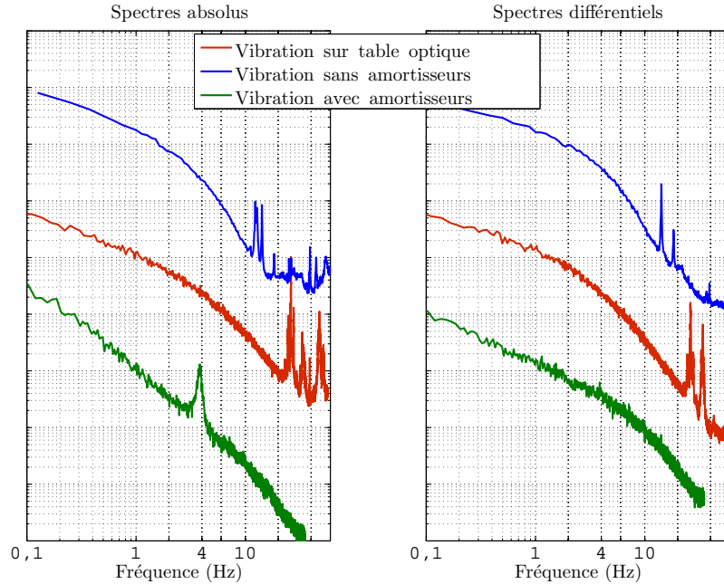
FIGURE 2.10 – Spectres obtenus pour des mesures de bruits mécaniques (bancs d’émission et de réception collés entre eux) dans différentes situations : profilés montés sur une table optique et instrument INTENSE avec/sans amortisseurs SLM.
