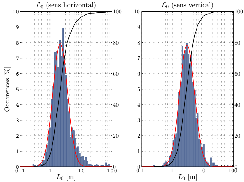
FIGURE 3.52 – Histogrammes des \mathcal{L}_0 obtenus à partir des variances des AA pour les mesures de décembre 2014.
