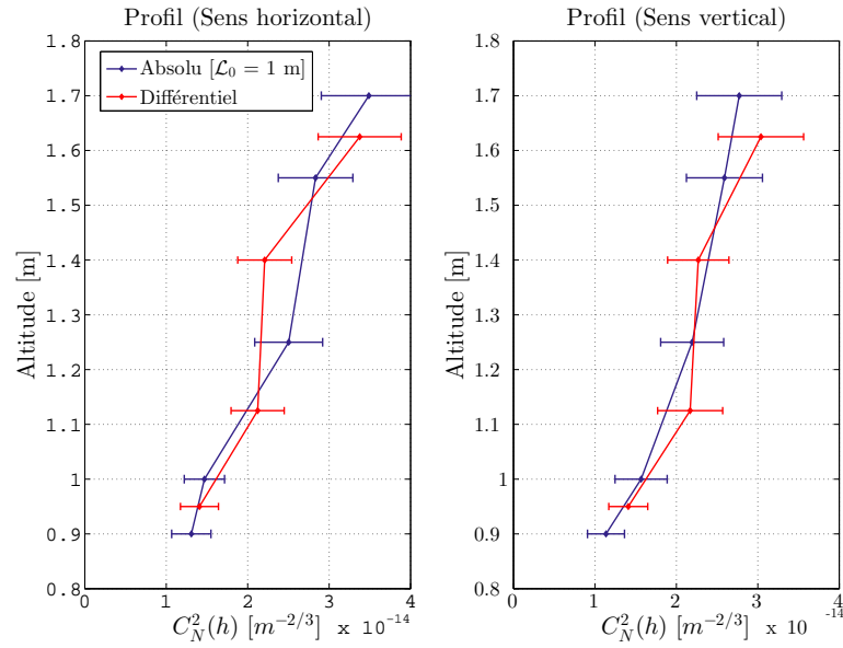
FIGURE 3.47 – Profil du C_n^2(h) obtenu à partir de la médiane et des écarts-types des C_n^2(h) obtenus à partir des variances absolues et différentielles des AA. L'échelle externe pour les variances absolues est considérée égale à \mathcal{L}_0 = 1\text{m} . Seules les bases contenant les faisceaux voisins sont tracées pour les mesures différentielles.
