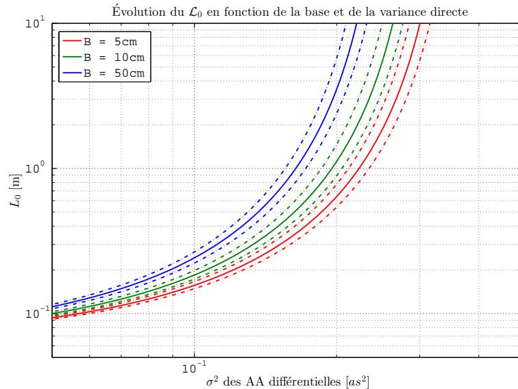
FIGURE 2.13 – Sensibilité du \mathcal{L}_0 aux erreurs sur les variances absolues des AA pour différentes bases.
