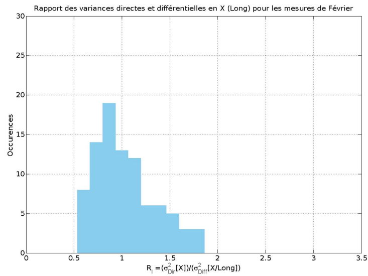
FIGURE 13 – Histogramme du rapport R en x avec une base longitudinale pour les mesures de Février L_0(l) médian égale à 1.2550 mètres
