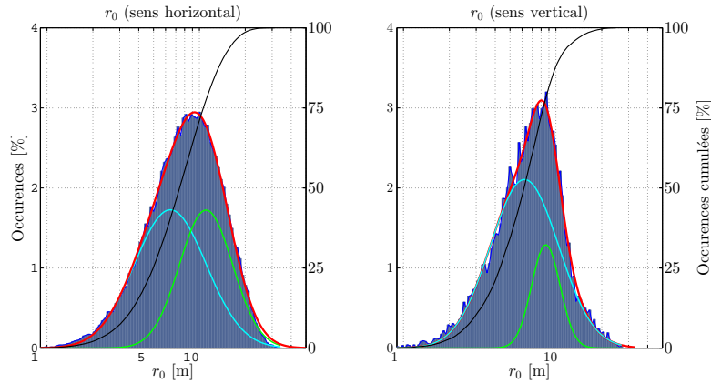
FIGURE 3.59 – Histogrammes des r_0 dans les deux directions pour différentes bases.
