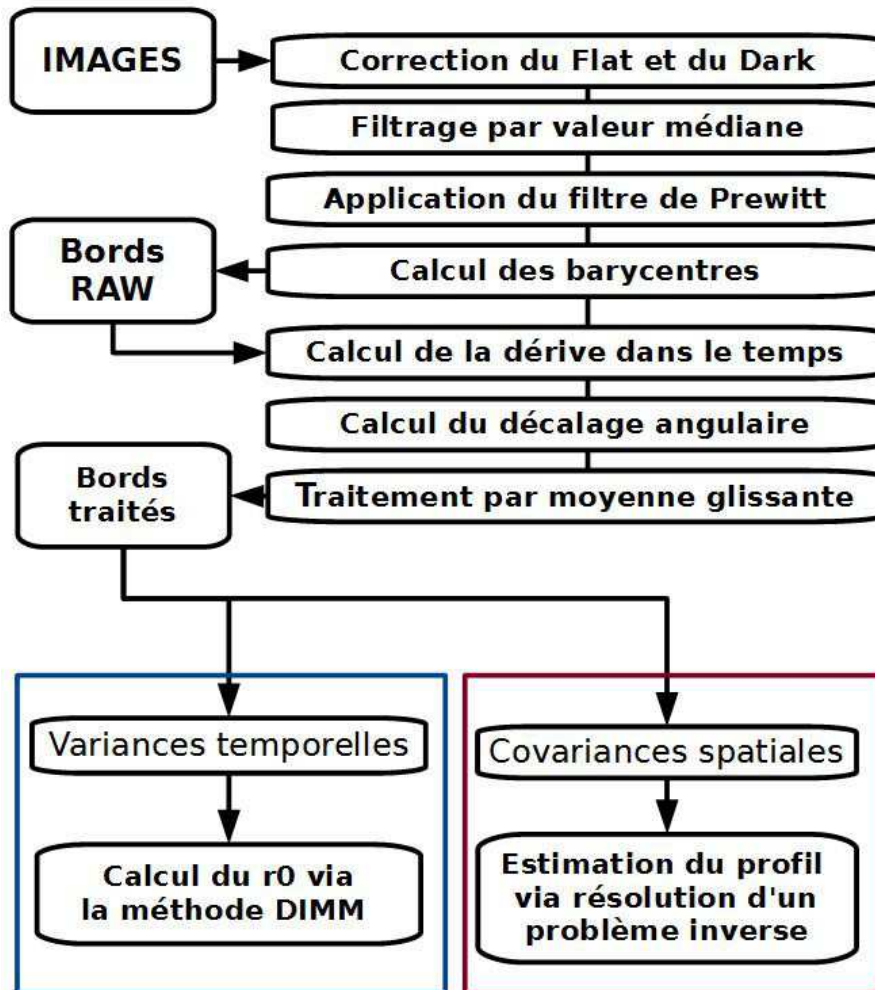
FIGURE 4.19 – Diagramme des étapes de l’algorithme de pré-traitement.
