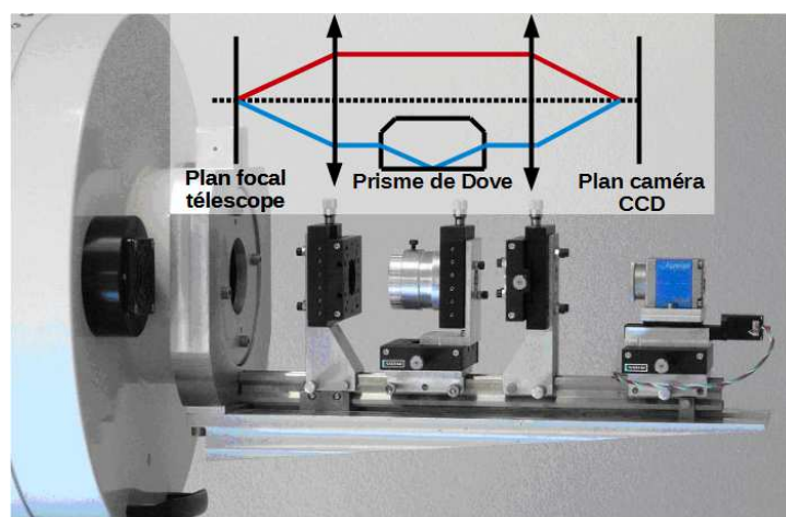
FIGURE 4.10 – Photographie du dispositif optique de l'instrument PML.
