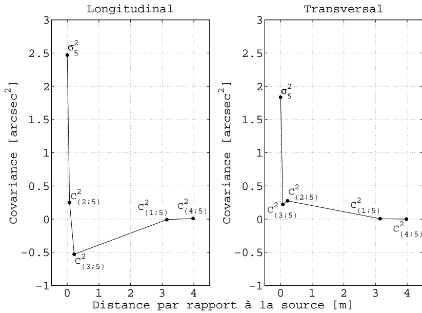
FIGURE 4.30 – Covariances entre le faisceau croisé et les autres signaux laser avec l'utilisation d'une bougie comme source de chaleur. La covariance est tracée en fonction de la distance entre la source de chaleur et le faisceau concerné. Dans le cas ci-dessus, la bougie était située entre les faisceaux 2 et 3.
