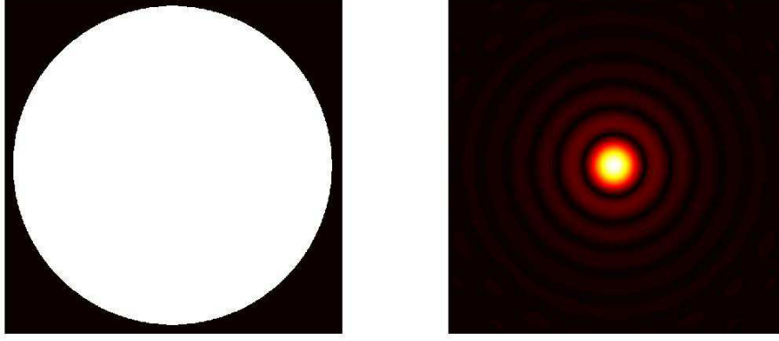
FIGURE 1.3 – Représentation de la fonction pupille et de sa FEP associée.
