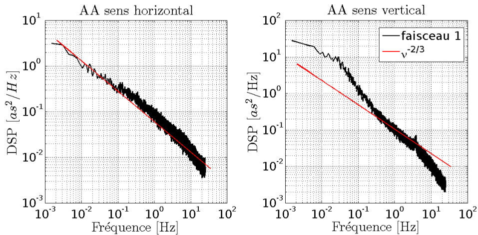
FIGURE 3.25 – DSP des fluctuations des AA dans le sens horizontal et vertical pour les mesures dans la salle à fort flux d'air.
