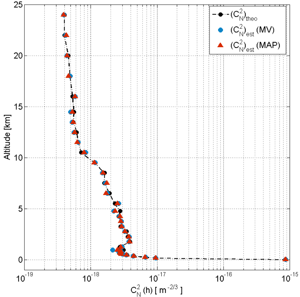
FIGURE 4.22 – Profils estimés à partir de covariances théoriques affectées par un bruit de photons.
