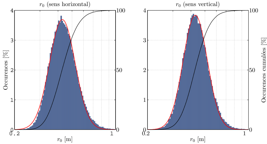
FIGURE 3.51 – Histogrammes des r_0 pour l’ensemble des mesures différentielles. Les r_0 obtenus à partir des variances différentielles des AA pour les deux directions sont présentés. Les AA exploités pour cette figure sont les mesures obtenues en décembre 2014. Une loi log-normale en rouge ajuste les histogrammes tandis que les fonctions de répartition sont tracées en noir.
