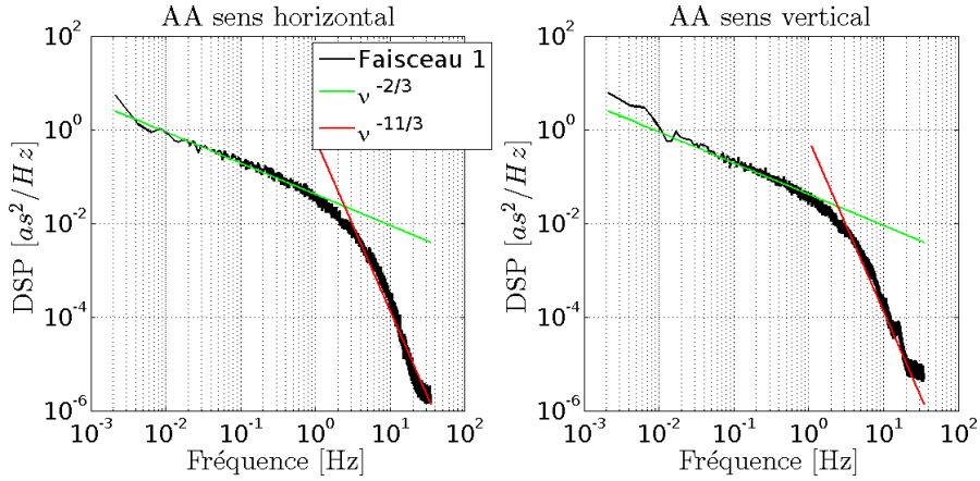
FIGURE 3.33 – DSP des fluctuations des AA dans les deux directions (horizontale et verticale). Les tendances en -2/3 et -11/3 sont tracées sur la même figure.
