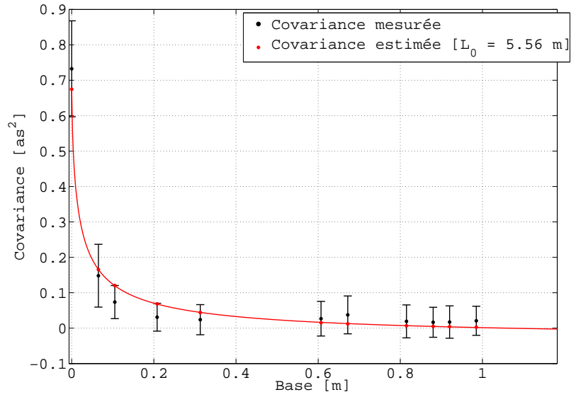
FIGURE 3.23 – Covariance médiane obtenue à partir des mesures des AA pour l’ensemble des faisceaux. Les barres d’erreurs correspondent aux écart-types des mesures. La covariance théorique pour le modèle de Von-Kàrmàn ajustant au mieux les données est tracée en rouge.
