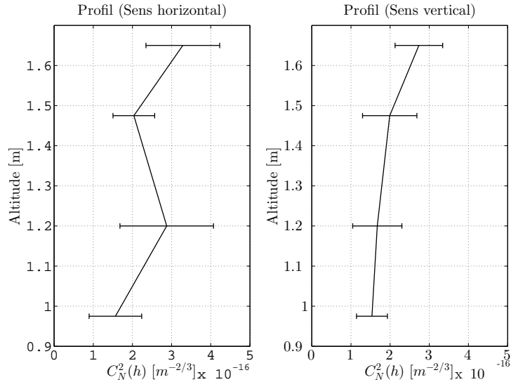
FIGURE 3.58 – Profil des mesures du C_n^2(h) obtenu à partir de la médiane et des écarts-types des C_n^2(h) via les variances différentielles des AA pour les mesures de décembre 2014.
