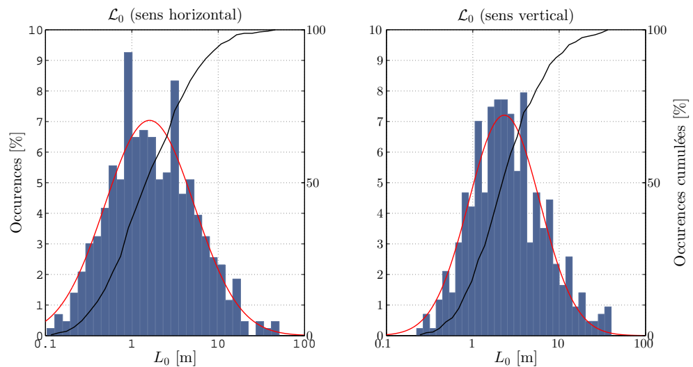
FIGURE 3.66 – Histogrammes du \mathcal{L}_0 obtenus à partir des variances des AA dans le sens horizontal et vertical. Une distribution log-normale ajustant les données est tracée conjointement en rouge tandis qu'une fonction de répartition est dessinée en noir.
