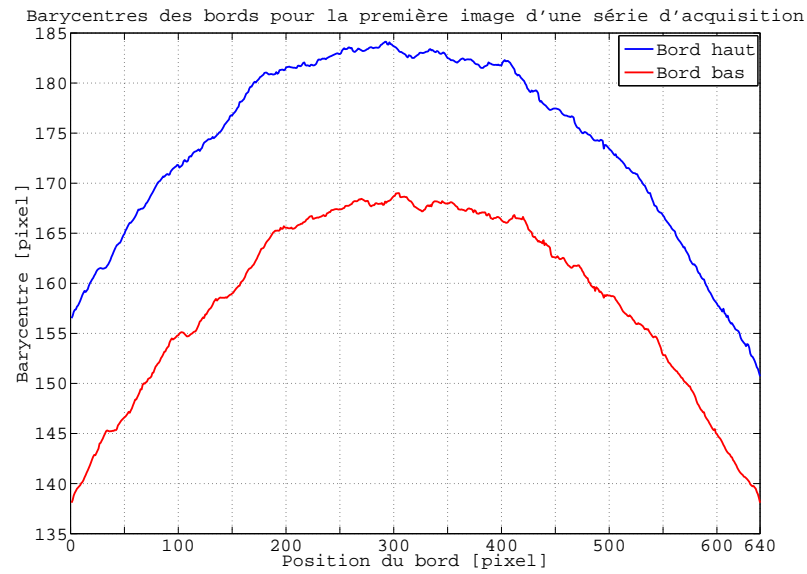
FIGURE 4.15 – Exemples de bords obtenus par calcul barycentrique d'une image du limbe de la lune. Deux bords (haut et bas) sont obtenus pour chaque image du fait de l'exploitation d'un couple de sous-pupilles.
