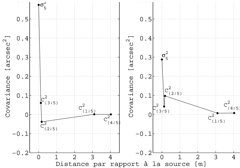
FIGURE 4.31 – Covariances entre le faisceau croisé et les autres signaux laser avec l'utilisation d'une bougie comme source de chaleur. Cette dernière a été déplacée de 5cm en direction du faisceau n°3.
