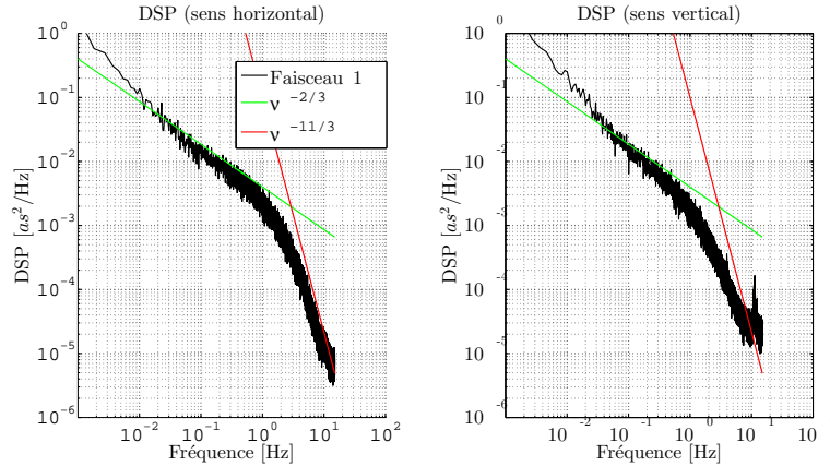
FIGURE 3.67 – DSP des fluctuations des AA dans les deux directions. Les tendances en -2/3 et en -11/3 sont tracées sur la même figure.
