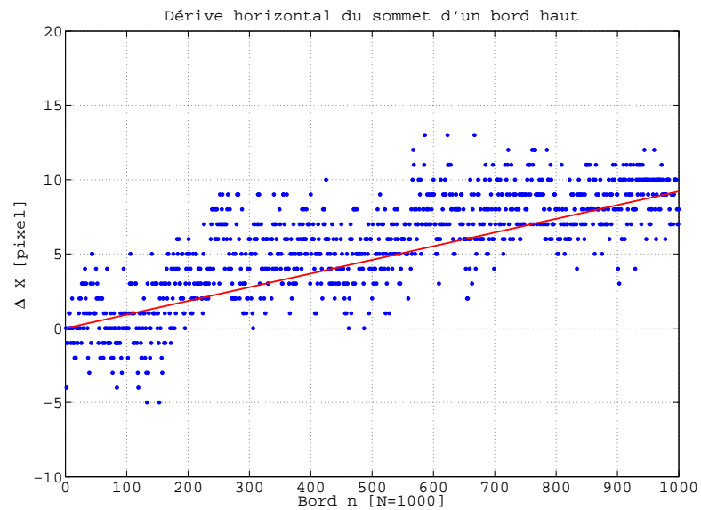
FIGURE 4.16 – Exemple d'une dérive horizontale des mesures observées sur une série de N=1000 bords obtenus à partir du limbe de la lune.
