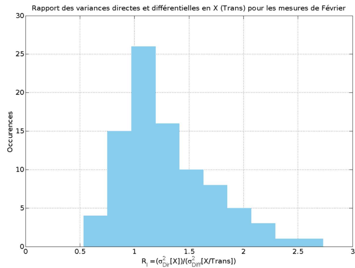
FIGURE 15 – Histogramme du rapport R en x avec une base transversale pour les mesures de Février. L_0(t) médian égale à 0.2685 mètre
