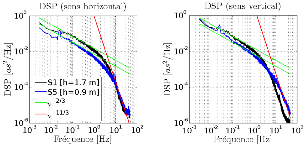
FIGURE 3.54 – DSP des fluctuations des AA issues des mesures de décembre 2014 dans les deux directions. Les tendances en -2/3 et -11/3 sont tracées sur la même figure.
