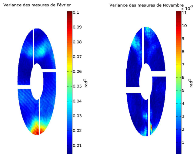
FIGURE 2 – Moyenne des mesures de Février et de Novembre en radian
