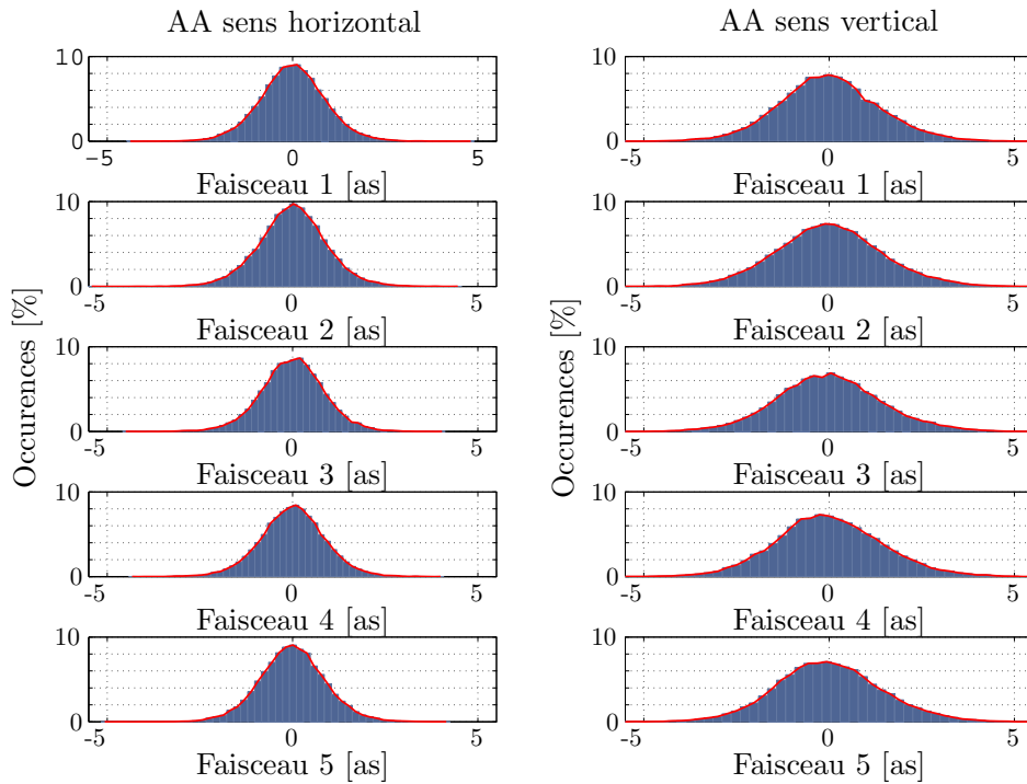
FIGURE 3.20 – Histogrammes des AA pour chaque faisceau dans les deux directions de mesure.
