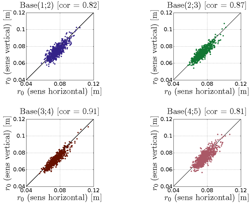
FIGURE 3.21 – Comparaisons entre les estimations du r_0 à partir des variances différentielles des AA dans le sens horizontal et vertical.
