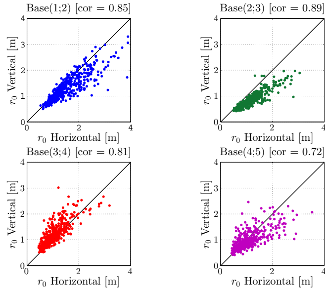
FIGURE 3.63 – Comparaison des r_0 obtenus à partir des variances différentielles des AA dans le sens horizontal et dans le sens vertical pour différentes bases. Les bases utilisées correspondent à celles des faisceaux voisins.
