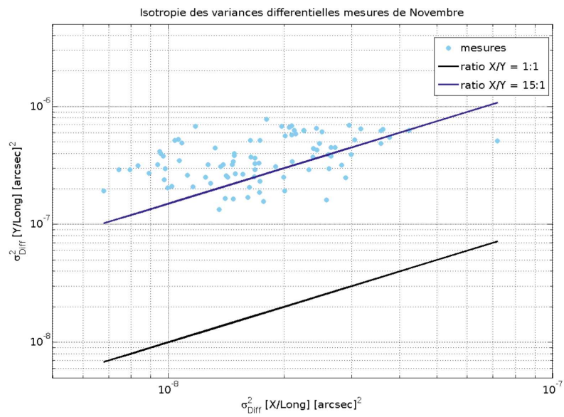
FIGURE 9 – Variance des fluctuations d’AA pour le mois de Novembre
