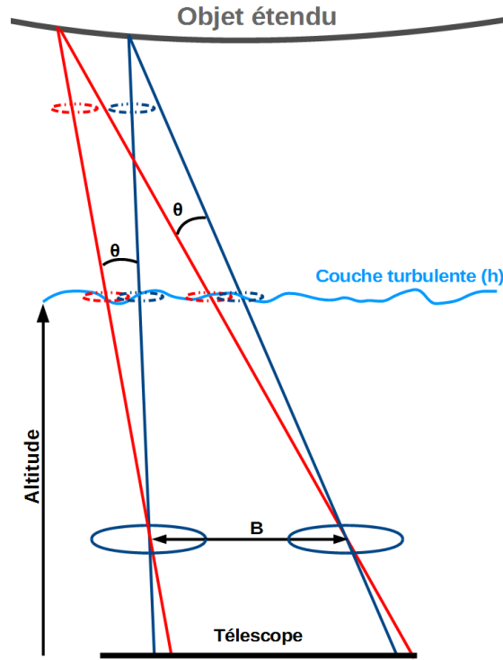
FIGURE 4.2 – Schéma de principe de la mesure différentielle des fluctuations des AA à partir d'un objet étendu pour un écart angulaire \theta .
