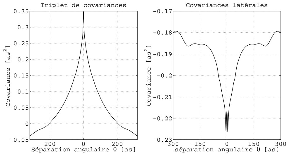
FIGURE 4.7 – Exemple d’une covariance différentielle obtenue par addition des différentes contributions des couches de l’atmosphère. Le profil utilisé pour le calcul est celui de la figure 4.8. A gauche se trouve la covariance différentielle et à droite est tracée la contribution des covariances latérales.
