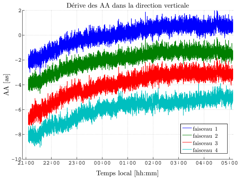
FIGURE 3.4 – Dérives dans le sens vertical des AA pour les différents faisceaux. Ces dérives sont principalement liées à la relaxation des amortisseurs SLM.
