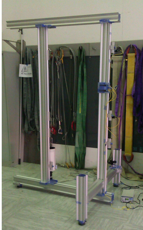
FIGURE 2.7 – Configuration d'essai de la structure verticale de l'instrument INTENSE permettant une étude de la stratification de la turbulence optique.
