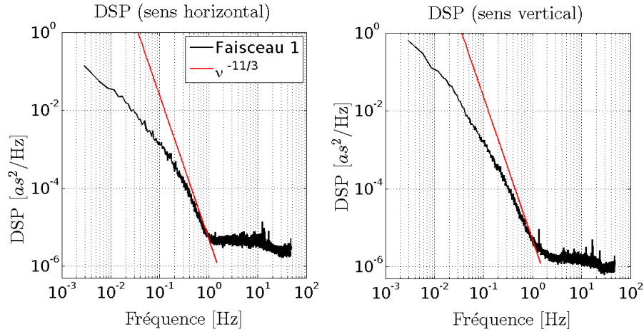
FIGURE 3.60 – DSP des fluctuations des AA issus des mesures de décembre 2014 dans les deux directions. La tendance en -11/3 est tracée sur la même figure.
