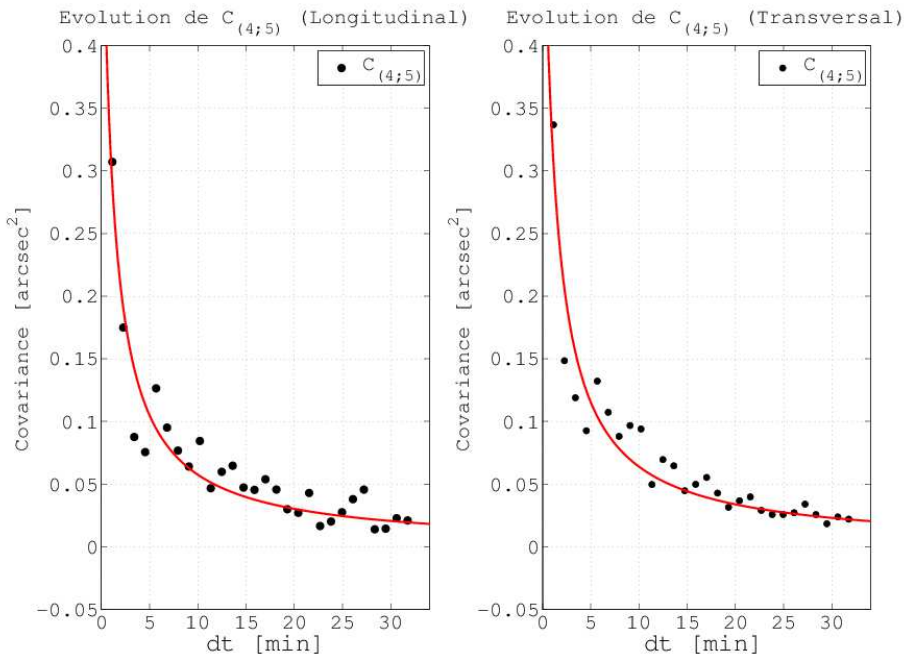
FIGURE 4.28 – Évolution de la covariance C_{(4;5)} dans le temps. L'impact de la chaleur dégagée par le profilé sur la covariance est ici clairement visible. Les valeurs de C_{(4;5)} baissent au fur et à mesure du refroidissement de la barre métallique.
