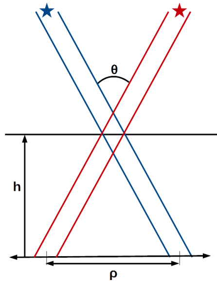
FIGURE 4.1 – Schéma de principe de la mesure du profil à partir d'une source double.
