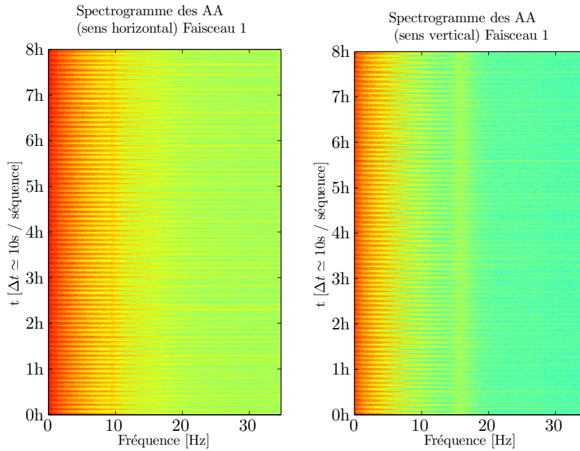
FIGURE 3.34 – Spectrogrammes des AA dans les deux directions. Les spectres sont obtenus à partir de séquences d’acquisition d’environ 10 secondes.
