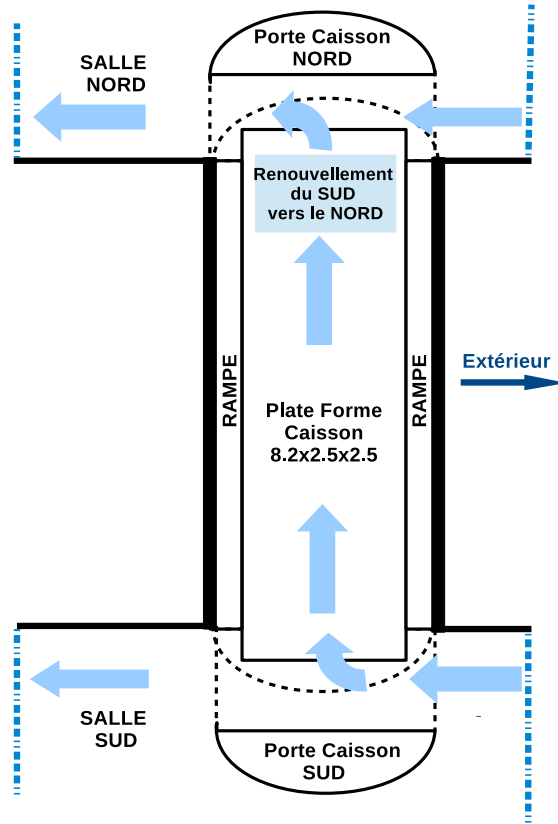
FIGURE 3.27 – Schéma du caisson et de la propagation du vent dans l'enceinte.
