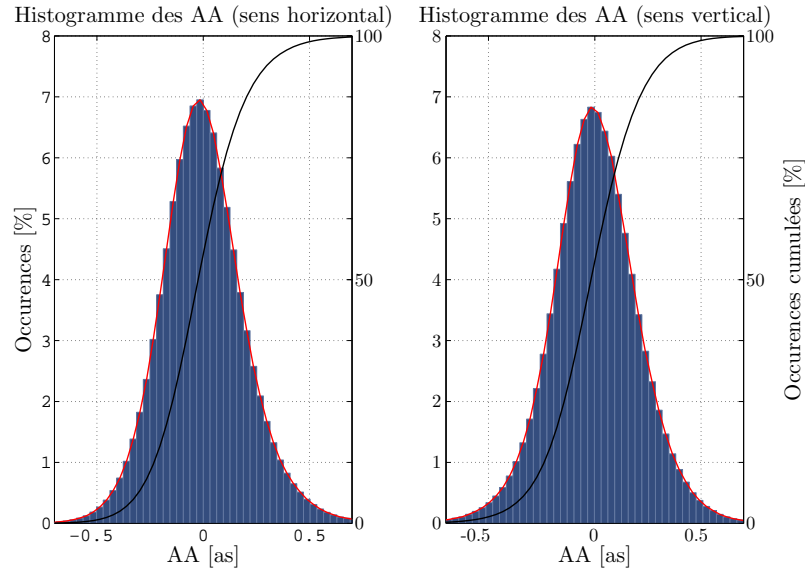
FIGURE 3.45 – Histogrammes des AA dans les directions horizontale et verticale. Les histogrammes sont obtenus à partir de l’ensemble des acquisitions des différents faisceaux. Une fonction de répartition est tracée en noir sur la figure.
