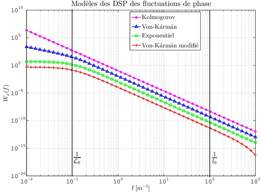
FIGURE 1.5 – Représentation des DSP des fluctuations de la phase pour différents modèles. Les différentes courbes sont tracées décalées entre elles pour plus de visibilité. Les échelles externe et interne sont respectivement égales à \mathcal{L}_0 = 10\text{m} et l_0 = 1\text{cm}
