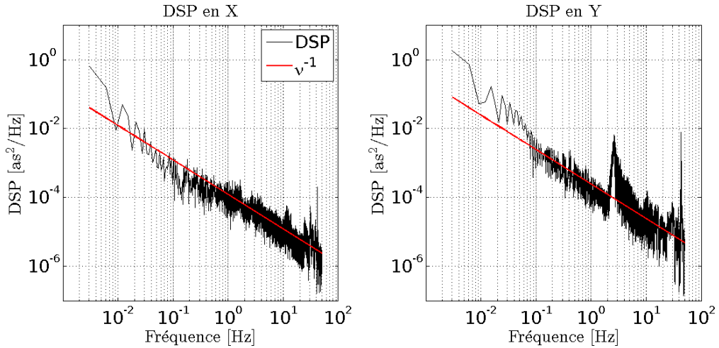
FIGURE 2.8 – DSP de l'instrument INTENSE en configuration verticale pour des mesures de bruits (bancs collés).
