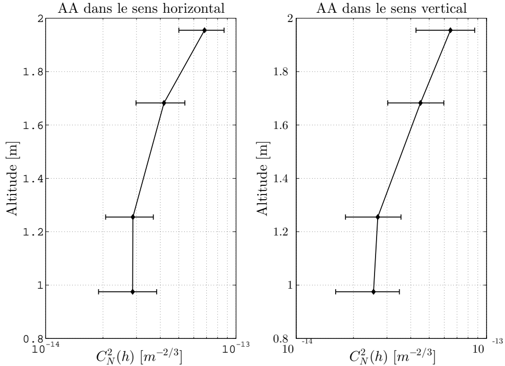
FIGURE 3.17 – Profil du C_n^2(h) à partir des mesures différentielles pour différentes altitudes médianes. Seules les bases exploitant des faisceaux voisins sont représentées.
