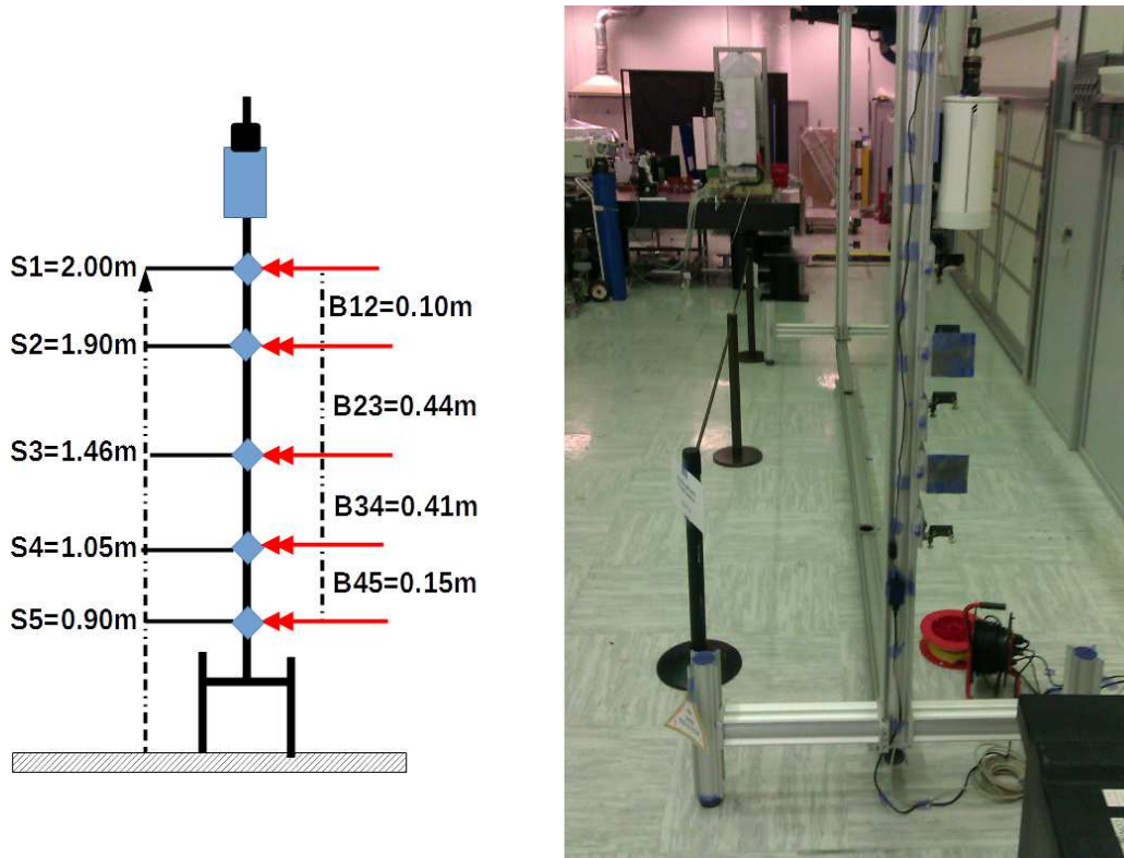
FIGURE 3.14 – Schéma et photographie de l'instrument INTENSE dans la configuration verticale pour les mesures dans le SAS.
