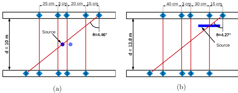
FIGURE 4.25 – Configuration de l'instrument INTENSE dans les deux cas étudiés. A gauche se trouve le cas d'une bougie installée à quelques centimètres sous les faisceaux n°2 et 3 au niveau de la zone de croisement avec le faisceau n°5. À droite se trouve le cas d'un profilé X95 précédemment chauffé et placé sous le croisement entre les faisceaux n°4 et n°5.
