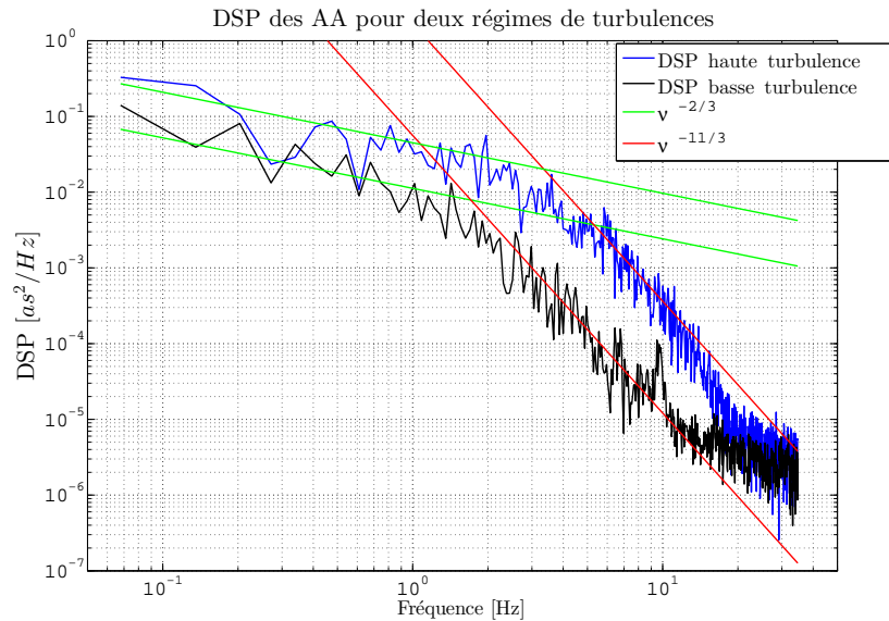
FIGURE 3.35 – DSP issues du spectrogramme des AA pour les mesures longitudinales. Les deux tendances extrêmes obtenues dans la figure 3.34 sont tracées sur celle-ci.
