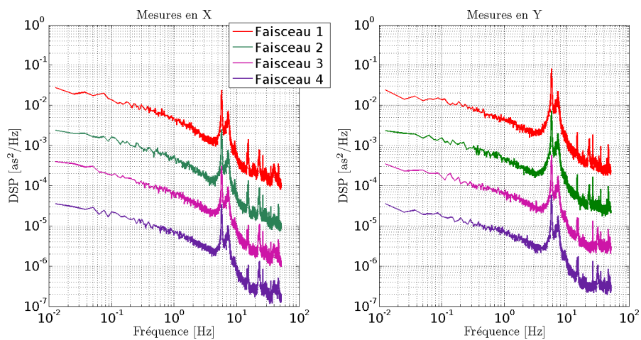
FIGURE 2.4 – Exemple de spectres du bruit mécanique obtenus à partir de la configuration initiale de l'instrument INTENSE en l'absence d'amortissement.
