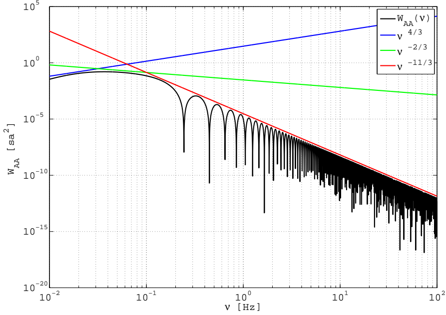
FIGURE 1.7 – DSP théorique des fluctuations des AA pour le modèle de Von-Kàrmàn. Les tendances usuelles sont également tracées.
