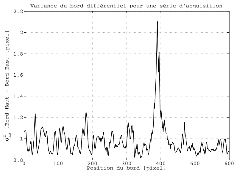
FIGURE 4.18 – Exemple d'écart important entre les pixels voisins du fait de la présence de détails (cratères, mers) non loin du limbe observé.
