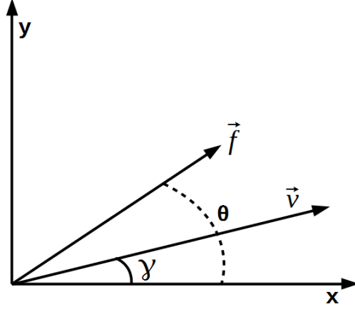
FIGURE 1.6 – Schéma d'illustration permettant la représentation du vecteur vitesse \vec{v} et du vecteur \vec{f} dans le référentiel x,y .
