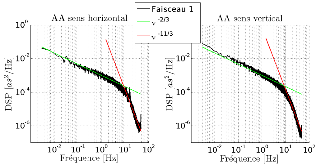
FIGURE 3.18 – DSP des fluctuations des AA dans le sens horizontal et vertical. Les tendances en -2/3 et -11/3 sont tracées sur la même figure.
