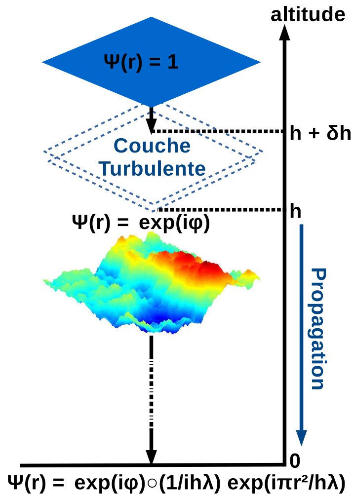
FIGURE 1.2 – Schéma décrivant la propagation d’une onde plane à travers une couche de turbulence.
