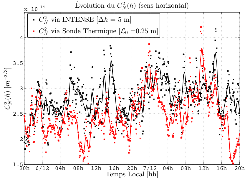
FIGURE 3.56 – C_n^2(h) calculés à partir des variances des AA dans le sens horizontal obtenus par l'instrument INTENSE et à partir de sondes thermiques. Le \mathcal{L}_0 global de 25cm permet de s'approcher au mieux des résultats obtenus par l'instrument INTENSE.
