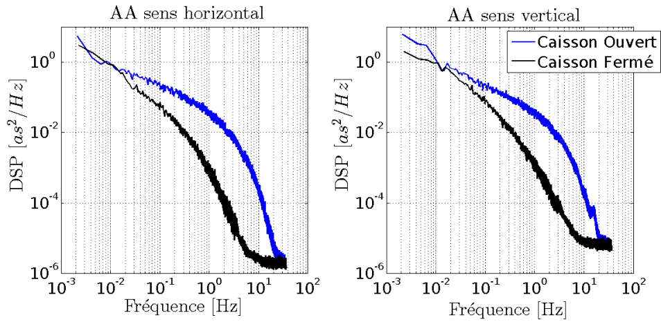
FIGURE 3.43 – Comparaison des DSP dans les cas caisson ouvert et caisson fermé. L'impact du système de ventilation sur l'énergie de la turbulence est ici clairement visible.
