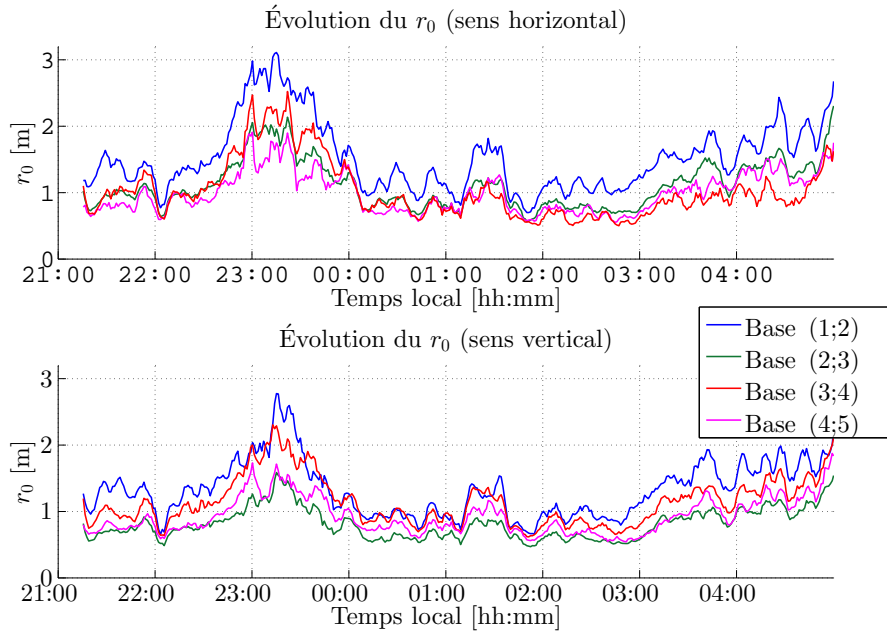
FIGURE 3.64 – Évolution des mesures du r_0 pendant la nuit du 15 au 16 septembre 2014 pour différentes bases. Les bases utilisées correspondent à celles des faisceaux voisins
