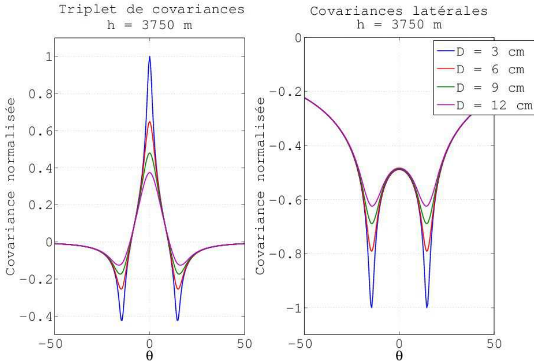
FIGURE 4.5 – Influence du diamètre D des sous-pupilles sur les covariances théoriques. A gauche le triplet de covariances pour une altitude h=3750\text{m} , à droite les covariances latérales pour la même altitude.
