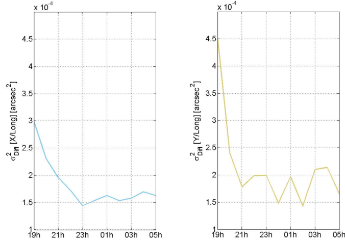
FIGURE 12 – Variance différentielle , base longitudinale en x/y, des fluctuations d'AA , mois de Novembre
