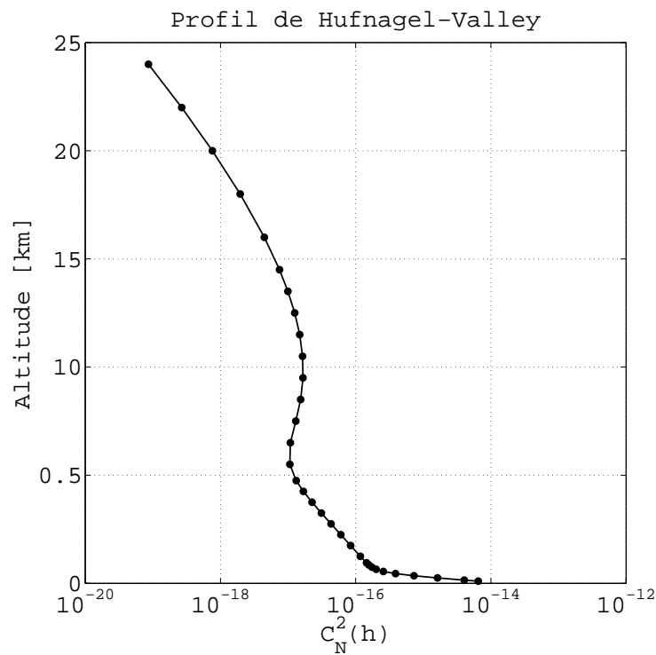
FIGURE 4.8 – Profil théorique obtenu à partir d’un modèle Hufnagel-Valley via l’exploitation des couches du tableau 4.1.
