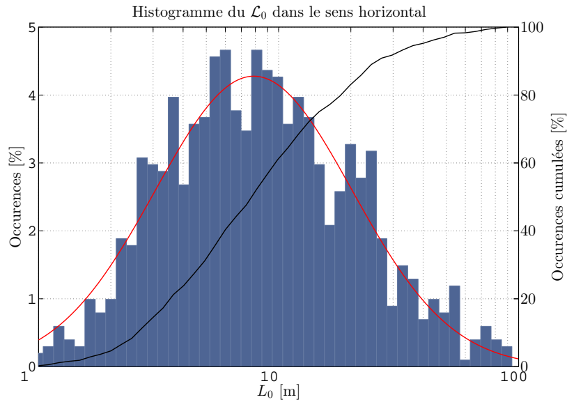
FIGURE 3.36 – Histogramme du \mathcal{L}_0 obtenu à partir des variances des AA dans le sens horizontal. Une distribution log-normale ajustant au mieux les données est tracée conjointement en rouge tout comme la fonction de répartition tracée en noir.
