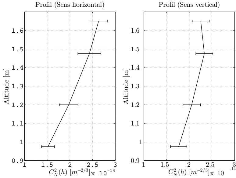
FIGURE 3.48 – Profil du C_n^2(h) obtenu à partir de la médiane et des écarts-types des C_n^2(h) via les variances différentielles des AA pour les mesures de décembre 2014.
