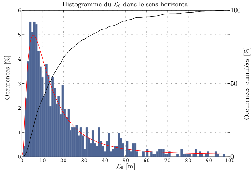
FIGURE 3.12 – Histogramme des \mathcal{L}_0 obtenu à partir des variances absolues des AA dans le sens horizontal. L’ajustement des données par une distribution log-normale est tracé en rouge. La fonction de répartition est tracée en noir.
