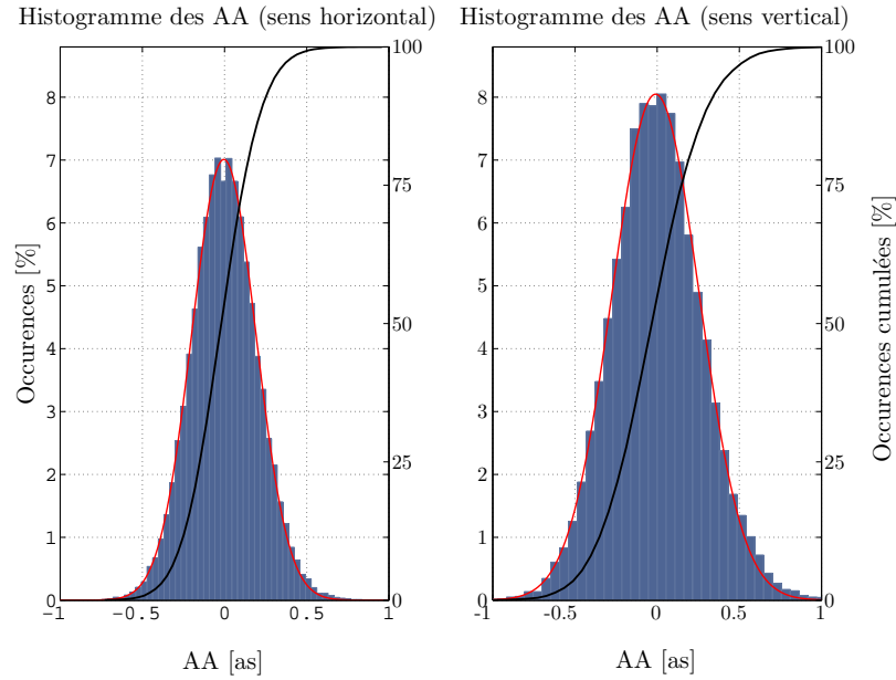
FIGURE 3.6 – Histogrammes des AA dans le sens horizontal et vertical pour l’ensemble des mesures obtenues par les différents faisceaux. La courbe noire correspond à la fonction de répartition des AA.
