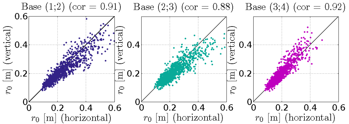
FIGURE 3.32 – Comparaison des r_0 obtenus à partir des variances différentielles des AA dans le sens horizontal et dans le sens vertical pour trois bases. Les bases utilisées correspondent aux couples de faisceaux voisins.
