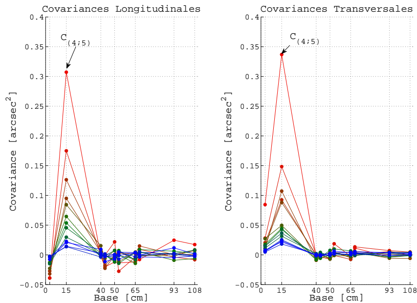
FIGURE 4.27 – Covariance à partir des différentes bases pour les mesures avec le profilé. Ce dernier refroidit avec le temps (du rouge vers le bleu) ce qui a une influence sur les résultats. La covariance des faisceaux se croisant au dessus du profilé est grandement affectée par la turbulence artificielle au contraire des bases plus éloignées.
