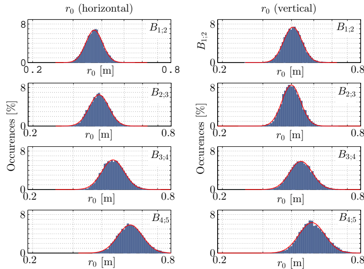
FIGURE 3.49 – Histogrammes des r_0 dans les deux directions pour différentes bases. Les histogrammes sont obtenus à partir des variances différentielles des mesures de décembre 2014.
