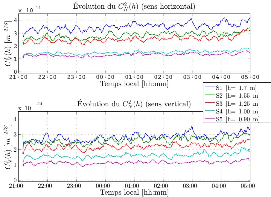
FIGURE 3.46 – Évolution du C_n^2(h) pour chaque faisceau obtenu à partir des variances absolues des AA. L'échelle externe est ici considérée égale à \mathcal{L}_0 = 1\text{m} .
