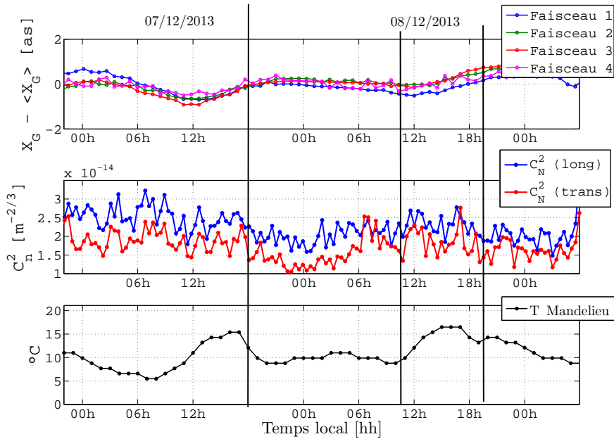
FIGURE 3.40 – Comparaison entre la position médiane des faisceaux sur la caméra CCD, les C_N^2(h) issus des variances différentielles et les mesures de température de l’air extérieur.
