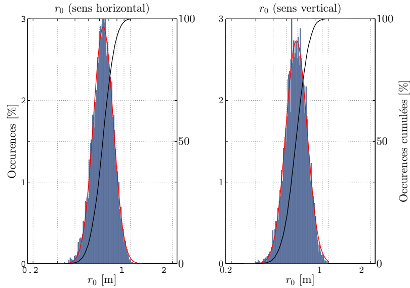
FIGURE 3.11 – Histogrammes des r_0 obtenus dans les deux directions à partir de l'ensemble des mesures différentielles. Les histogrammes sont représentés en échelle logarithmique et une fonction gaussienne obtenue par ajustement des données est tracée conjointement en rouge. Les fonctions de répartition sont aussi tracées en noir sur la figure.
