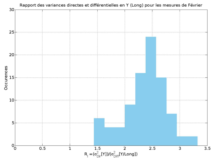
FIGURE 14 – Histogramme du rapport R en y avec une base longitudinale pour les mesures de Février. L_0(l) médian égale à 0.0231 mètre
