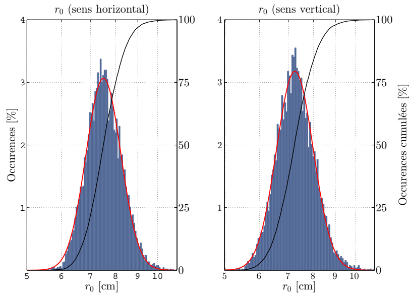
FIGURE 3.22 – Histogrammes des r_0 obtenus à partir de l’ensemble des mesures. L’ajustement des histogrammes par des fonctions de distribution gaussienne (en rouge) et les fonctions de répartition (en noir) sont tracées sur la figure.
