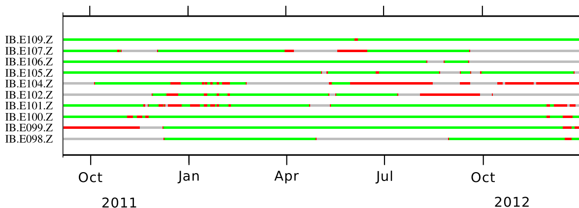
FIGURE 1.1 : Taux de fonctionnement journalier sur la composante verticale de 10 stations du réseau IberArray (Díaz et al., 2009). Une couleur grise indique un taux de fonctionnement nul. Une couleur rouge indique un taux de fonctionnement non nul inférieur à 90%. Une couleur verte indique un taux de fonctionnement supérieur à 90%.
