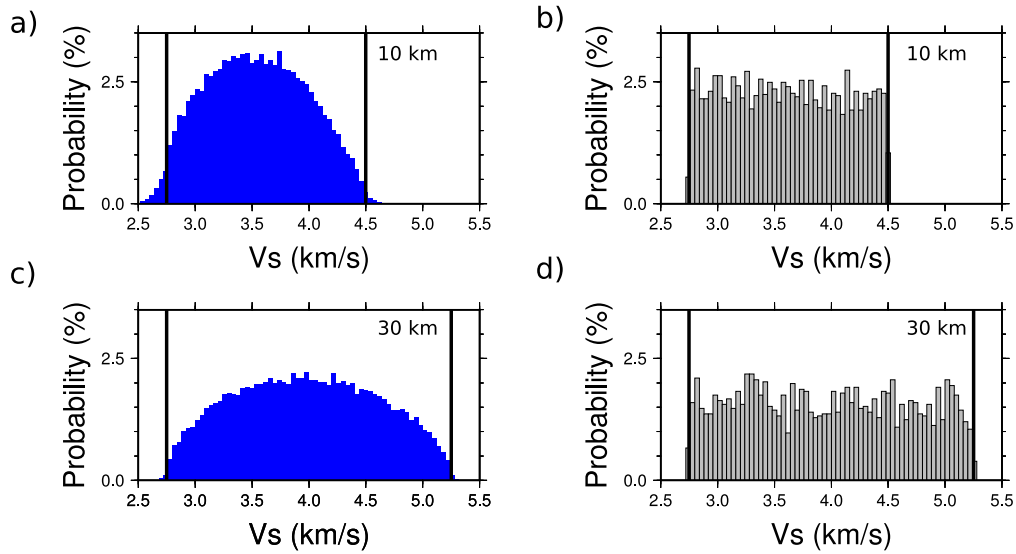
FIGURE 4.7 : Densités de probabilité marginale a priori à 10 km (a et b) et 30 km de profondeur (c et d) calculées sur les modèles de vitesse continu (a et c) et sur les points de Bézier (b et d). La taille des intervalles est de 0.04 km/s. Les lignes noires verticales indiquent les bornes du prior.
