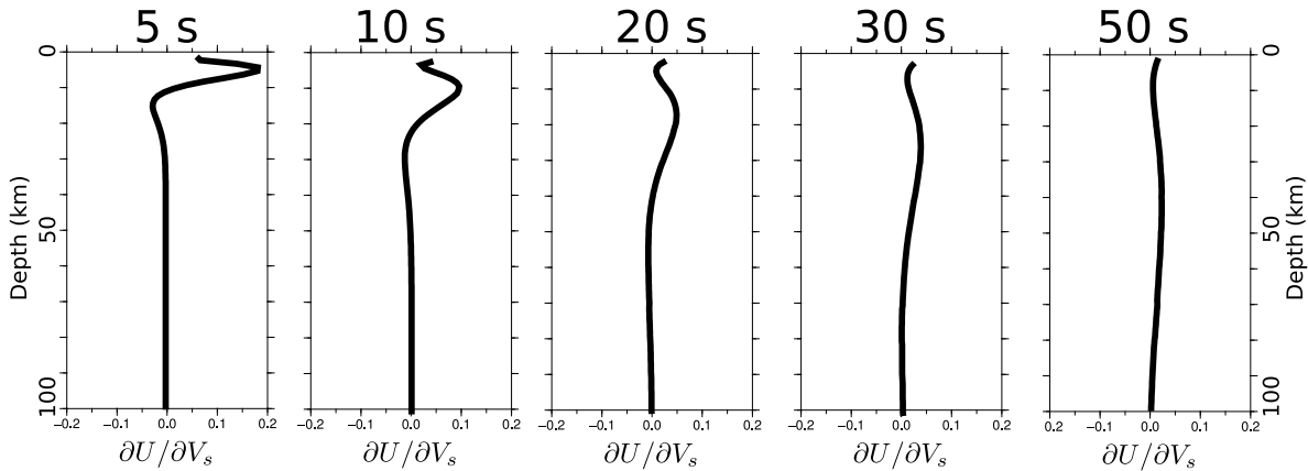
FIGURE 4.1 : Sensibilité de la vitesse de groupe du mode fondamental des ondes de Rayleigh à la vitesse sismique cisailante en fonction de la profondeur, pour 5, 10, 20, 30, et 50 s de période. Les noyaux de sensibilités, non normalisés, ont été calculés dans un modèle de terre 2 couches de type croûte-manteau (Computer Programs in Seismology, Herrmann, 2013 ).
