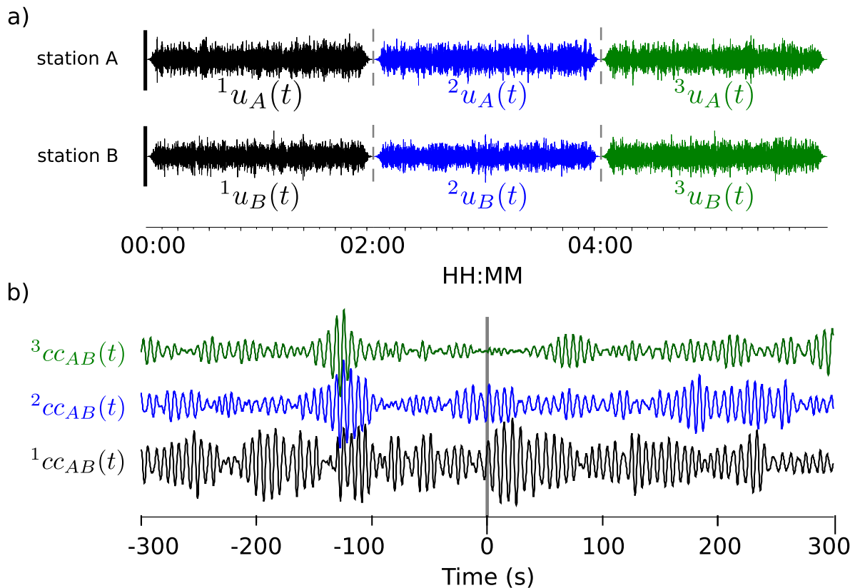
FIGURE 1.4 : Illustration du calcul des intercorrélations individuelles. a) Extraction de segments de 2h à deux stations A et B. Un fenêtrage en cosinus amorti est appliqué sur les bords de chaque fenêtre. b) Intercorrélations individuelles calculées entre les stations A et B associées à chaque segment.
