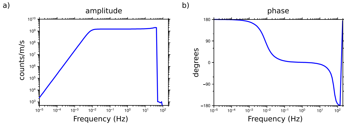
FIGURE 1.2 : Réponse instrumentale de la station large bande PY41 pour le canal HHZ. a) réponse en amplitude, b) réponse en phase.
