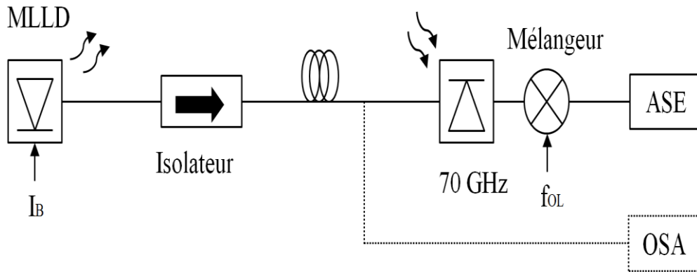
Figure 2.23. Banc de mesure : spectre optique et spectre RF
