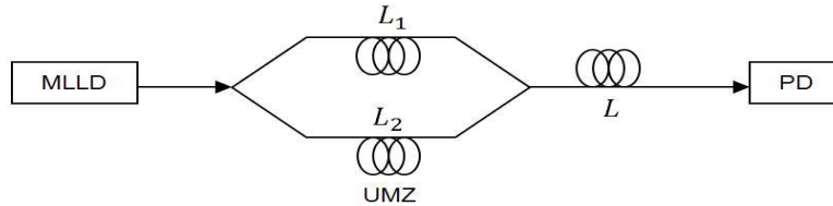
Figure 3.44. Schéma du système pour réduire la sensibilité à la dispersion chromatique
