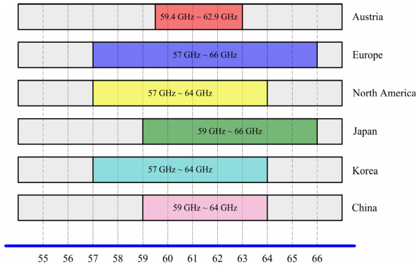
Figure 1.1. Spectres autorisés dans la bande de 60 GHz suivant les organismes de standardisation [2]
