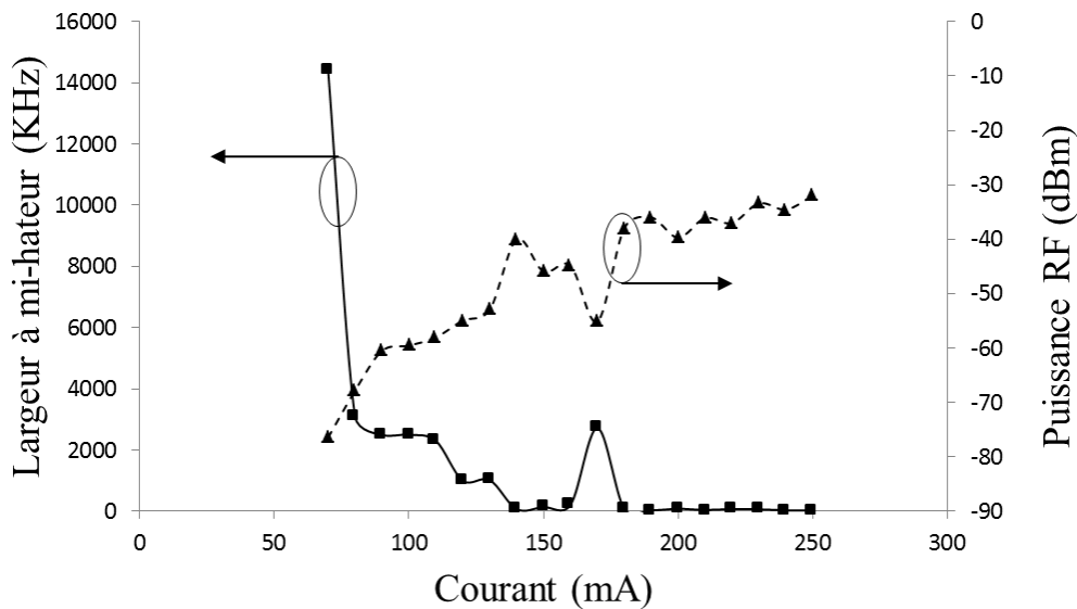
Figure 2.24. Variation de la puissance RF (signal généré par le battement) et de la largeur à mi-hauteur du laser L872 en fonction du courant de polarisation
