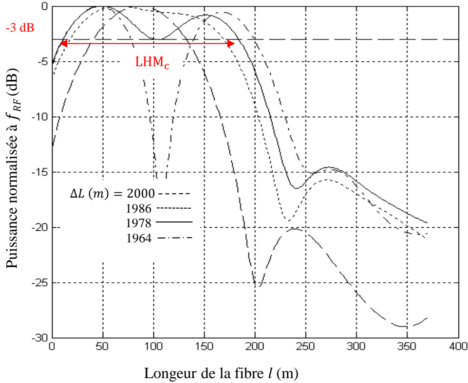
Figure 3.50. Variation de la puissance RF en fonction de la longueur L du SMF
