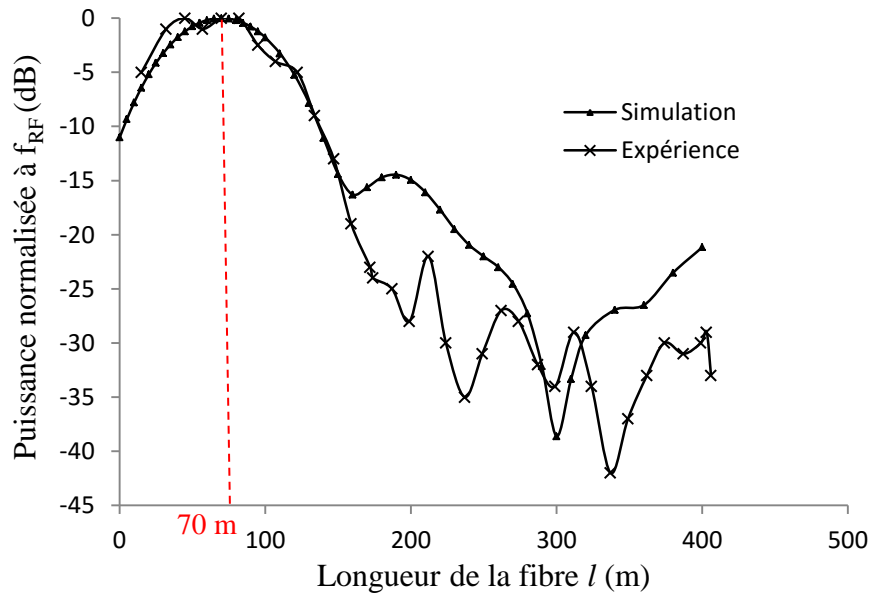
Figure 3.43. Variation de la puissance RF en fonction de la longueur de la fibre (expérience et simulation)
