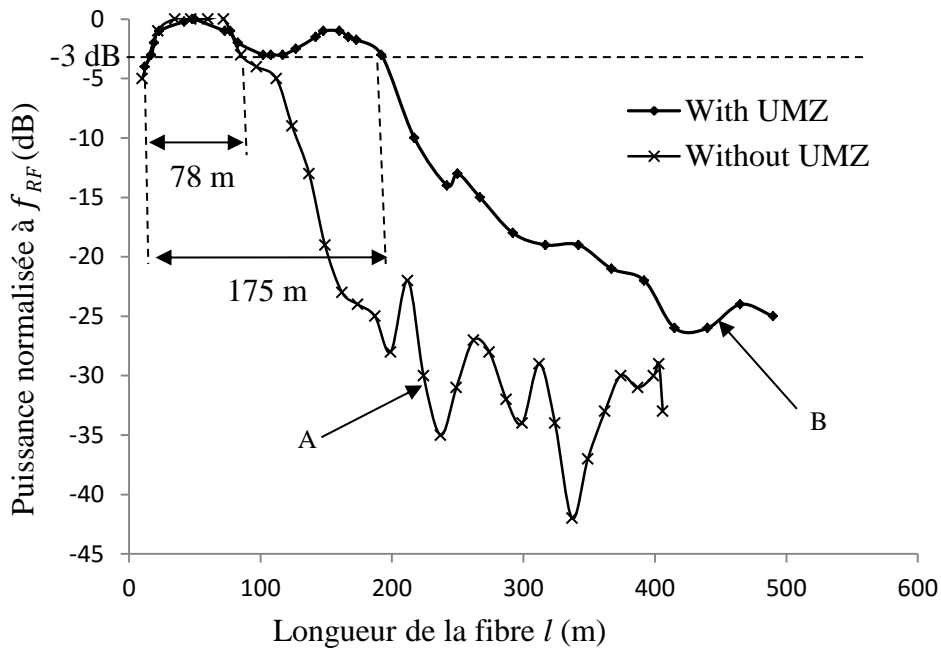
Figure 3.49. Résultats expérimentaux: variation de la puissance RF par rapport à la longueur de la fibre SMF sans, (A), et avec, (B), l'UMZ
