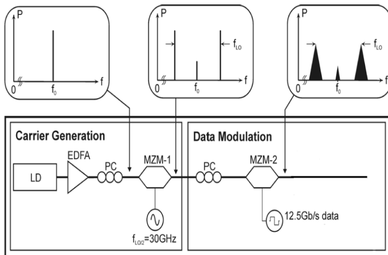
Figure 1.7. Génération des ondes mmW avec deux MZM [17]
