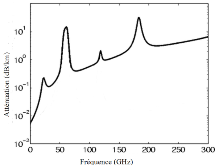
Figure 1.2. Spectre d'atténuation de la molécule de l'oxygène [46]
