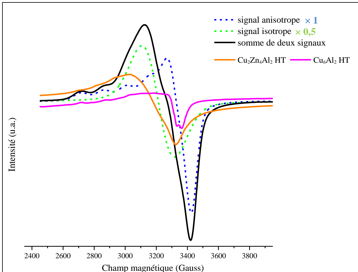
Figure II-8 : Signaux RPE, isotrope et anisotrope, calculés par simulation avec la représentation de leur sommation
