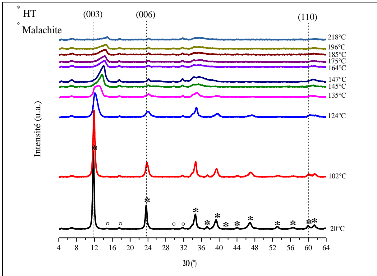
Figure II-12 : Suivi par DRX de la calcination sous air de \text{Cu}_4\text{Zn}_2\text{Al}_2 HT entre 20^\circ et 218^\circ\text{C}
