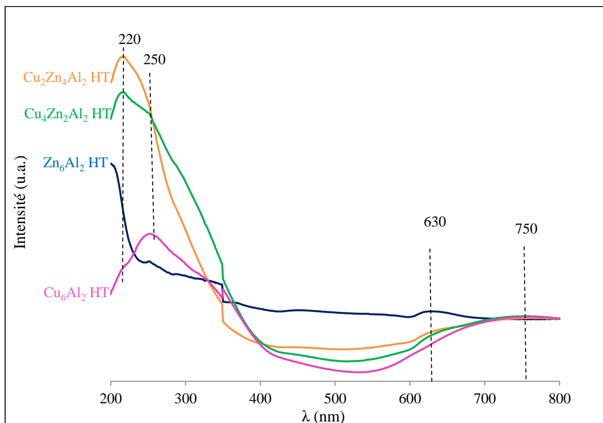
Figure II-6 : Spectres UV-Visible des solides \text{Cu}_x\text{Zn}_{6-x}\text{Al}_2 HT dans la zone spectrale 200-800 nm
