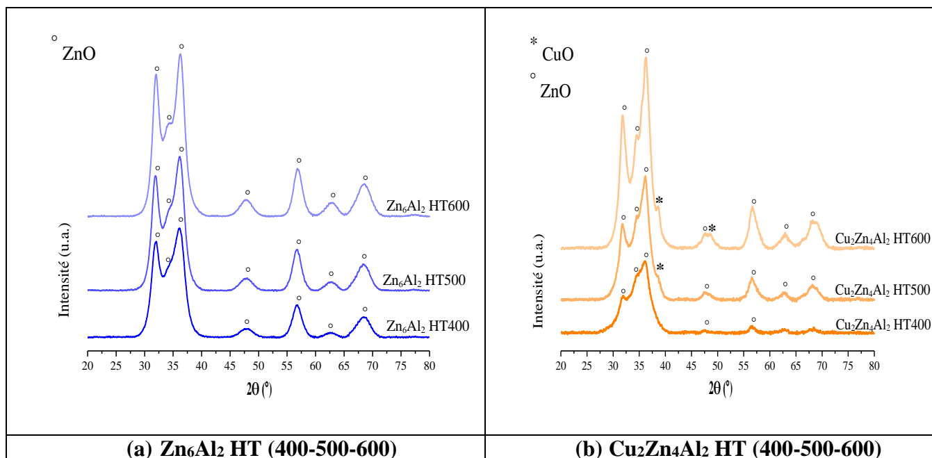
Figure II-18: Diffractogrammes RX des solides \text{Cu}_x\text{Zn}_{6-x}\text{Al}_2 HT calcinés à 400^\circ , 500^\circ et 600^\circ\text{C} (*48-1548: CuO, °36-1451: ZnO) [(a) \text{Zn}_6\text{Al}_2 HT(400-500-600), (b) \text{Cu}_2\text{Zn}_4\text{Al}_2 HT(400-500-600), (c) \text{Cu}_4\text{Zn}_2\text{Al}_2 HT(400-500-600) et (d) \text{Cu}_6\text{Al}_2 HT(400-500-600)]
