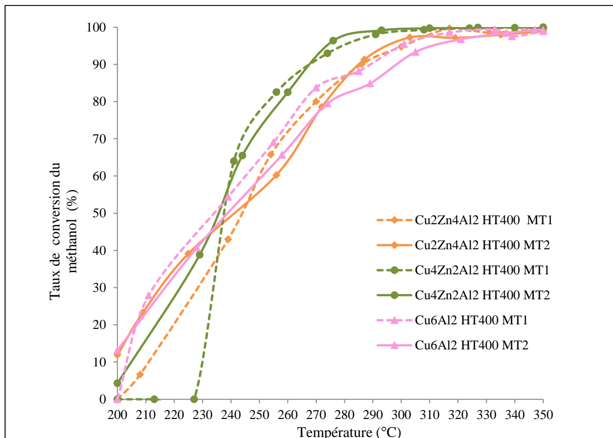
Figure II-38: Évolution de taux de conversion du méthanol en fonction de la température en présence des solides \text{Cu}_x\text{Zn}_{6-x}\text{Al}_2 HT calcinés à 400^\circ\text{C} pendant la montée 2 (MT2)
