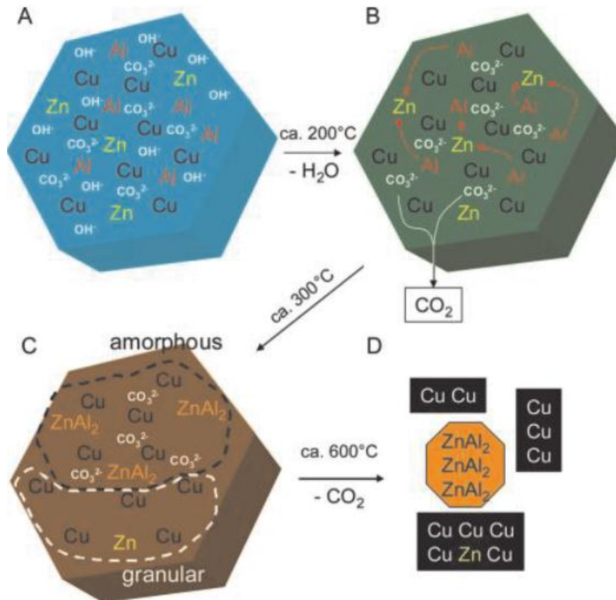
Figure II-16: Modèle de décomposition thermique d'un hydrotalcite à base de Cu, Zn et Al.
