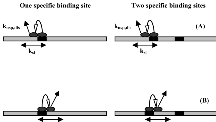
Figure 90 : Représentation schématique de la méthode de base pour mesurer les taux de glissement. (Rau et Sidorova 2010).
