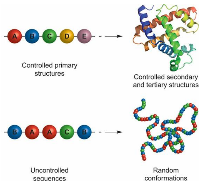
Figure 1. Importance de la régularité des séquences en synthèse de polymères. L'architecture principale bien définie des biopolymères conduit à la formation de structures secondaires et tertiaires ( haut ), à l'inverse des structures peu contrôlées des polymères synthétiques usuels ( bas ). Réimprimé avec la permission de Macmillan Publishers Ltd: Nature Chemistry,[2] copyright 2010.
