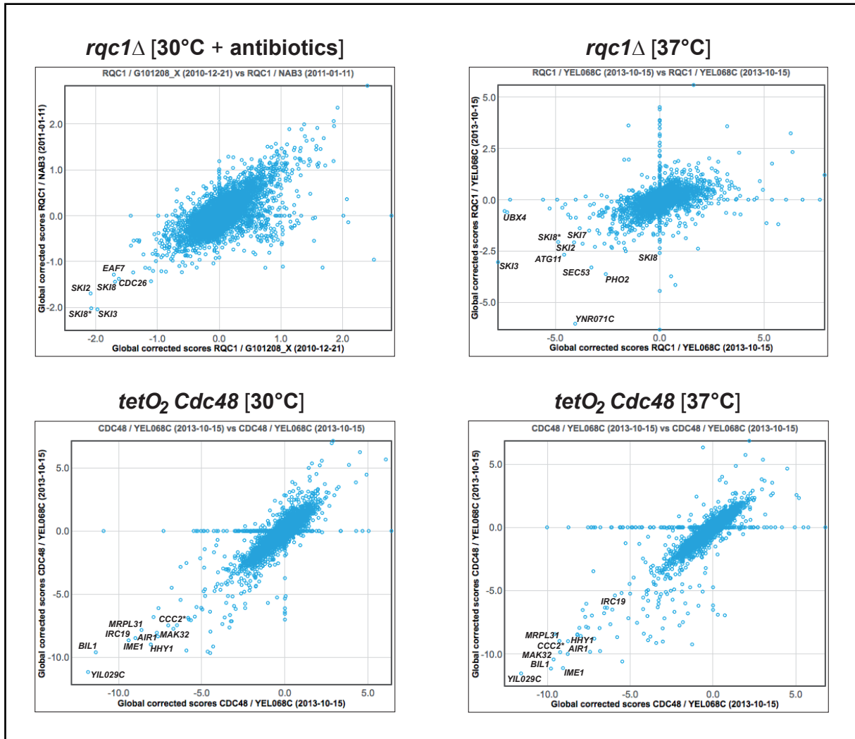
Figure 42. Cribles GIM des souches rqc1 Δ et tetO 2 Cdc48 à 30°C et 37°C Cribles GIM réalisés selon (Decourty et al., 2008). Les gènes correspondant aux mutants présentant les plus fortes interactions fonctionnelles sont indiqués.
