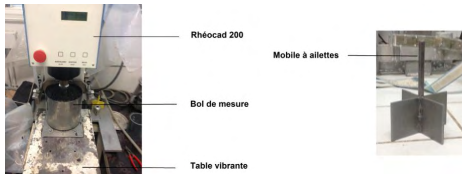
Figure III – 2: Dispositif de mesure des propriétés rhéologiques
