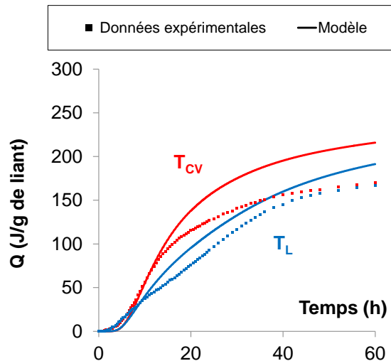
Figure IV – 15 : Comparaison de l'évolution de la chaleur d'hydratation mesurée et celle du modèle pour les mortiers bas pH
