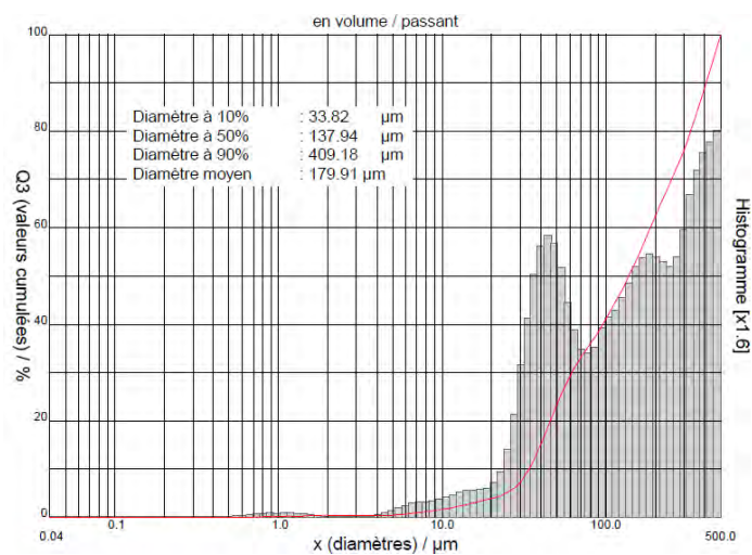
Figure II – 6 : Granulométrie laser du liant T CV
