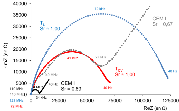
Figure V – 35 : Spectres d'impédance mesurés sur les bétons bas pH et comparés avec les résultats expérimentaux d'un béton à base de CEM I de [Mercado, 2012]
