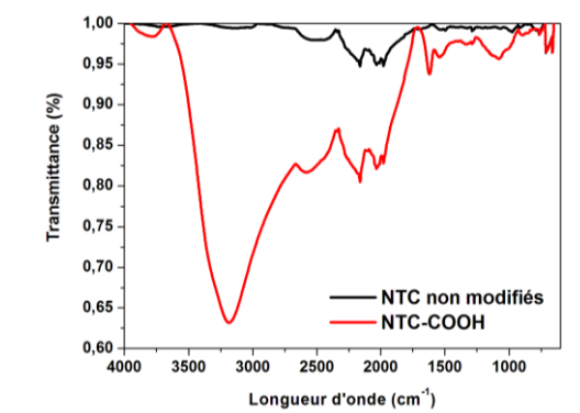
Figure XXXIV : Spectre infrarouge à transformée de Fourier des NTC avant oxydation et après oxydation, mesuré avec un ATR utilisant un cristal de Diamant sur 256 scans.
