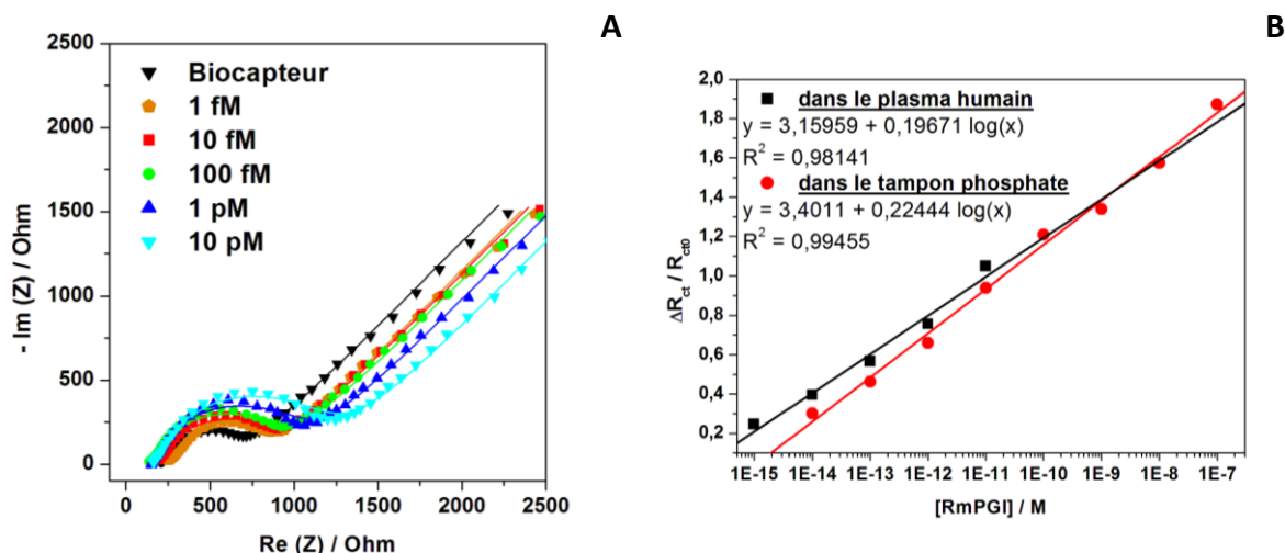
Figure XXXII : (A) Diagrammes de Nyquist obtenus après chacune des cinq concentrations de RmPGI testées (de 1 fM à 10 pM). Les graphes ont été réalisés dans [Fe(CN)_6]^{3-/4-} dans PBS, pH 7,4, dans une gamme de fréquence allant de 100 kHz à 0,1 Hz. Les symboles sont les données expérimentales tandis que les traits pleins correspondent aux courbes de fit utilisant le circuit électrique de type Randles équivalent. (B) Droites d'étalonnage établies à partir des résultats de d'impédancemétrie avec en noir les mesures dans le plasma humain et en rouge les mesures dans le tampon phosphate.
