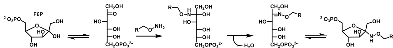
Schéma XXIX : Mécanisme du greffage du biorécepteur.
