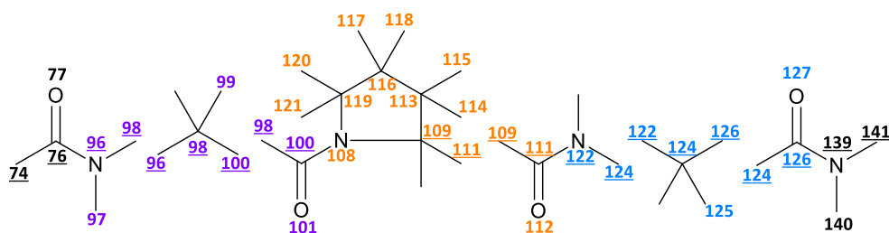
Schéma VIII : Représentation schématique du segment Asp7-Gln9 fragmenté selon SIBFA avec les coordonnées de certains atomes dupliqués.
