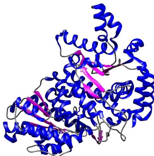
Figure VI : Structure tridimensionnelle d'un monomère de l'AMF/PGI humaine (PDB : 1IAT). 39
