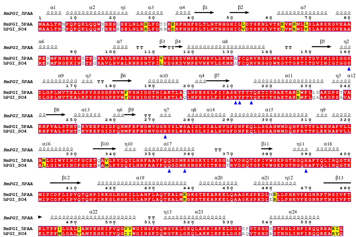
Figure XXVI : Alignement de séquence entre l'AMF/PGI humaine et celle de lapin. Les acides aminés du site actif sont pointés par les triangles bleus. Les acides aminés identiques sont surlignés en rouge, les acides aminés fortement similaires sont en jaune et les faiblement similaires ne sont pas surlignés.
