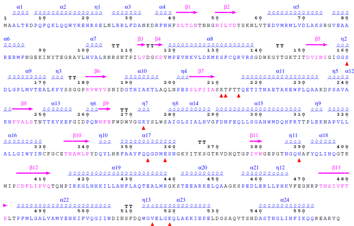
Figure VII : Séquence primaire d'un monomère de l'AMF/PGI humaine (PDB : 1IAT) 39 et structures secondaires associées (α : hélices alphas, η : hélices 3_{10} , β : feuillets bêtas et T : coudes). Les triangles rouges pointent les acides aminés du site actif.
