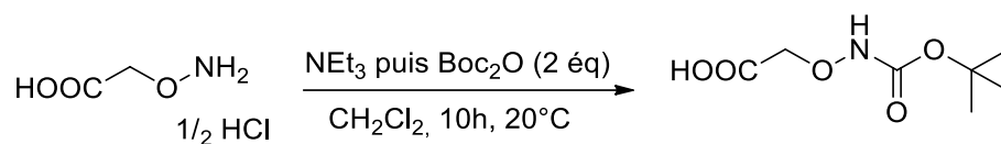
Schéma XXIII : Synthèse de l'acide (Boc)aminoxyéthanoïque.
