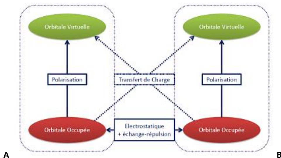
Schéma XIII : Décomposition de l'énergie d'interaction par l'approche RVS.
