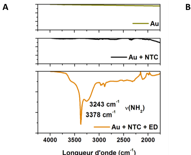
Spectre infrarouge à transformée de Fourier avec un ATR utilisant un cristal de Diamant de la surface après le greffage de l'éthylène diamine..
