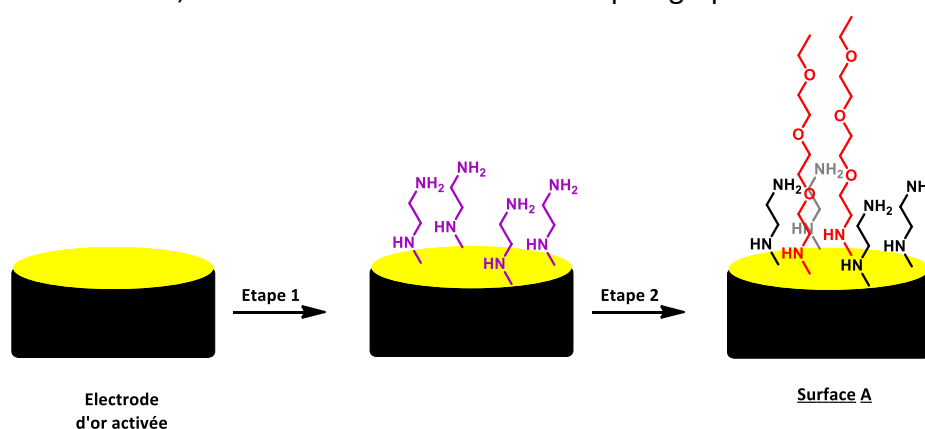
Schéma XXVI : Schéma de la fonctionnalisation de la surface d'or.
