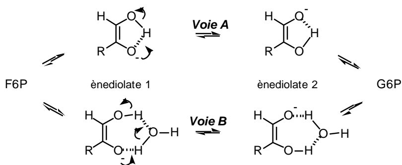
Schéma VI : Proposition de mécanismes de transfert du proton entre les oxygènes des carbones C1 et C2 des substrats F6P et G6P dans la réaction d'isomérisation catalysée par les PGI.
