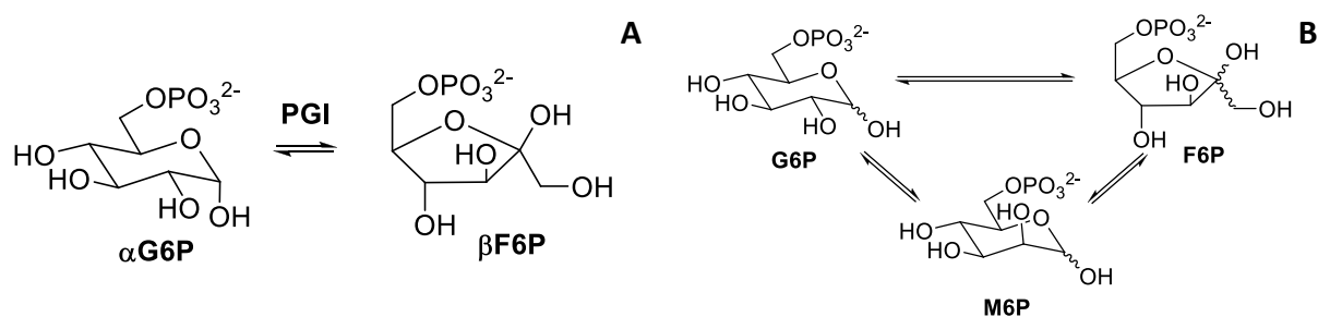
Schéma IV : (A) Réaction catalysée par la PGI. (B) Autres réactions catalysées par la PGI de muscle de lapin.
