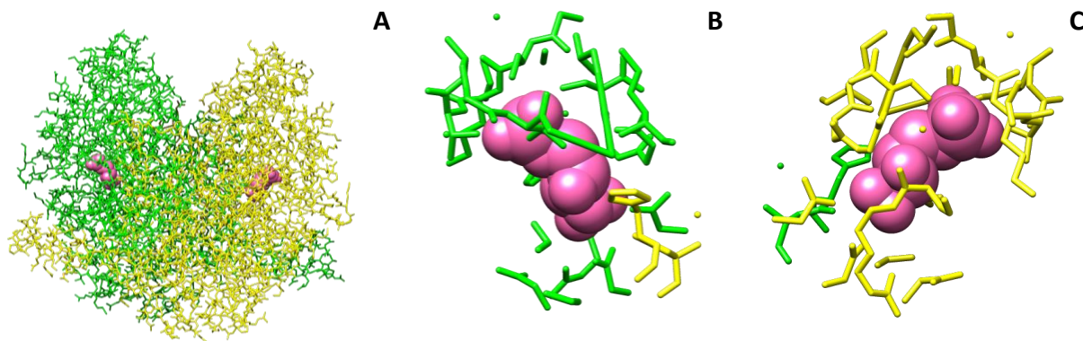
Figure IX : Visualisation par Chimera des deux monomères A (en vert) et B (en jaune) de l'AMF/PGI humaine (PDB : 1IRI). 38 (A) Dimère entier. (B) et (C) 4-phosphate-D-érythrose en rose et les acides aminés au voisinage (jusqu'à une distance de 5 Å) au niveau du monomère A et du monomère B respectivement.
