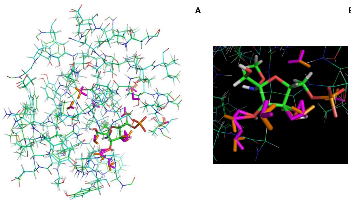
Figure XXV : Présence de clashes stériques lors de l'insertion du mime de biorécepteur dans l'AMF réduite en présence des onze molécules d'eau. (A) Vue 'ensemble et (B) zoom sur le mime de biorécepteur.
