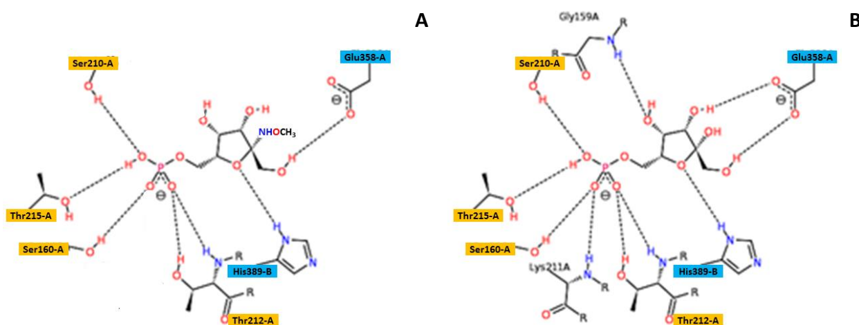
Schéma XVIII : (A) Interactions intermoléculaires déterminées dans le complexe hAMF/PGI—F6P-nome. (B) Interactions intermoléculaires déterminées dans le complexe mAMF/PGI—F6P (PDB 2CX5).
