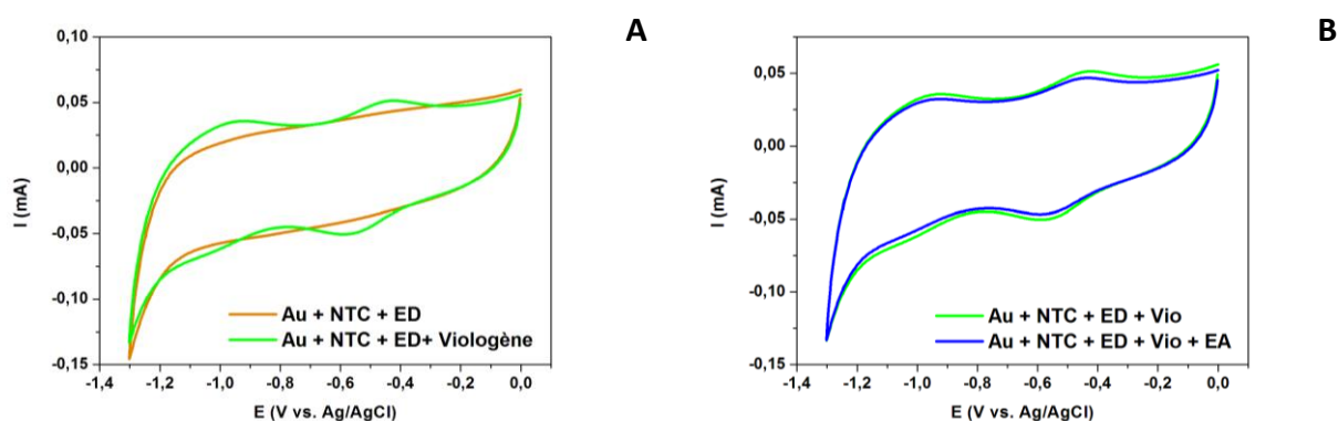
Figure XXXIX : Voltampérométries cycliques du greffage du viologène (A) et du blocage de la surface par l'éthanolamine (B). Les analyses ont lieu dans du PBS durant 5 cycles à 100 mV/s.
