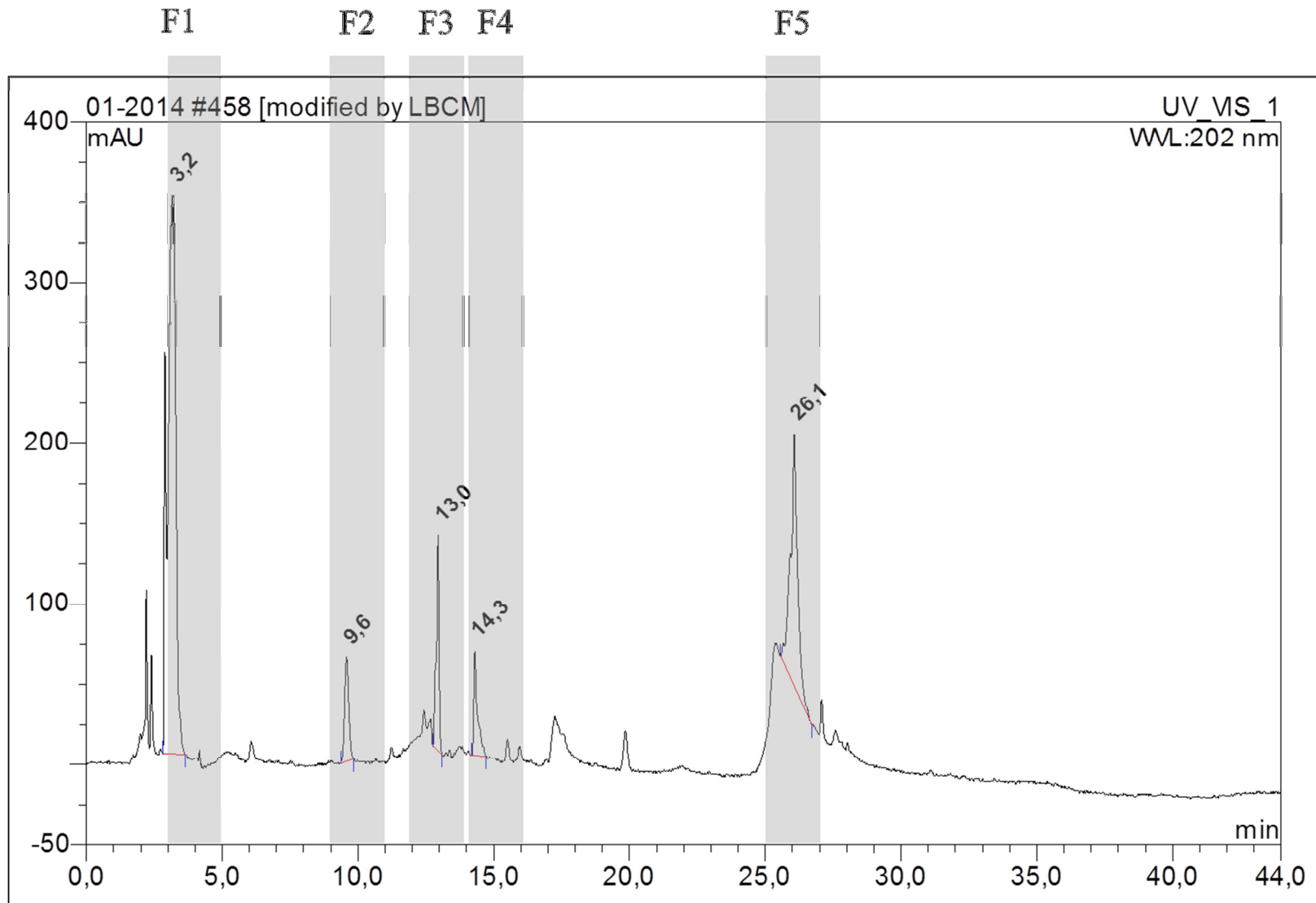
Figure 46 : Chromatogramme de l'EMSR de 2013. Les zones grisées représentent les 5 fractions différentes sélectionnées par chromatographie liquide analytique.
