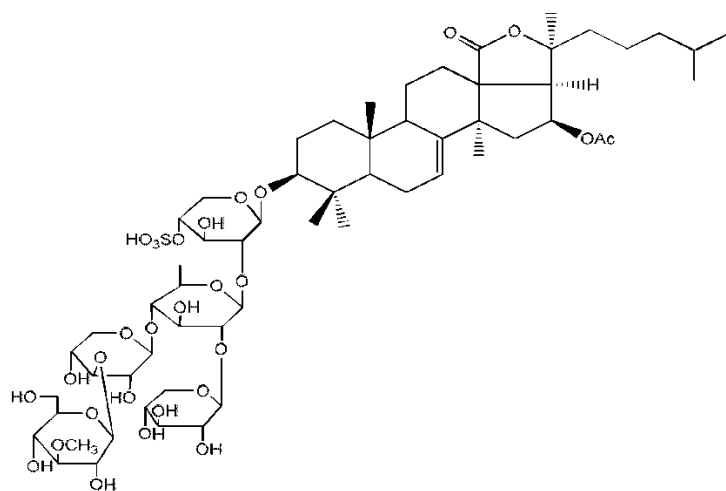
Figure 69: Représentation structurale de Frondoside A 6
