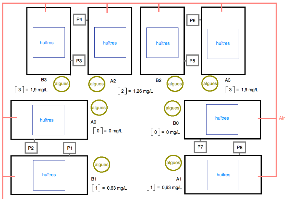
Figure 30 : Schéma des installations des conditions d'expérimentation d'évaluation de l'EMSR en toxicologie algue sur le modèle C. virginica (P : Pompe péristaltique)
