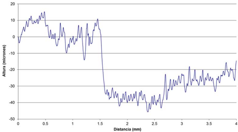
Fig. 2.40. Perfil de rugosidad de las superficies a unir. En la figura se muestra uno de los perfiles radiales obtenidos para una de las superficies a unir de los tubos.
