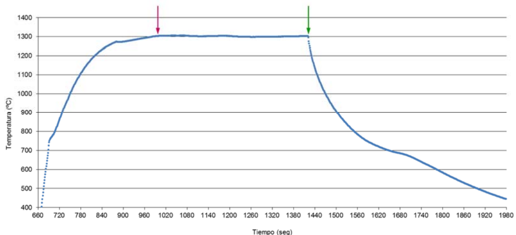
Fig. 3.2. Ciclo térmico al que fue sometida la juntura. Con una flecha roja se indica cuando esta alcanza T_P , de 1300°C. La flecha verde indica el momento en que se apagó el horno, luego de permanecer 7 min a T_P .
