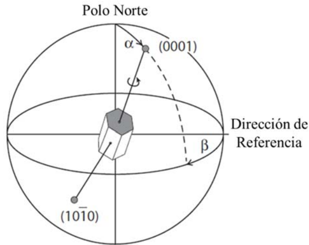
Fig. 2.18. Orientación del plano (0001) en un cristal hexagonal. La posición del polo (0001) en la esfera unidad con respecto a un marco de referencia externa se encuentra descrita por los dos ángulos \alpha y \beta . Sin embargo, el cristal todavía puede girar alrededor del polo (0001). Para una única definición de la orientación del cristal más información es necesaria, como por ejemplo la posición del polo (10-10).
