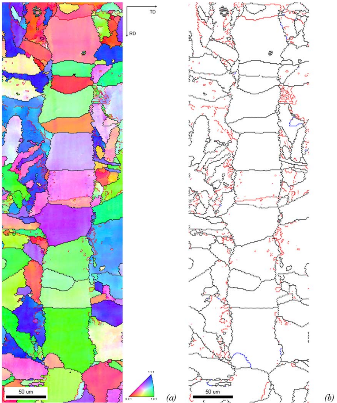
Fig. 4.18. EBSD en la juntura. (a) IPF de la ND en la juntura. En trazo negro se indican los HAGB, mientras que en trazo rojo se indican los LAGB. Se destaca como prevalecen los primeros; (b) Detalle de (a), donde solo se indican los bordes de grano, discriminando los HAGB entre aquellos que corresponden a una determinada CSL - en este caso particular \Sigma 3 , en azul - de aquellos que separan granos con una orientación cristalográfica aleatoria entre sí.
