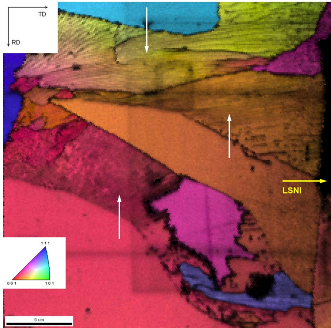
Fig. 6.12. Detalle de la IPF de la Fig. 6.11, al que se le superpuso el mapa de IQ. Además de la ferrita y el LSNI, se pueden distinguir las lamelas de cementita pertenecientes a las colonias perlíticas (flechas blancas).
