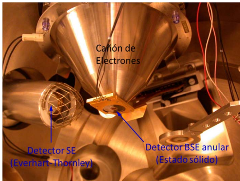
Fig. 2.4. Detectores de SE y BSE en un SEM. Disposición típica respecto del cañón de electrones, dentro de la cámara de vacío del equipo.
