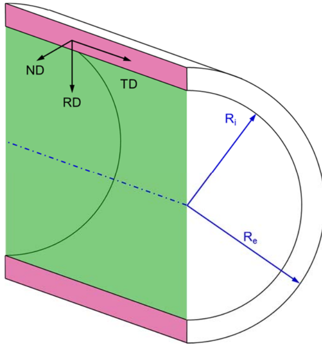
Fig. 4.3. Definición de los ejes coordenados ND, RD y TD.
