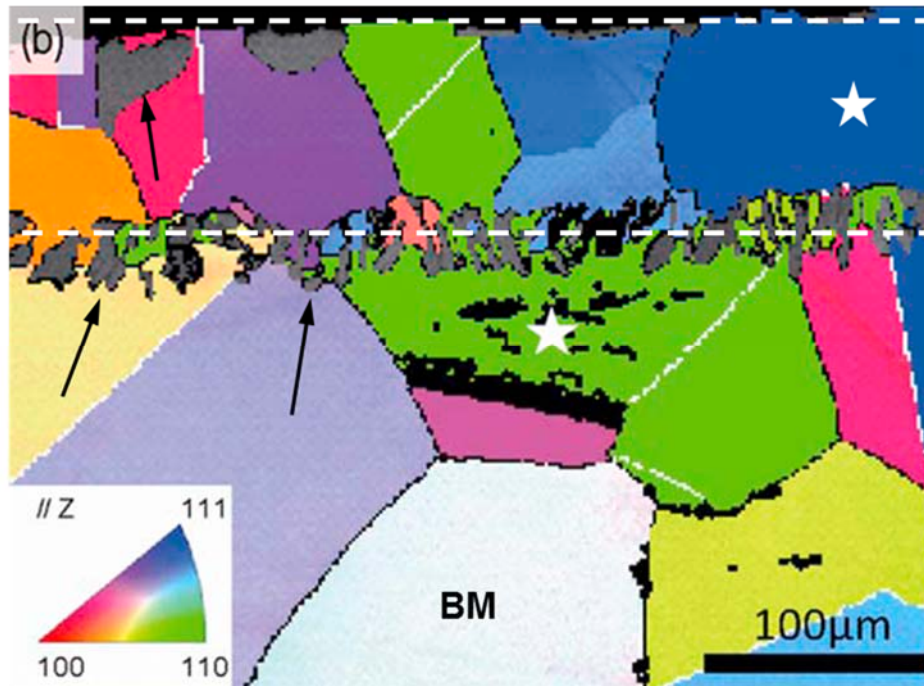
Fig. 4.43. IPF de la ND de la unión TLPB de la fase \alpha -Ni (Grupo espacial: 225/Fm-3m ) realizada por Ruiz-Vargas et al [Ruiz-Vargas 2013]. Los granos marcados con una estrella solidificaron isotérmicamente (delimitados por líneas de trazo) en forma epitaxial respecto de granos del BM. Además, con flechas, se indican los precipitados de la fase intermetálica Ni_3B (Grupo espacial: 62/Pnma ), que no fueron indexados.
