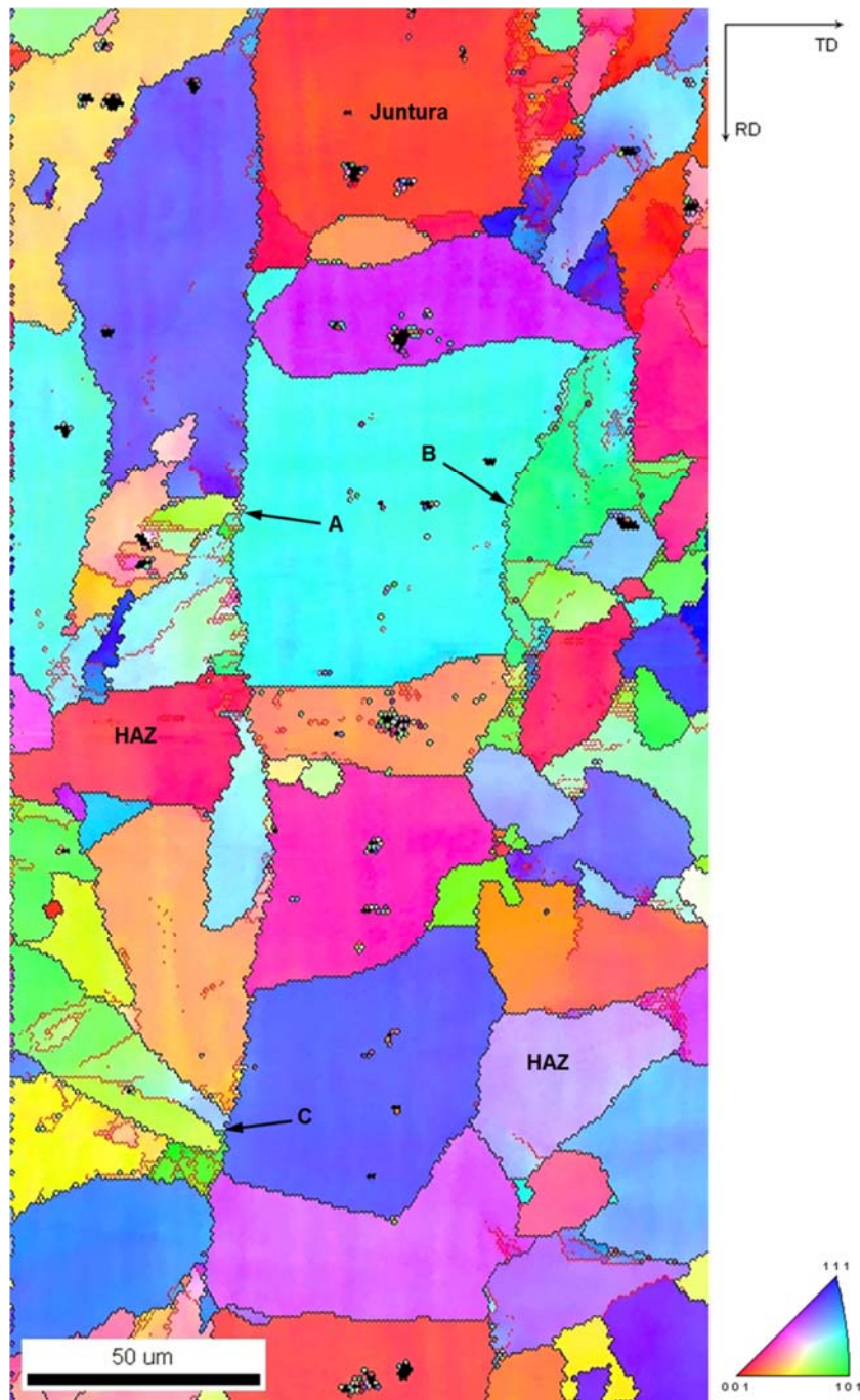
Fig. 4.16. IPF de la ND en la junta. Las flechas A, B y C indican las posiciones que fueron posteriormente observadas mediante SEM en la Fig. 4.17. En trazo negro se indican los HAGB ( \theta > 15^\circ ), mientras que en trazo rojo se indican los LAGB ( \theta \leq 15^\circ ).
