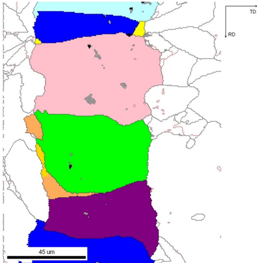
Fig. 4.20. EBSD en la junta, próxima a la superficie interna. En color, los granos pertenecientes a la junta. No se aprecian diferencias sustanciales respecto a otras posiciones en la junta, con una solidificación isotérmica prácticamente completa y una microestructura preponderante del Tipo A.
