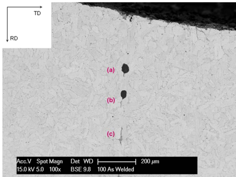
Fig. 4.21. Inclusiones en la Zona Exterior. Se destacan los detalles (a), (b) y (c) pertenecientes a la Fig. 4.22 (Nital 2%).
