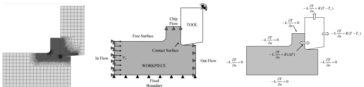
Figure II-22 : Maillage initial et conditions aux limites en déplacements et en températures du modèle numérique [Bro09].
