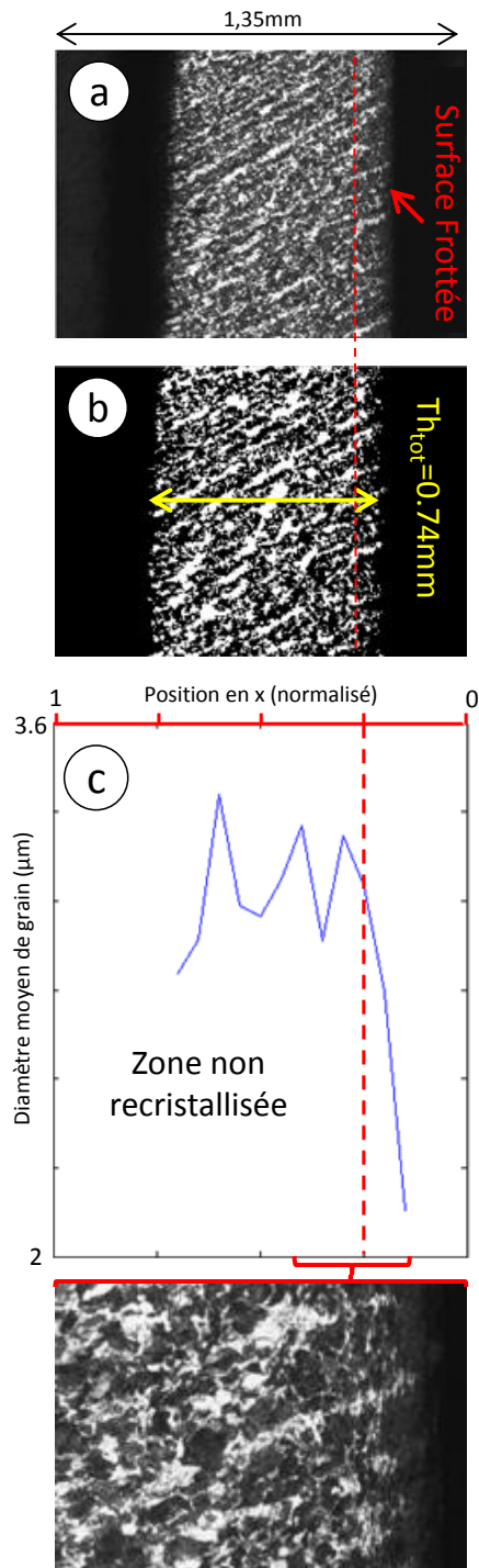
Figure III-13 : Analyse micrographique pour une vitesse de coupe de 40 \text{ m} \cdot \text{min}^{-1} et une profondeur de coupe de 0.3 \text{ mm} .
