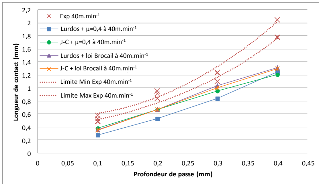
Figure IV-20 : Comparaison des résultats expérimentaux et numériques en termes de longueurs de contact pour une vitesse de coupe égale à 40\text{m}\cdot\text{min}^{-1} .
