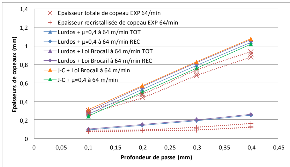
Figure IV-26 : Comparaison des résultats expérimentaux et numériques en termes d'épaisseurs de copeau pour une vitesse de coupe égale à 64m.min -1 .
