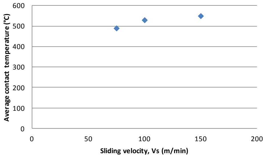
Figure I-16 : Evolution de la température de contact en fonction de la vitesse de glissement [Rec09].
