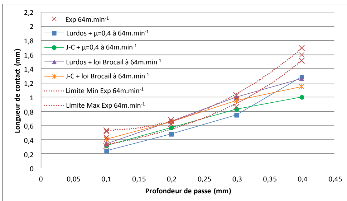
Figure IV-21 : Comparaison des résultats expérimentaux et numériques en termes de longueurs de contact pour une vitesse de coupe égale à 64\text{m}\cdot\text{min}^{-1} .
