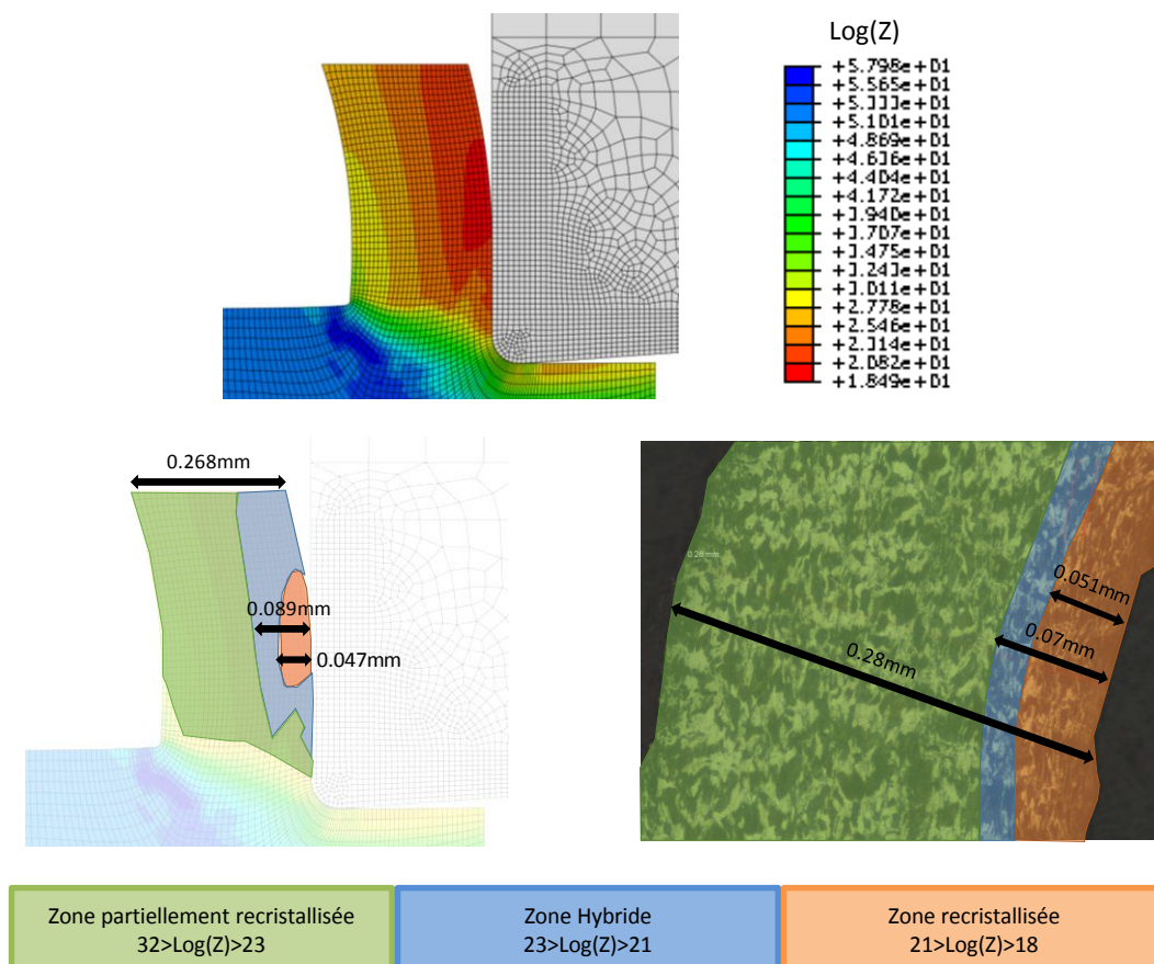
Figure III-17 : Résultats expérimentaux et numériques pour une profondeur de coupe égale à 0,1mm et une vitesse de coupe de 64\text{m}\cdot\text{min}^{-1}
