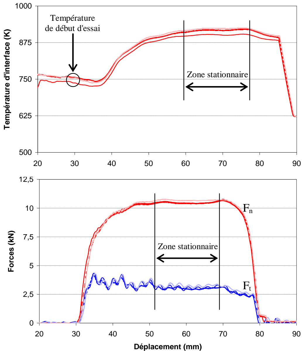
Figure II-4 : Résultats expérimentaux pour la configuration 6 ( 80\mu\text{m} , 24\text{m}\cdot\text{min}^{-1} et 477^\circ\text{C} ).
