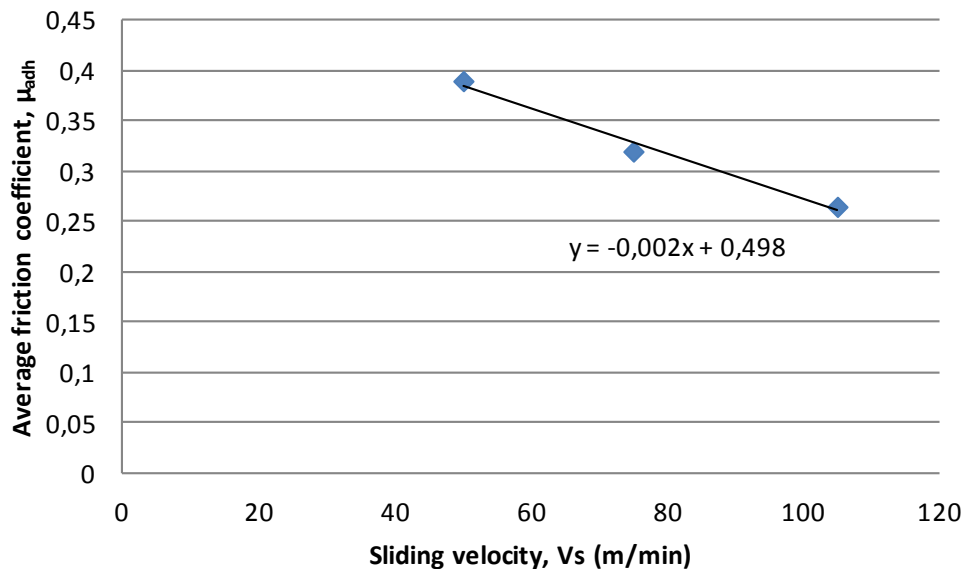
Figure I-17 : Evolution du coefficient de frottement d'adhésion en fonction de la vitesse de glissement [Rec09].
