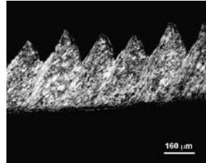
Figure I-3 : Copeau festonné obtenu lors de l'usinage d'un acier inoxydable 316L avec un outil WC-Co non revêtu (vitesse de coupe = 100\text{m}\cdot\text{min}^{-1} , profondeur de passe = 0,2\text{mm} ) [Out 06].
