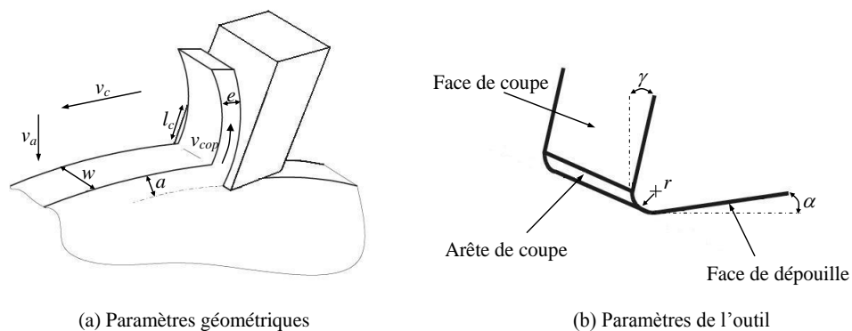
Figure I-1 : Représentation de la coupe orthogonale.
