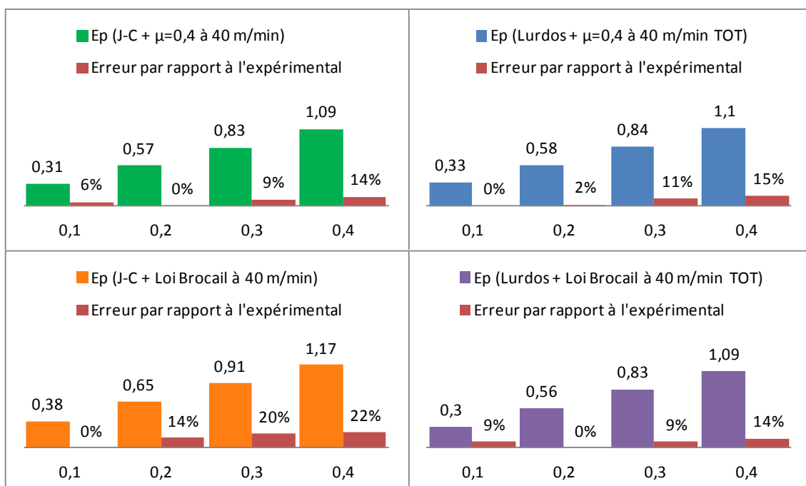
Figure IV-27 : Erreurs commises par rapport aux résultats expérimentaux pour chaque profondeur de passe en termes d'épaisseurs de copeau pour une vitesse de 40m.min -1
