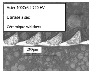
Figure I-4 : Copeau en dent de scie (vitesse de coupe = 110\text{m}\cdot\text{min}^{-1} , profondeur de passe = 0,1\text{mm} ) [Pou 02].
