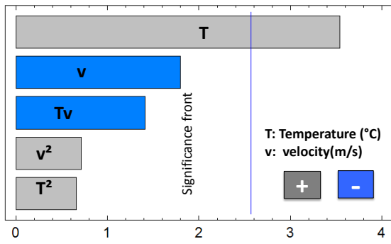
Figure VII.11. Effet de la température et de la vitesse de l'air sur l'accessibilité initiale pour DIC5
