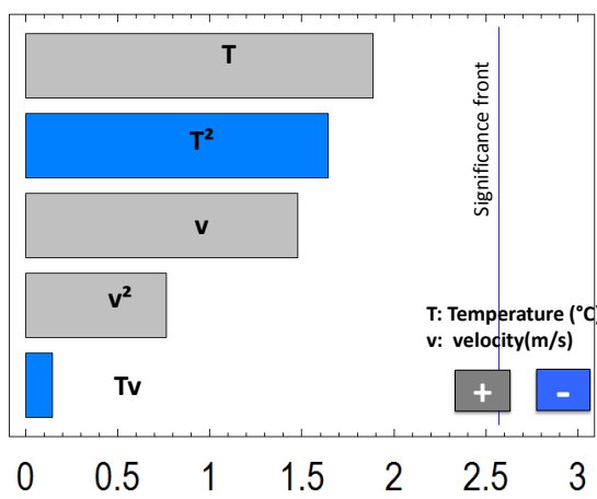
Figure VII.41.Effet de la température et de la vitesse de l'air sur l'accessibilité initial pour le traitement DIC5
