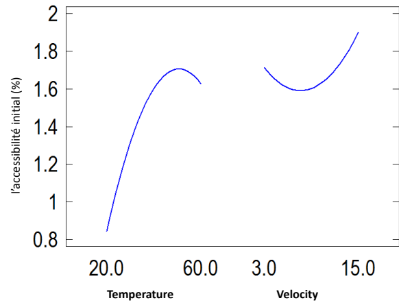
Figure VII.40.Effet de la température et de la vitesse de l'air sur l'accessibilité initial pour le traitement DIC4
