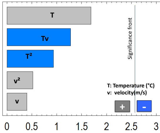
Figure VII.40.Effet de la température et de la vitesse de l'air sur l'accessibilité initial pour le traitement DIC4
