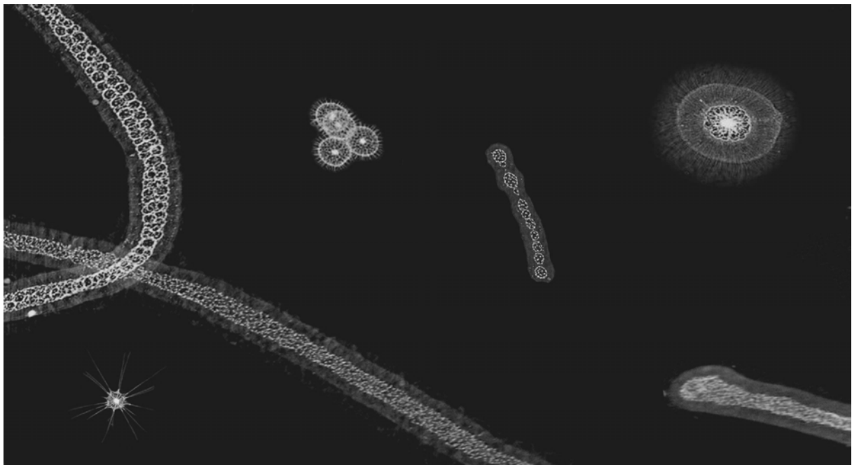
Figure 23 | Illustration de différents Rhizaria observés grâce à l' ISIIS ( In Situ Ichthyoplankton Imaging System). Images issues du projet de science participative Plankton Portal ( http://www.planktonportal.org )
