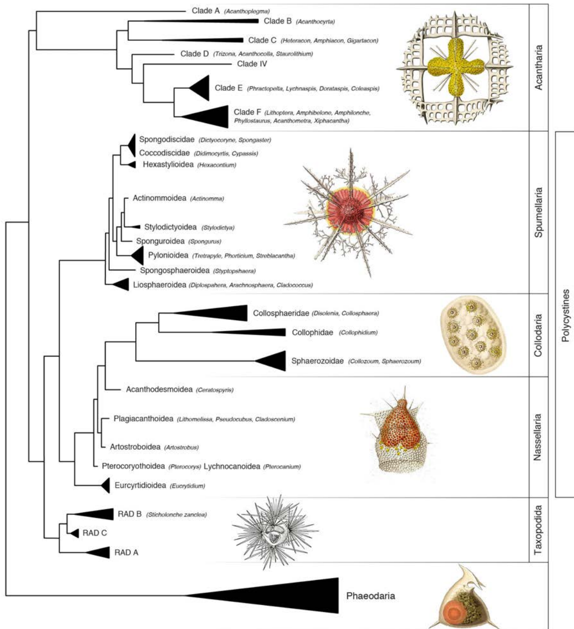
Figure 7 | Arbre schématique des Radiolaires. Les relations entre chaque ordre sont basées sur les connaissances morpho-moléculaires actuelles. La taille des branches correspond au nombre d'espèces vivantes. Les Phaeodaires, appartenant aux Cercozoaires, sont placés comme « outgroup ». Modifié d'après Suzuki et Not (2015).
