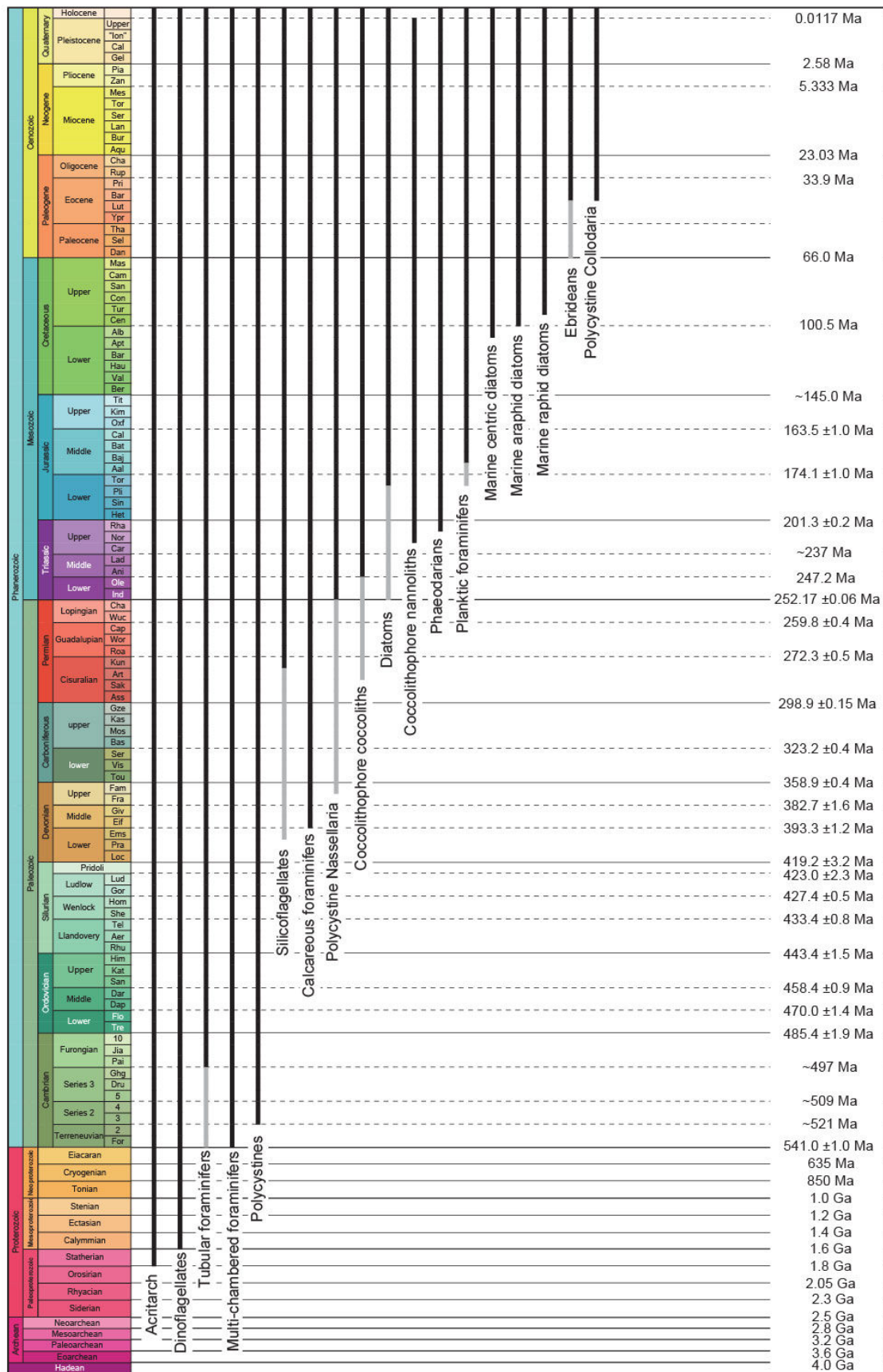
Figure 6 | Histoire géologique des protistes marins fossiles. Lignes noires : étendue des données fossiles pour chaque taxon. Lignes grises : étendue incertaines des données fossiles. Modifié d'après Suzuki et Oba (2015).
