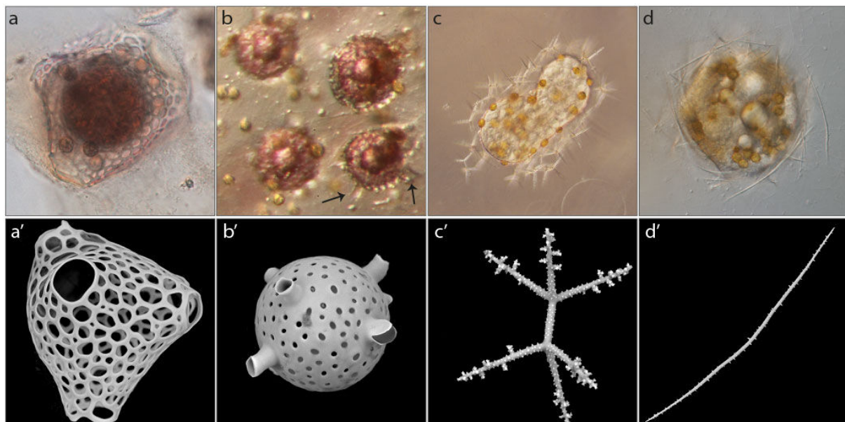
Figure 12 | Illustration des différentes formes de structures en silice observable chez les Collodaires. (a,a') Disolenia zanguebarica et son squelette aux larges pores. (b-b') Siphonosphaera abyssii et son squelette aux longues extensions. (c-c') Sphaerozoum armatum et ses spicules tri-radiés aux multiples extensions micrométriques. (d-d') Rhaphidozoum acuferum et ses spicules simples.
