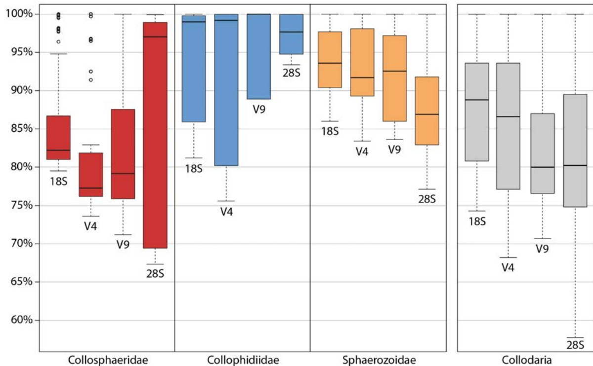
Figure 20 | Divergence interspécifique (pourcentage) pour le gène 18S RNA, ses régions hypervariables V4 et V9, ainsi que le gène 28S. La divergence est présentée au sein de chaque famille (gauche) et pour les Collodaires dans leur ensemble (droite).
