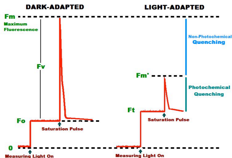
Fig. 6 : Schéma des différentes variables mesurables par fluorescence en fonction de l'état d'adaptation à la lumière de la feuille étudiée.
