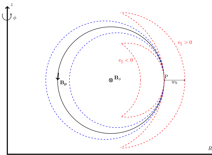
FIGURE 7.1.2. Projection schématique de la trajectoire dans un plan poloïdal des positions gyrocentres de particules passantes (trajectoires en bleu) et piégées (trajectoires en rouge) passant par un même point P . En réalité, leurs trajectoires sont très allongées dans la direction toroïdale \hat{\phi} . Le signe de v_{\parallel} indiqué correspond à des particules chargées positivement, l'axe magnétique vertical étant à gauche sur le schéma [18].
