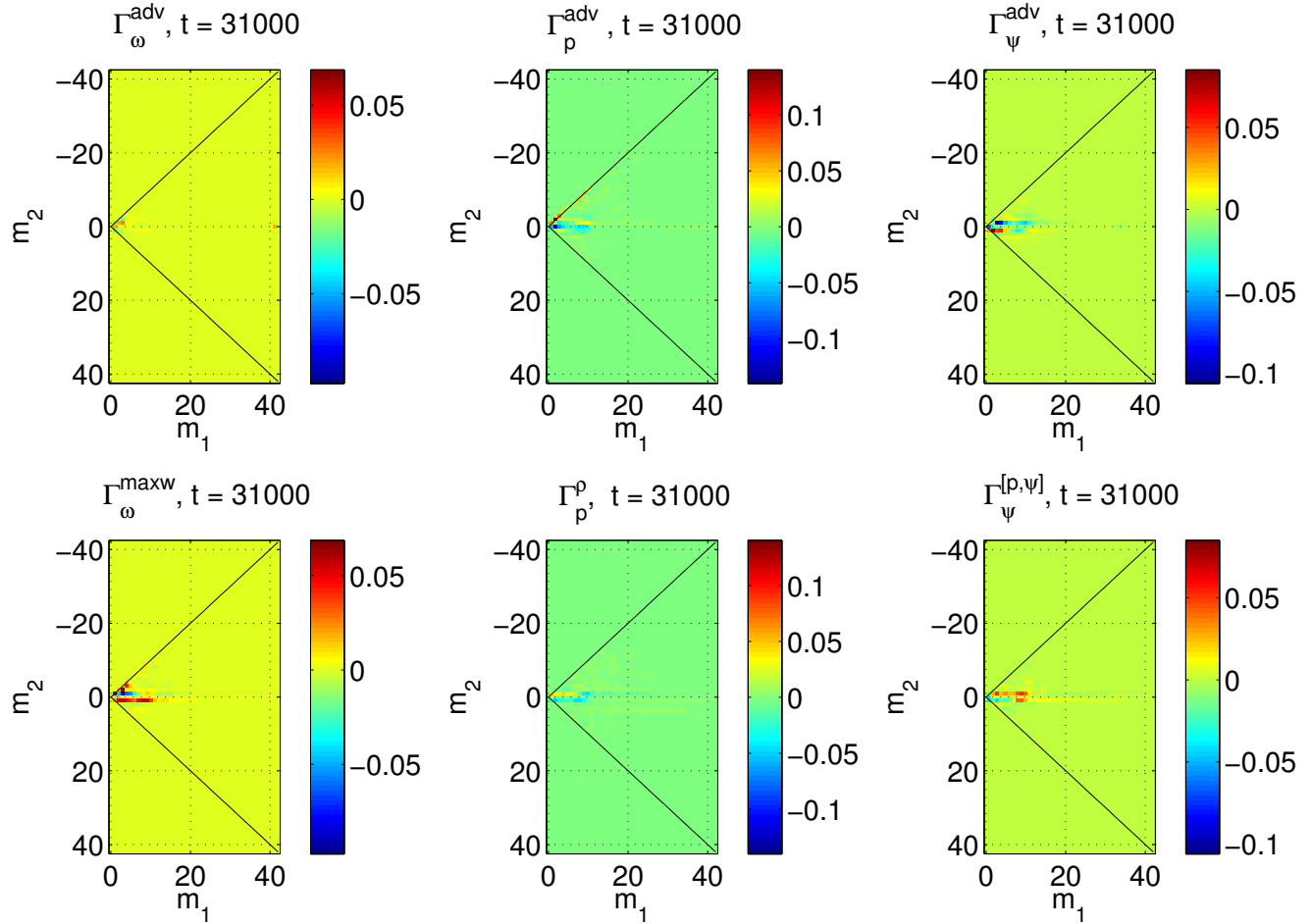
FIGURE 4.4.5. \Delta' = -0.45 . Fonction de transferts des différentes non-linéarités dans la phase non-linéaire à t = 31000\tau_A : [Colonne de gauche] Fonctions de l'équation de vortacité. [Colonne du milieu] Fonctions de l'équation d'évolution des fluctuations de pression. [Colonne de droite] Fonctions de l'équation d'évolution du flux magnétique.
