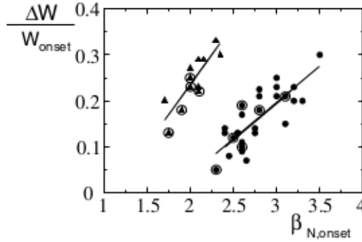
FIGURE 1.2.1. Cette figure est issu de la lettre [52](Autorisation à demander): L’ordonnée est \Delta E_{\text{th}}(w_s)/E_{\text{th}} et “onset” se réfère à la mesure des quantités au moment où le mode NTM m/n=3/2 apparaît. Les données sont issues de décharges produites sur ADEX upgrade. Des résultats similaires ont été obtenus sur JET.
