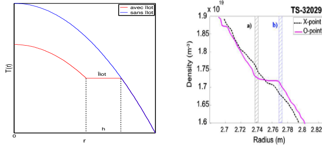
FIGURE 1.1.2. [Gauche] Représentation schématique de l'aplatissement du profil de température électronique d'un îlot. [Droite] Mesure expérimentale de l'aplatissement de la densité dans un îlot par réflectométrie (Graphe issue de [129] avec l'aimable autorisation des auteurs).
