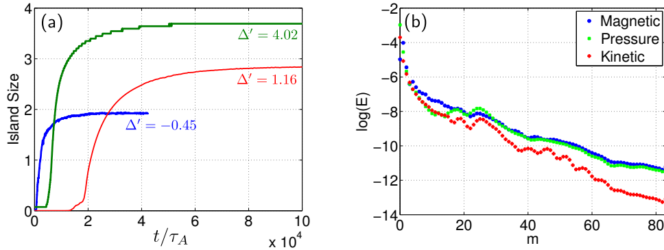
FIGURE 4.3.4. [Gauche] Taille d'îlot en fonction du temps pour différents \Delta' . [Droite] Spectres à t = 40000\tau_A et \Delta' = -0.45 .
