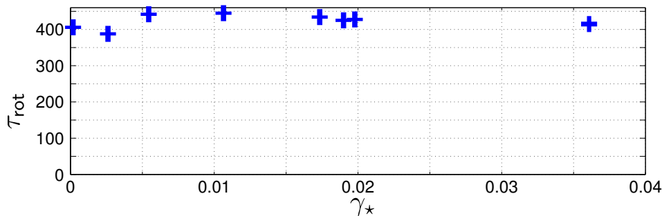
FIGURE 4.3.9. Période de rotation poloidale de l'îlot \tau_{rot} en fonction de \gamma_* .
