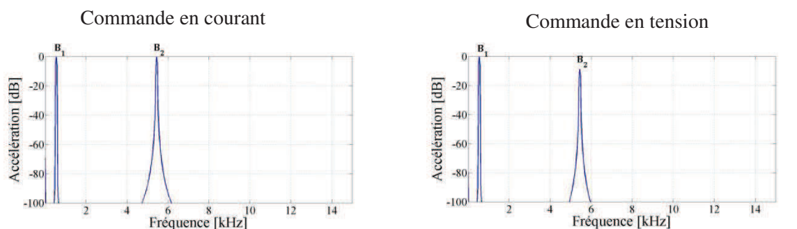
Figure III.57 : Spectres de l'accélération de la référence BPS8 vis-à-vis des défauts liés à k_m(x)
