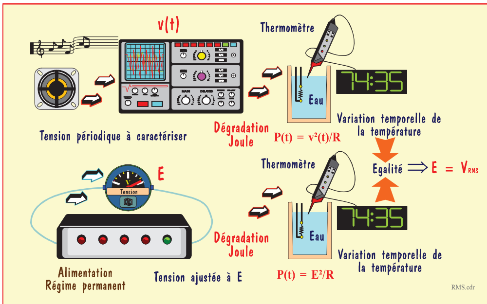
Figure I.1 : Détermination d'une tension RMS par conversion totale du signal en chaleur
