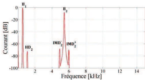
Figure III.36 : Spectre du courant de MORE représentant les distorsions liées à L_c(x)
