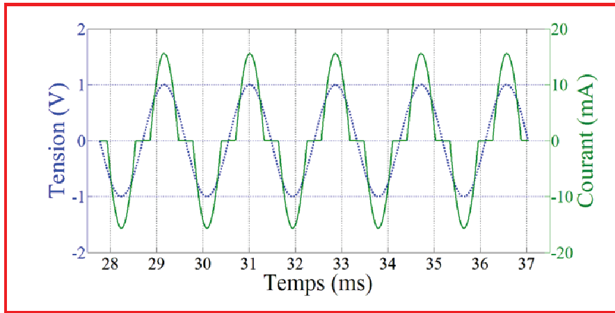
Figure III.72 : Evolutions concomitantes de la tension et du courant sollicitant la charge ZX
