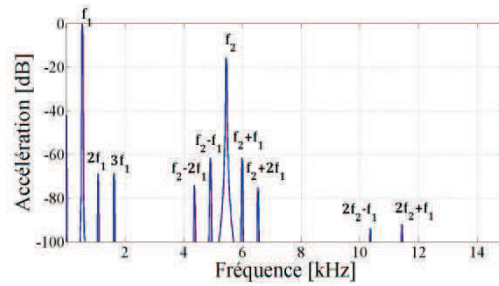
Figure III.29 : Spectre de l'accélération de STRU représentant les distorsions liées à L_c(x)
