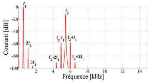
Figure III.28 : Spectre du courant de STRU représentant les distorsions liées à L_c(x)
