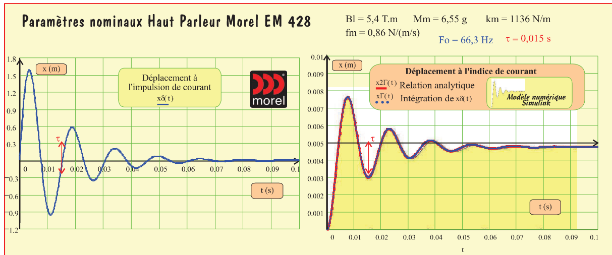
Figure I.6 : Réponses impulsionnelle et indicielle d'un haut parleur médium idéalisé
