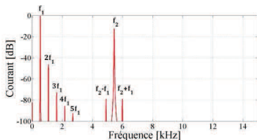
Figure III.8 : Spectre du courant de STRU représentant les distorsions liées à B_1(x)
