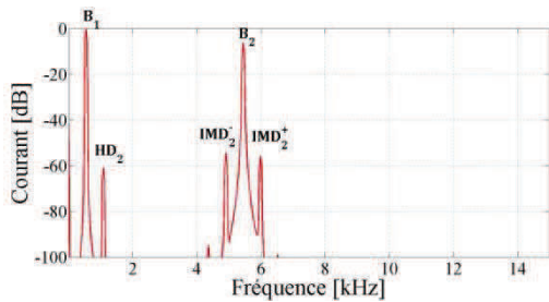
Figure III.32 : Spectre du courant de PION représentant les distorsions liées à L_c(x)
