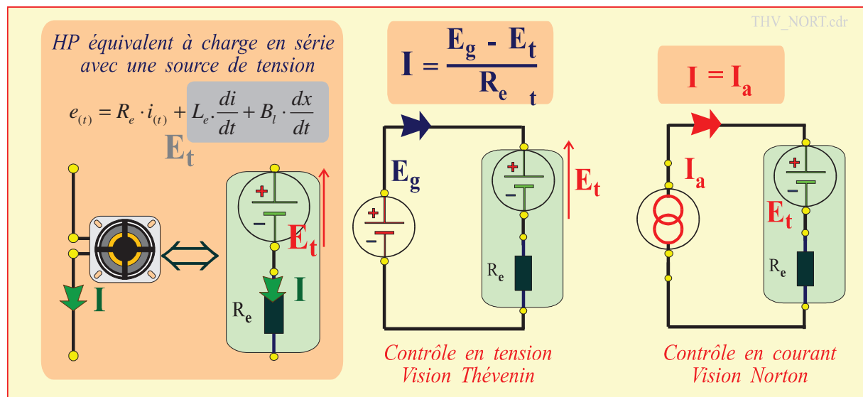
Figure II.10 : Implication relative des paramètres B_l , R_e , L_e sur un comportement d'ensemble
