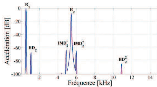
Figure III.37 : Spectre de l'accélération de MORE représentant les distorsions liées à L_c(x)
