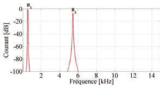
Figure III.22 : Spectre du courant de PION représentant les distorsions liées à k_m(x)
