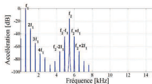
Figure III.9 : Spectre de l'accélération de STRU représentant les distorsions liées à B_1(x)
