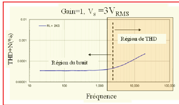
Figure III.66 : Grandeur THD+N (%) mesurée dans la bande passante d'un amplificateur
