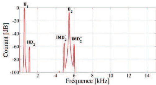
Figure III.30 : Spectre du courant de KLIP représentant les distorsions liées à L_c(x)
