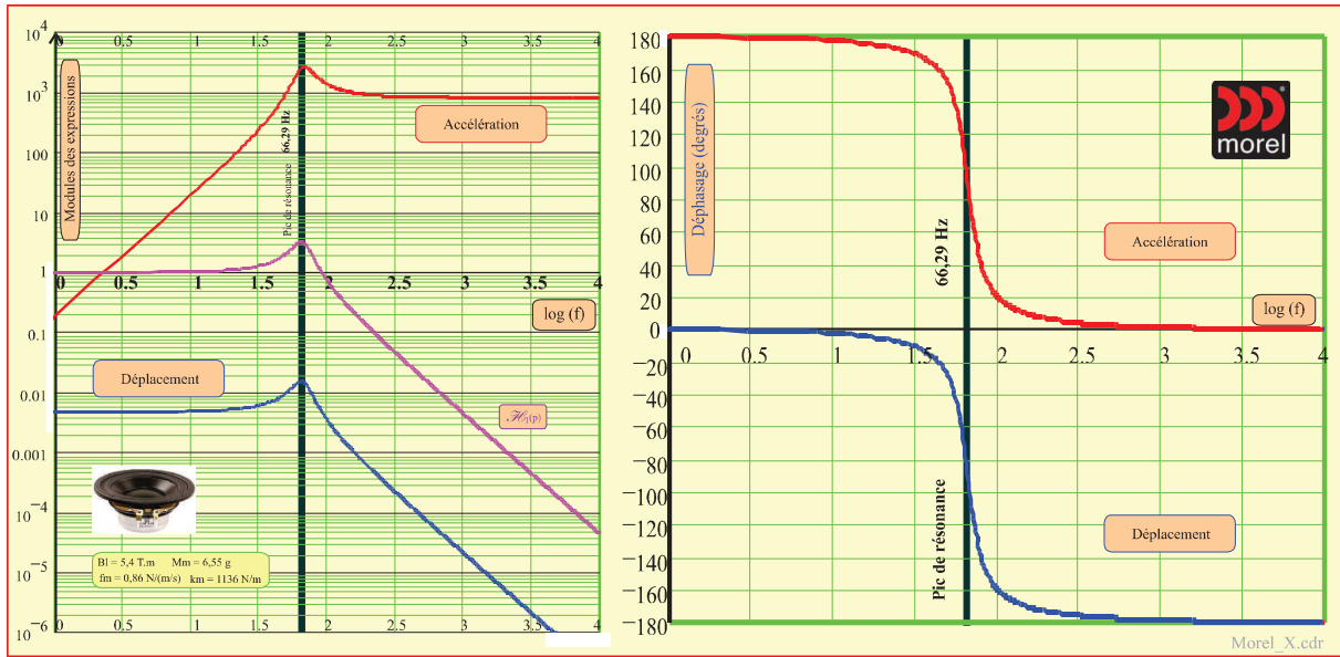
Figure I.8 : Comportement fréquentiel type des fonctions déplacement et accélération
