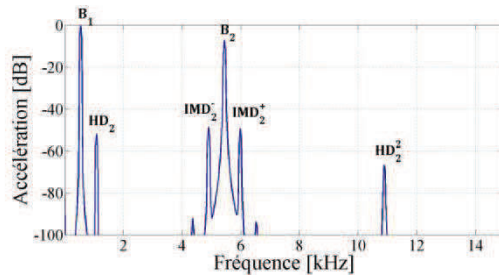
Figure III.31 : Spectre de l'accélération de KLIP représentant les distorsions liées à L_c(x)
