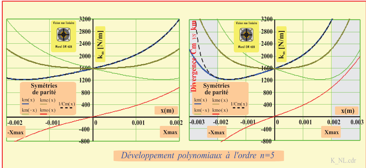
Figure II.16 : Représentation polynomiale de la rigidité k_m et de la compliance C_m
