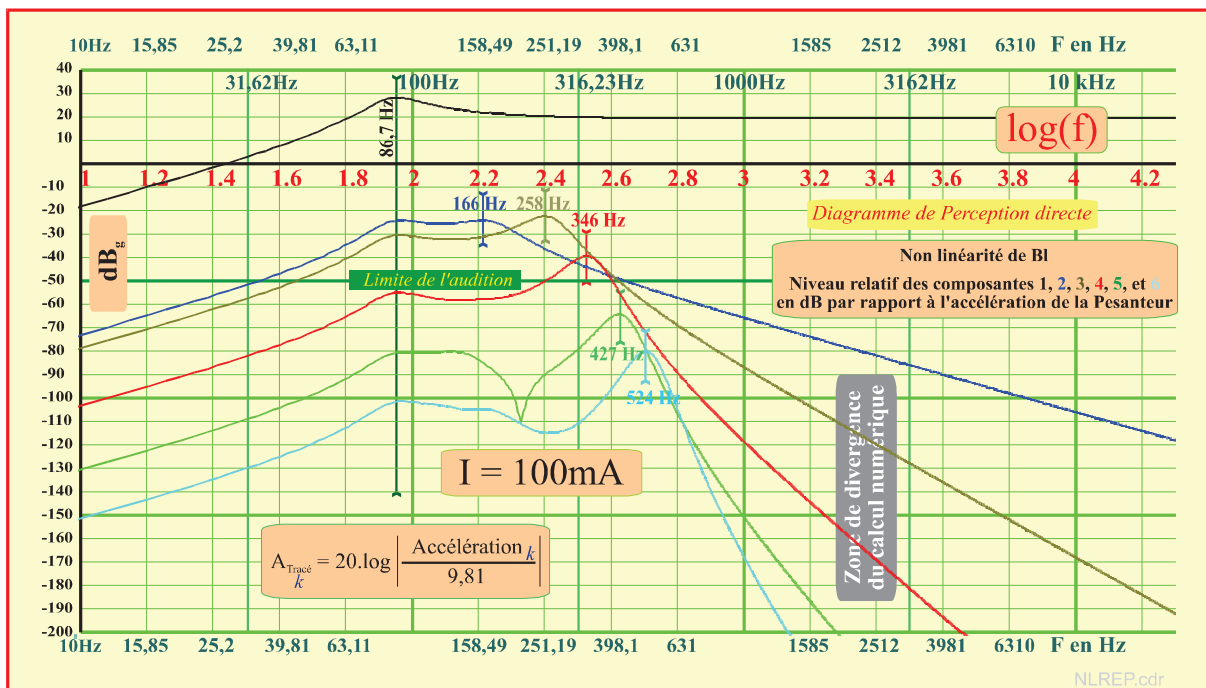
Figure II.23 : Evolutions en dB g et en lecture directe des cinq premières composantes harmoniques affectant le caractère non linéaire du facteur de force (figure II.14 édulcorée)
