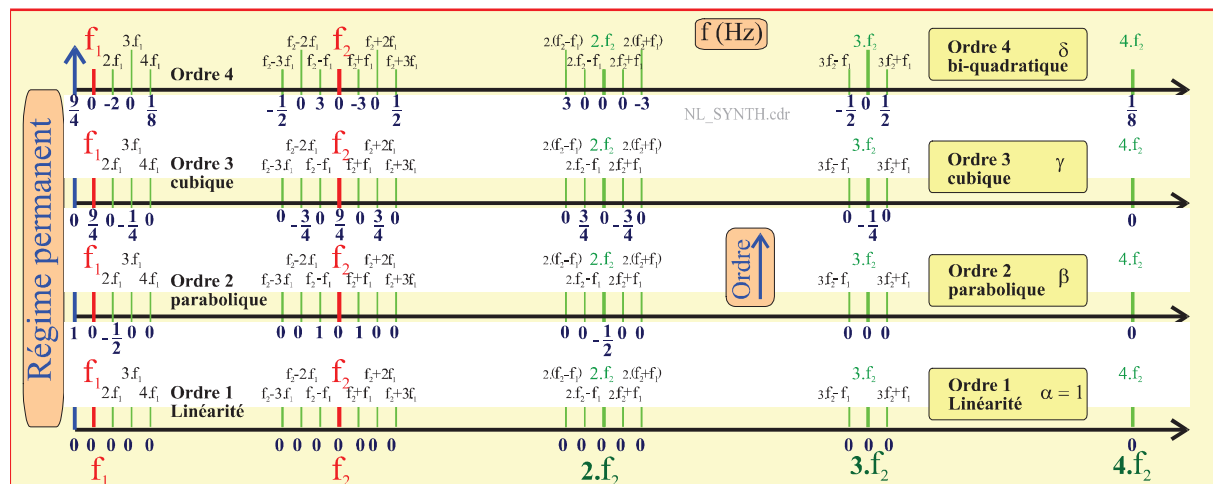
Figure II.7 : Récapitulatif des contributions de chaque ordre de non linéarité
