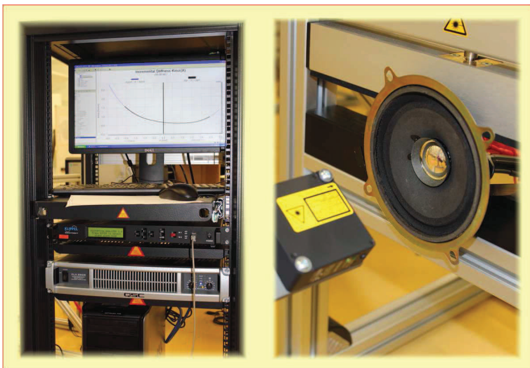
Figure III.2 : Appareil de mesure Klippel® de type laser , référencé ANR1282
