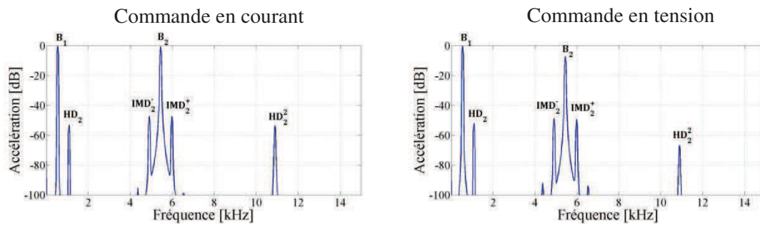
Figure III.58 : Spectres de l'accélération de la référence KLIP représentant les défauts de L_c(x)
