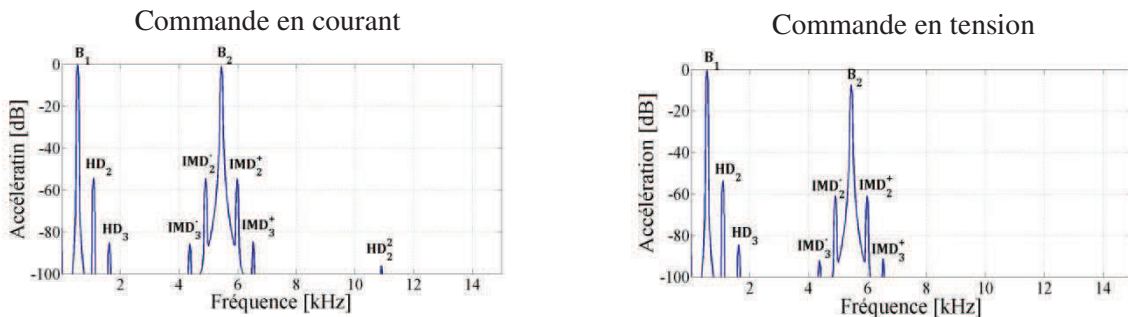
Figure III.50 : Spectre de l'accélération de la référence PION lié aux défauts de B_1(x)
