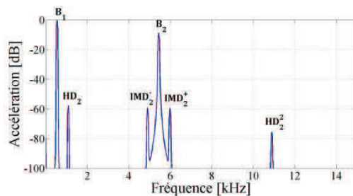
Figure III.33 : Spectre de l'accélération de PION représentant les distorsions liées à L_c(x)
