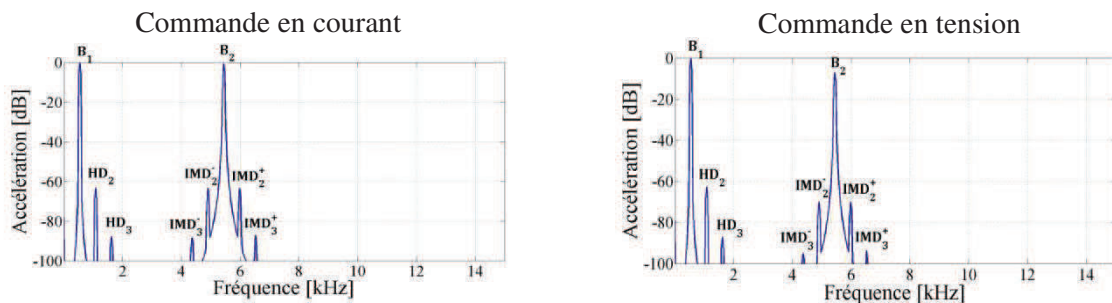
Figure III.49 : Spectre de l'accélération de la référence KLIP lié aux défauts de B_1(x)
