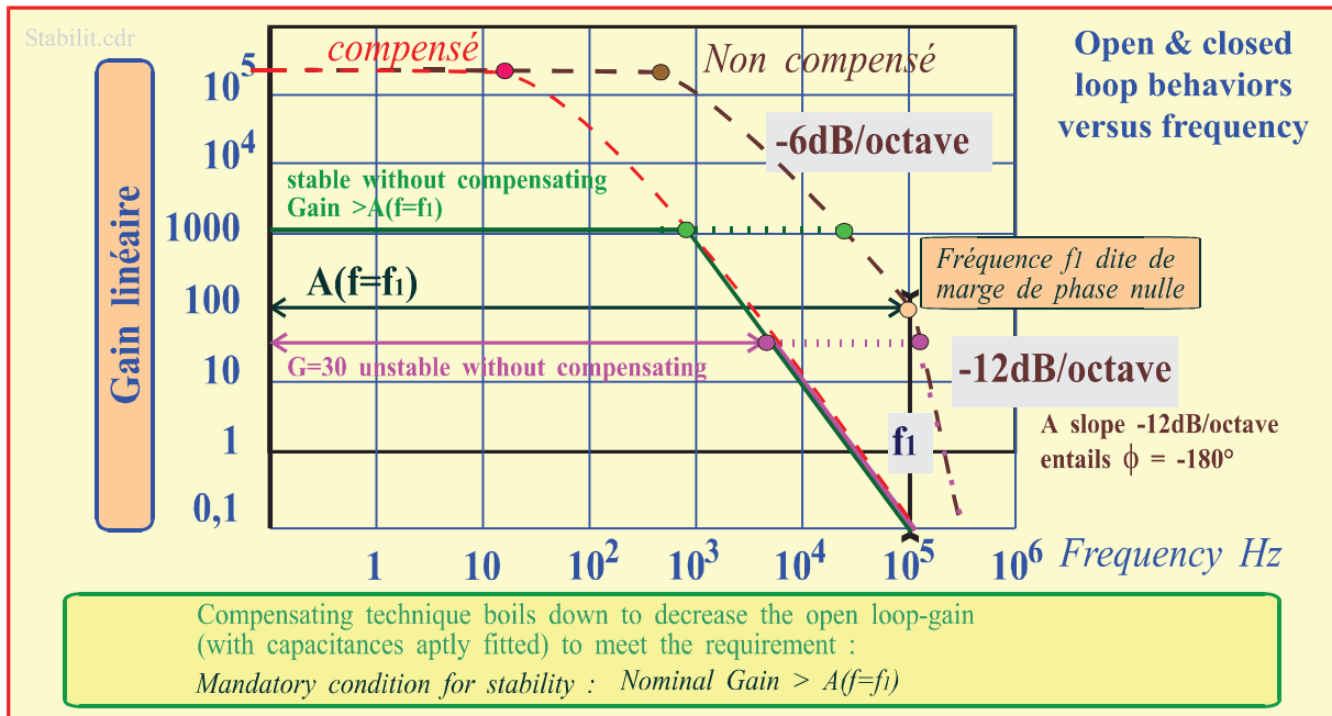
Figure I.21 : Comportement des amplificateurs opérationnels pourvus de compensation
