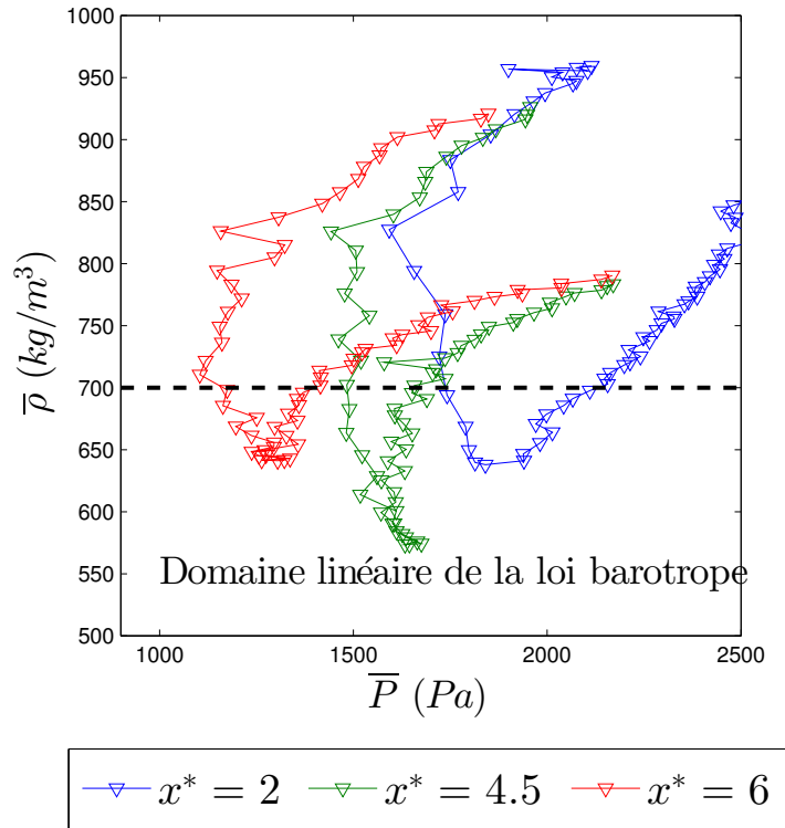
FIGURE 5.26: Masse volumique en fonction de la pression moyenne en cav3
