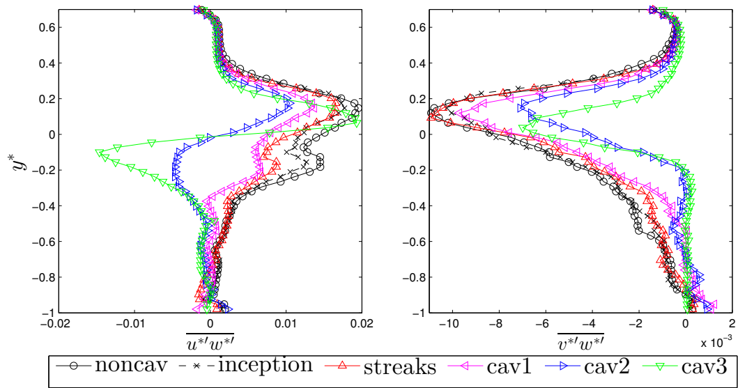
FIGURE 3.38: Profils des contraintes turbulentes \overline{u'^l w'^l} et \overline{v'^l w'^l} dans la zone de transport
