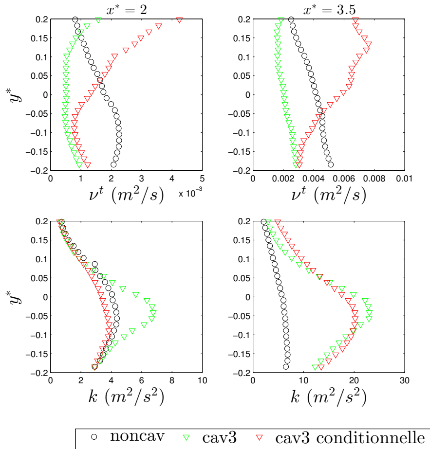
FIGURE 5.23: \nu^t et k en non cavitant, cav3 et cav3 conditionnelle
