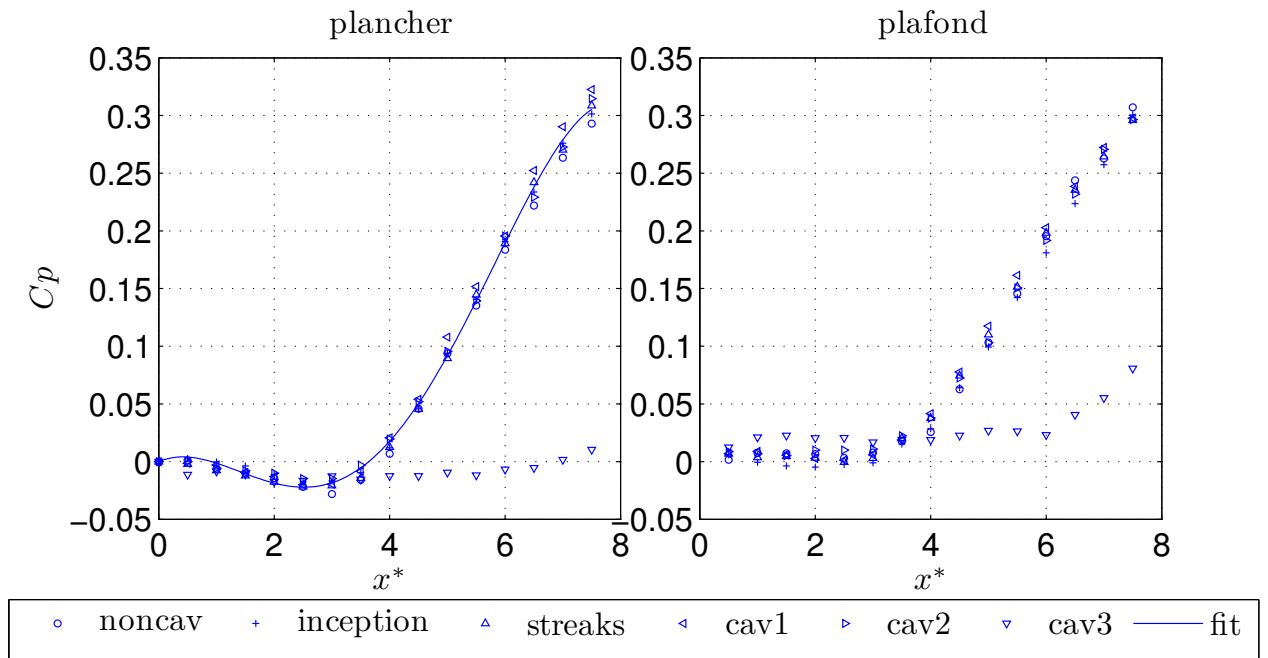
FIGURE 3.14: Coefficient de pression en paroi
