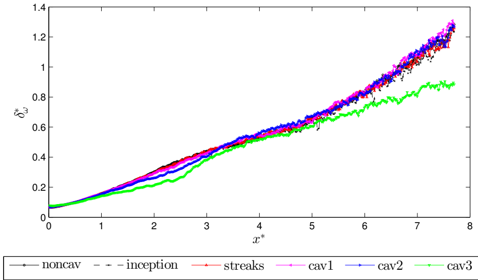
FIGURE 3.27: Évolution de l'épaisseur de vortacité dans l'écoulement
