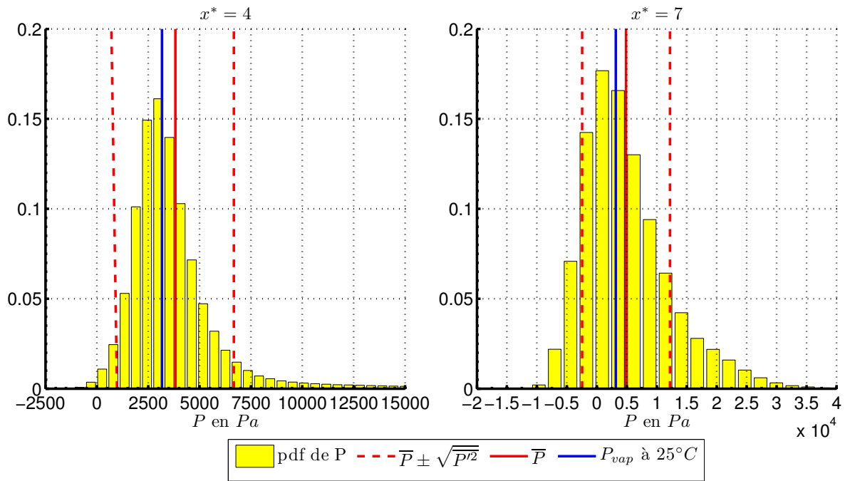
FIGURE 3.19: Densité de probabilité de la pression absolue en x^* = 4 et x^* = 7 pour le cas cav3
