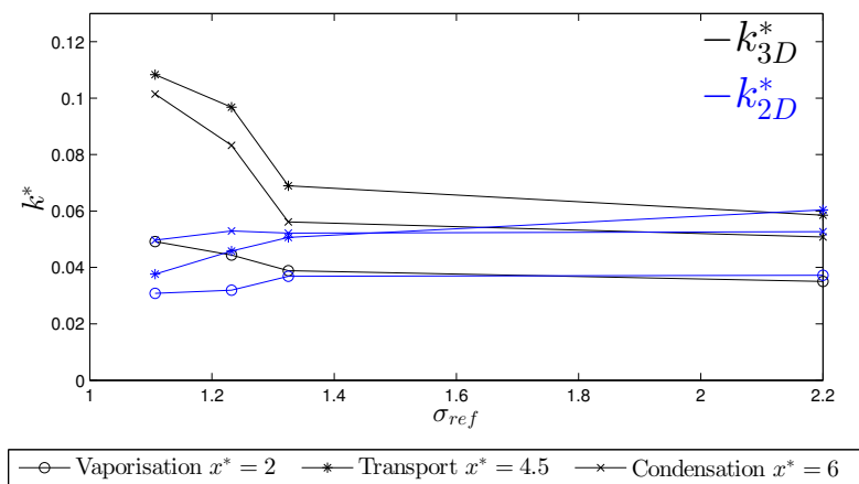
FIGURE 3.36: Évolution de l'énergie cinétique turbulente 3D et 2D
