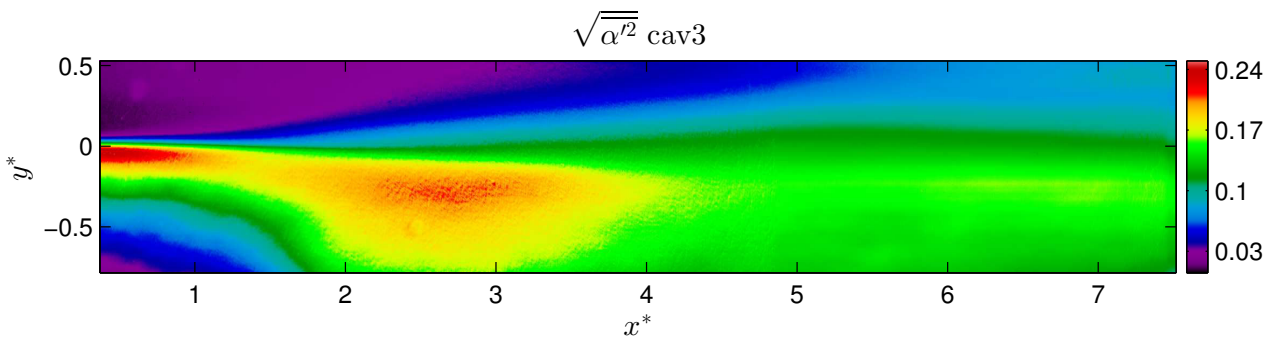
FIGURE 3.10: Écart type de taux de vide en cav3
