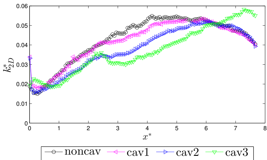
FIGURE 3.33: Évolution du maximum d'énergie cinétique turbulente 2D k_{2D}^* par section
