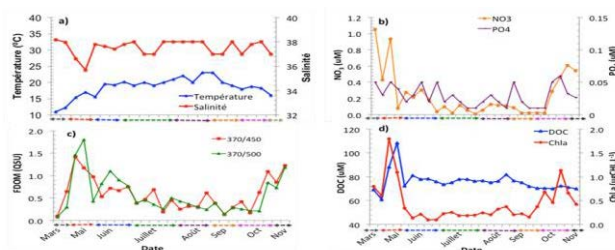
Figure 3. Evolution temporelle de a) Salinité et Température (°C), b) concentrations en nitrate (NO 3 ) et phosphate (PO 4 ) en µM ; c) FDOM (QSU) et d) Chlorophylla a (Chla en µgChL -1 ) et carbone organique dissous (DOC en µM).
