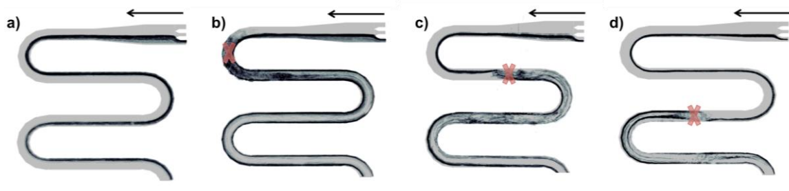
Figure II.22. Mélange de deux phases d'huile selon la Méthode II (billes en suspension dans l'huile, v_{\text{huile}} = 36 \cdot 10^{-6} \text{ m}^2 \cdot \text{s}^{-1} ). Les ultrasons sont focalisés au niveau de la croix rouge en différentes positions (b, c et d) ou désactivés (a).
