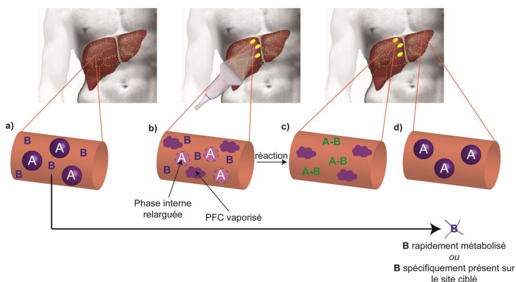
Figure I.35. Principe de la stratégie de chimie in situ : a ) deux partenaires réactionnels A et B sont isolés au moyen de microgouttes de PFC, b ) sur le site à traiter, le produit A encapsulé est libéré sous l'effet des ultrasons, c ) A et B peuvent ainsi réagir pour former le produit actif A-B , d ) hors de la zone focale, le composé A reste encapsulé dans les microgouttes tandis que le partenaire réactionnel B est soit métabolisé, soit spécifiquement présent sur le site à traiter.
