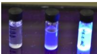
Figure I.19. De gauche à droite (sous illumination UV) : blanc (DMSO pur), coumarine A et produit de la réaction entre A et B .
