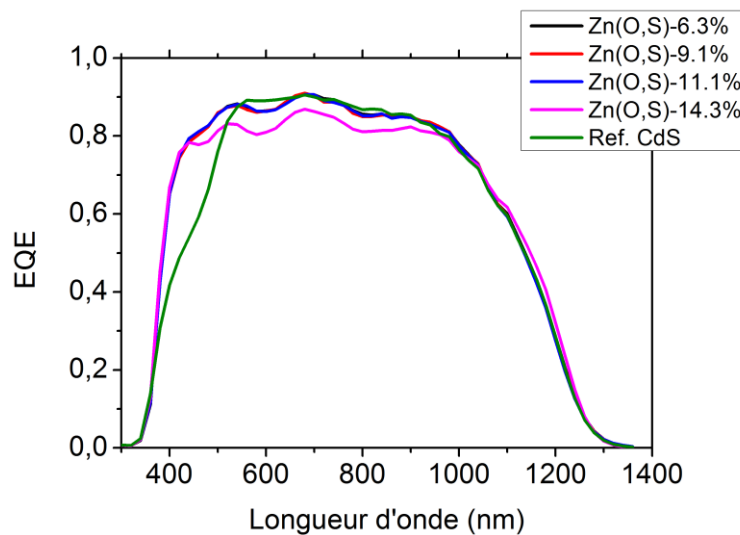
Figure 5.11 Influence du rapport H_2S/(H_2O+H_2S) sur les rendements quantiques externes des cellules CIGS Ed /Zn(O,S).
