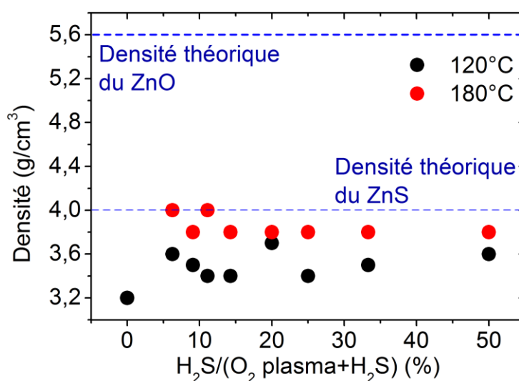
Figure 4.21 Influence du rapport \text{H}_2\text{S}/(\text{O}_2 \text{ plasma} + \text{H}_2\text{S}) sur la densité des couches minces de Zn(O,S) PEALD à T_{\text{dep}} = 120 et 180^\circ\text{C} .
