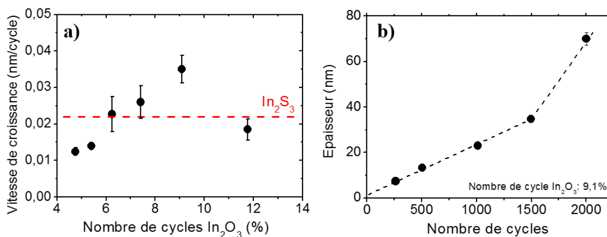
Figure 3.8 Influence du nombre de cycles \text{In}_2\text{O}_3 sur a) la vitesse de croissance des couches minces d' \text{In}_2(\text{S},\text{O})_3 synthétisées par PEALD (la ligne en pointillés rouge est la référence \text{In}_2\text{S}_3 de l'étude) et b) sur l'épaisseur des couches minces (la ligne en pointillés est un guide pour les yeux).
