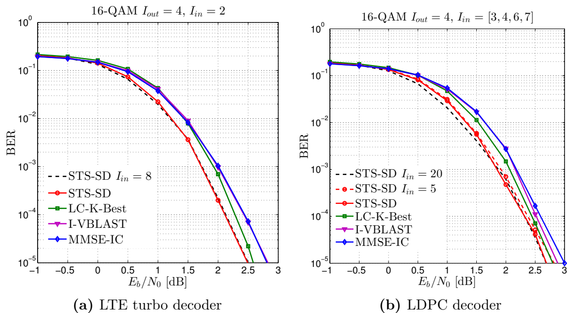
Figure 2: Performances d'un système à multiplexage spatial 4 \times 4 en utilisant différents détecteurs MIMO (STS-SD, LC-K-Best, I-VBLAST and MMSE-IC) dans un canal de Rayleigh, (a) décodeur turbo LTE, K_b = 1,024 , R_c = 1/2 , I_{out} = 4 , I_{in} = 2 , (b) décodeur LDPC N_b = 1,944 , R_c = 1/2 , I_{out} = 4 , I_{in} = [3, 4, 6, 7] .
