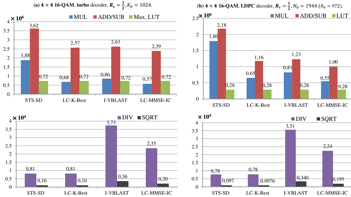
Figure 3: Complexité pour un système de multiplexage spatial 4 \times 4 avec une modulation 16-QAM des différentes techniques de détection avec (a) décodeur turbo, et (b) décodeur LDPC, R_c = 1/2 .
