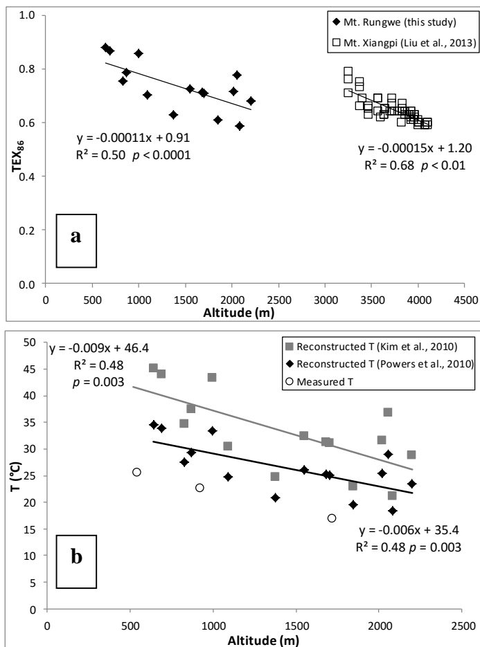
Figure 7 : (a) Variation du TEX_{86} en fonction de l'altitude le long du Mt. Rungwe (losanges) et le long du Mt. Xiangpi (carrés ; Liu et al., 2013) et (b) comparaison des reconstructions de la température de l'air le long du gradient altitudinal du Rungwe à partir de la calibration marine de Kim et al. (2010 ; carrés) et de la calibration lacustre de Powers et al. (2010 ; losanges) avec les TMAA mesurées sur le site par des stations météorologiques fixes (cercles).
