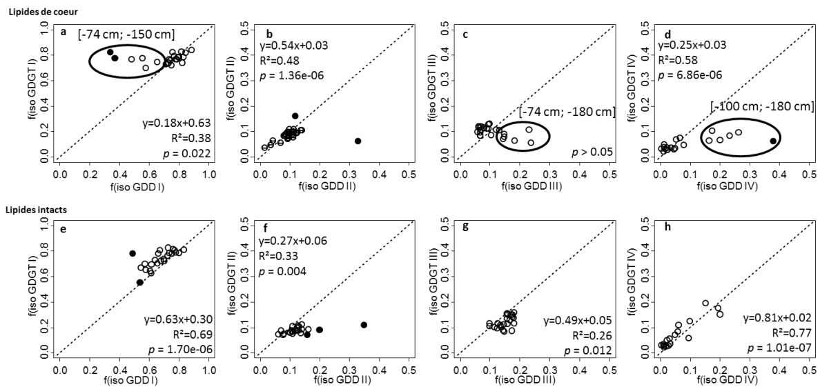
Figure 12 : Corrélation entre l'abondance relative de chaque alkanol diéther avec le tétraéther correspondant pour les composés d'origine bactérienne, sous forme de lipide de cœur (a-d) et lipide intact (e-h). La ligne 1:1 est représentée en pointillés.
