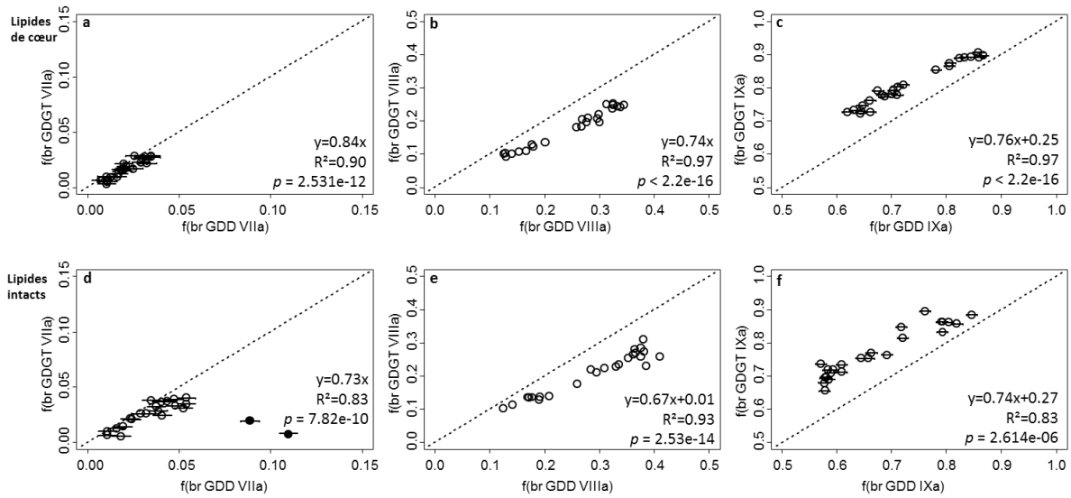
Figure 11 : Corrélation entre l'abondance relative de chaque alkanol diéther avec le tétraéther correspondant pour les composés d'origine bactérienne, sous forme de lipide de cœur (a-c) et lipide intact (d-f). La ligne 1:1 est représentée en pointillés
