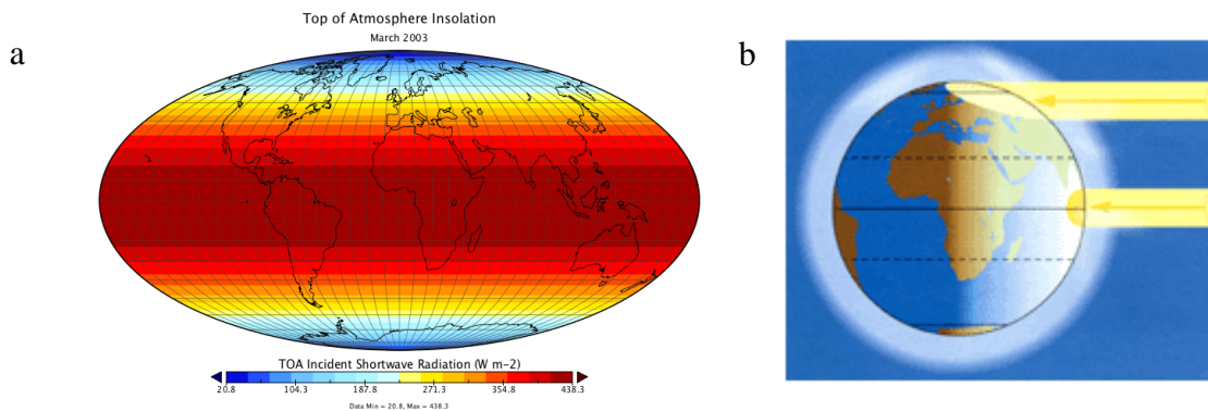
Figure 2 : L'incidence du rayonnement solaire est plus forte à l'équateur qu'aux pôles (a) (échelle 20.8 W/m 2 en bleu à 438.3 W/m 2 en rouge) du fait de la courbure terrestre (b). Source : sites internet du département de géosciences de Penn State (2a) et de l'académie d'Amiens (2b).
