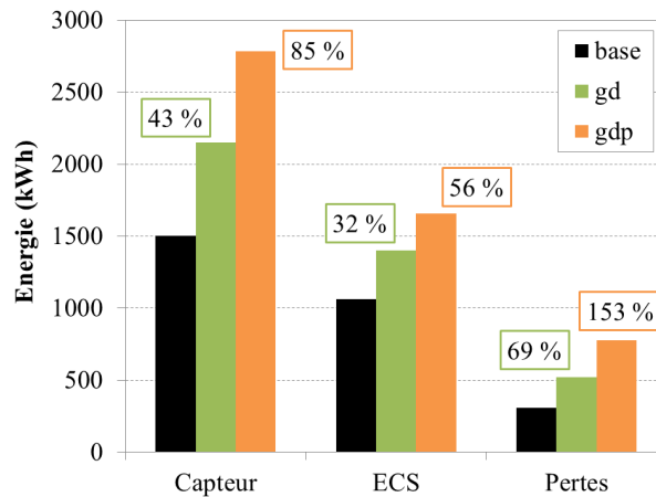
FIGURE 4.13 – Energie annuelle récupérée par le capteur, l'échangeur ECS, et perdue vers l'environnement pour des CSIS de taille différente
