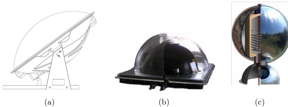
FIGURE 1.6 – CSIS à stockage hémisphérique (a : Nanosol de Ezing et b : CSIS de Solar Energie Stefanakis) et sphérique (c : Sferasol d'Ecozen)
