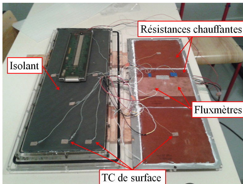
FIGURE B.2 – Installation des différents éléments du bloc de chauffe
