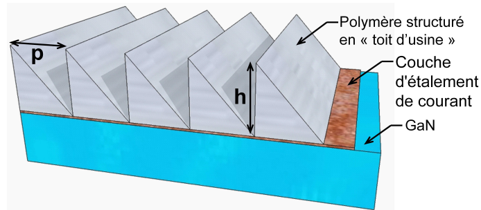
FIGURE 2.1 – Dispositif bio-inspiré de la structure observée chez la luciole. Une diode bleue au nitrure de gallium (GaN) est couverte (par-dessus la couche d'étalement de courant de la diode) d'une couche de polymère structurée à l'échelle micrométrique. Le système a été étudié pour diverses valeurs de la période p du réseau en "toit d'usine", et pour différentes hauteurs h des "toits".
