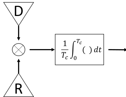
FIGURE 3.7 – Principe de la mesure iGNSS-R.
