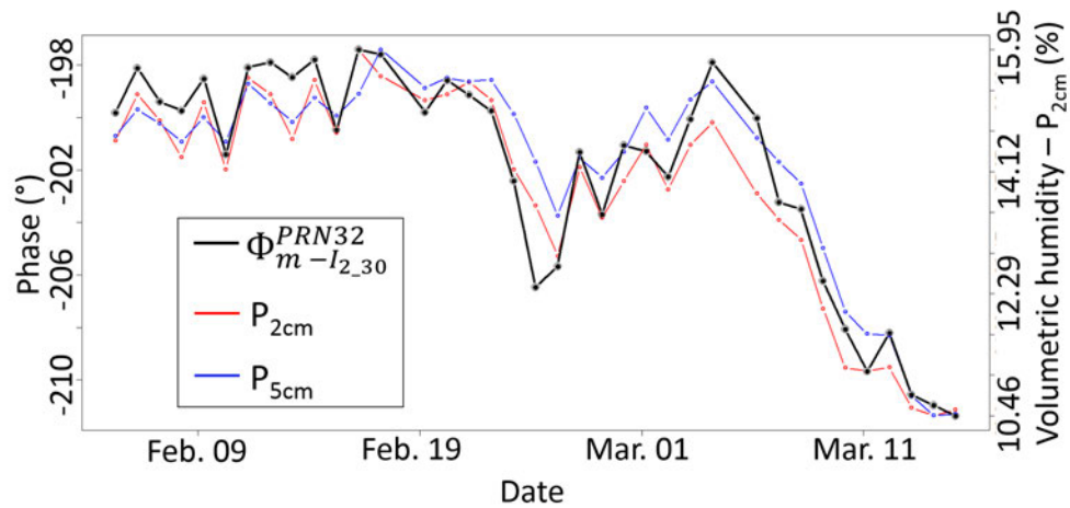
FIGURE 6.6 – Évolution des séries temporelles \phi_{m-I_{2,30}}^{PRN32} , P_{2cm} et P_{5cm} du 5 février au 15 mars 2014.
