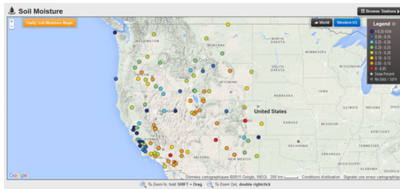
FIGURE 6.1 – Stations GNSS du réseau PBO H2O analysées par réflectométrie pour estimer l'humidité du sol.
