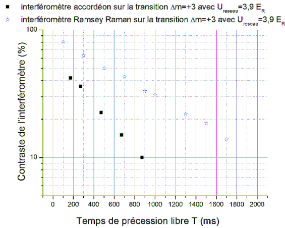
Figure 4.5 : Comparaison du contraste de l'interféromètre accordéon (carrés noirs) et Ramsey Raman (étoiles bleues), pour une transition \Delta m = 3 et à une profondeur de U_{reseau} = 3,9 E_R avec une puissance du laser infrarouge de P_{IR} = 0,5 W .
