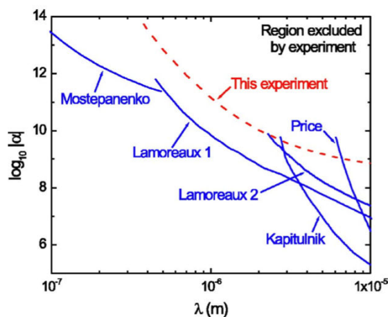
Figure 1.2 : Plan ( \alpha - \lambda ). Les limites Mosepanenko, Kapitulnik et Price viennent des références [Decca et al. , 2005], [Chiaverini et al. , 2003] et [Long et al. , 2003] et la ligne pointillée est le résultat de la première expérience du groupe de E. Cornell dont est tiré ce graphe [Harber et al. , 2005].
