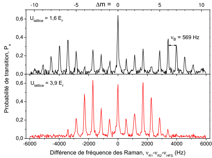
Figure 1.14 : Probabilité de transition P_e lors d'une transition Raman en fonction du désaccord \nu_{Ram} , centré sur \nu_{HFS} . Les résonances des états de Wannier Stark sont séparées de \nu_B . Les hauteurs relatives entre les différents pics nous renseignent sur la profondeur du réseau. Tiré de [Pelle, 2013].
