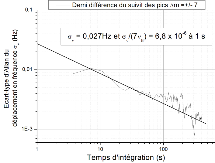
Figure 3.15 : Écart type d'Allan des fluctuations temporelles de fréquence de la spectroscopie Raman fine. Paramètres : \Delta m = 7 , U_{reseau} = 1,6 E_R , P_{IR} = 0,5 W , \tau_{Ram} = 900 s , \Omega_{\Delta m = \pm 7} \times \tau_{Ram} = \pi , désaccord Raman 300 GHz.
