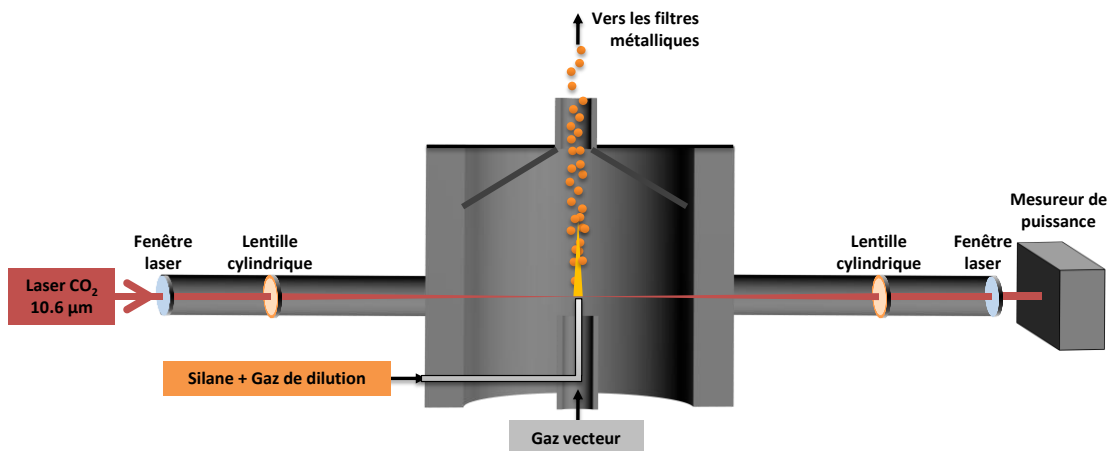
Figure II.9. Schéma du réacteur en configuration simple étage
