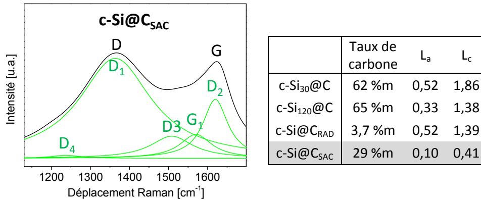
Figure IV.51. Déconvolution des bandes D et G et calcul des rapports L_a et L_c sur l'échantillon c-Si@C SAC
