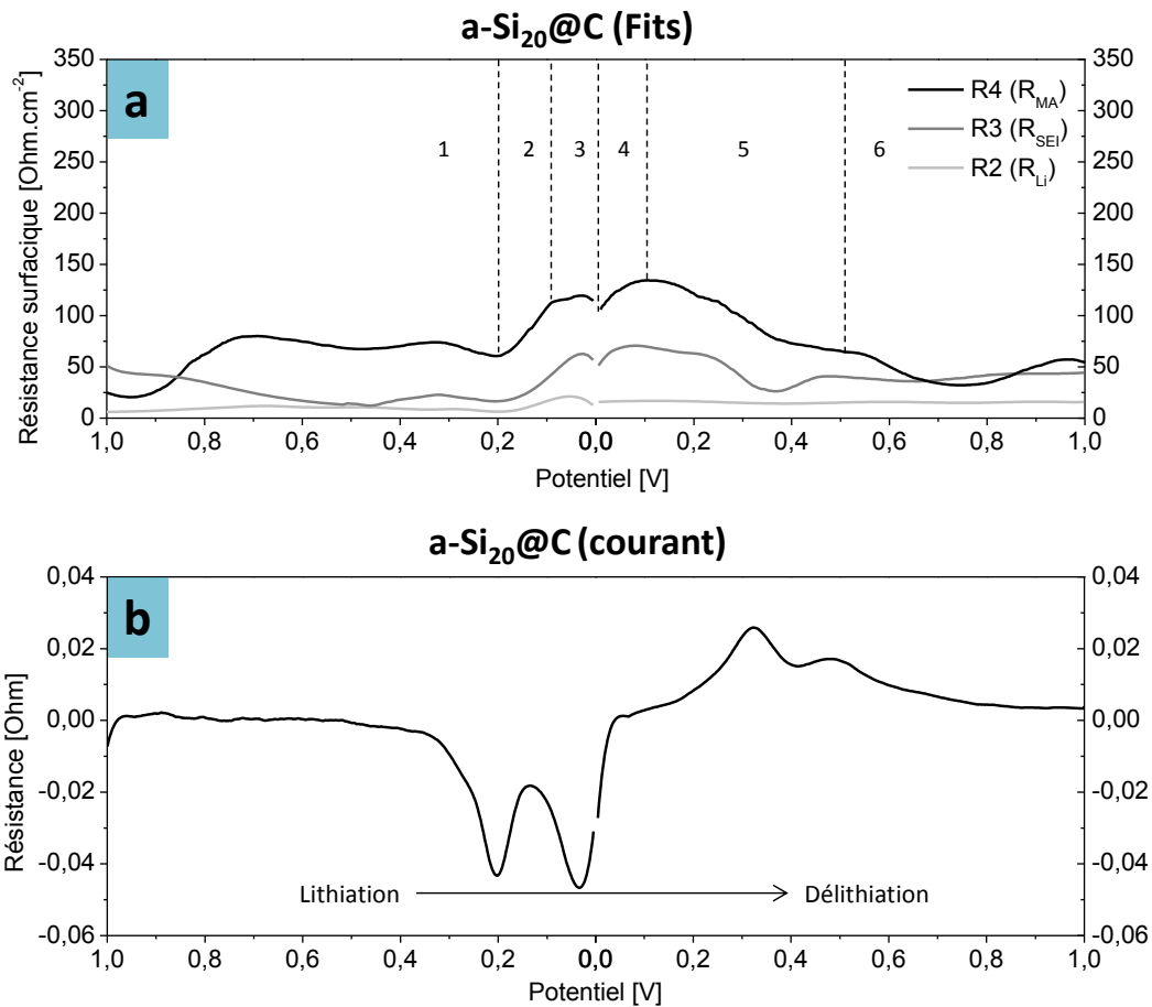
Figure V.24. Evolution des variables R2, R3 et R4 sur les spectres SIE de a-Si 20 @C (a) et évolution du courant (b)
