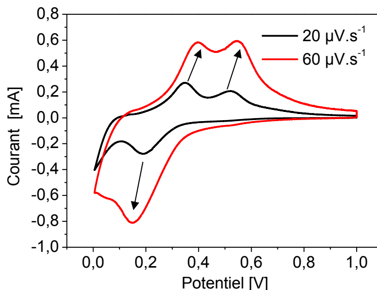
Figure V.1. Exemple de voltamogrammes obtenus sur c-Si 30 à 20 et 60 \mu\text{V}\cdot\text{s}^{-1} (soit 72 et 216 \text{mV}\cdot\text{h}^{-1} )
