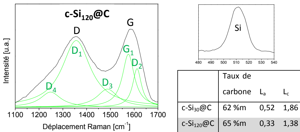
Figure IV.21. Déconvolution des bandes D et G de l'échantillon c\text{-Si}_{120}\text{@C} et calcul des dimensions L_a et L_c
