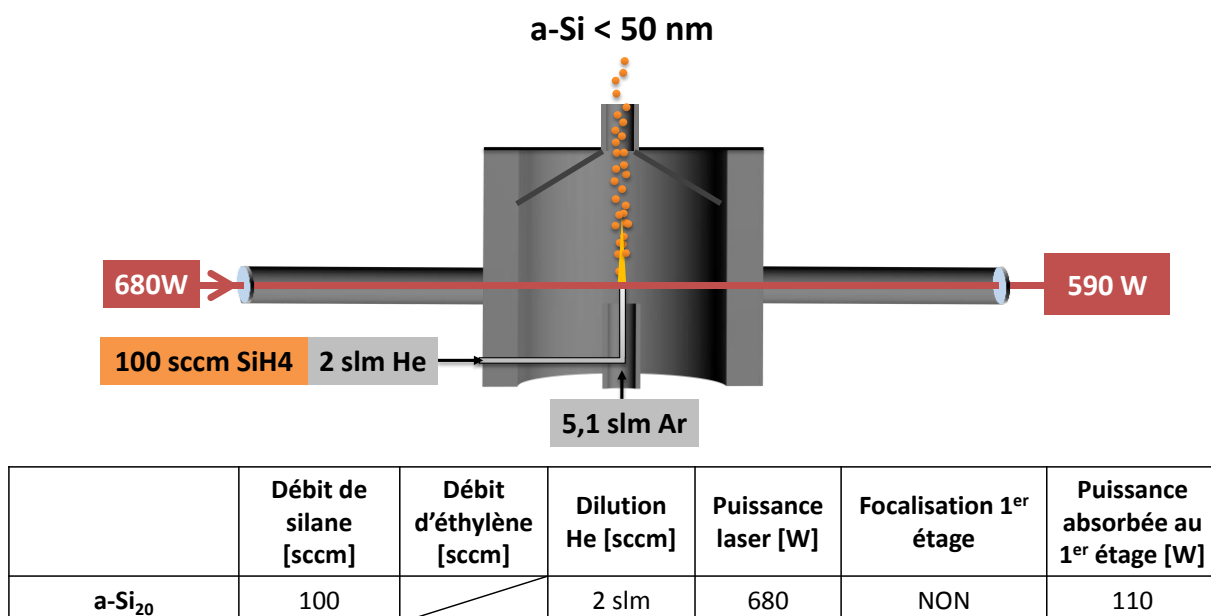
Figure IV.33. Schéma représentant les conditions de synthèse de nanoparticules de silicium amorphes a-Si 20
