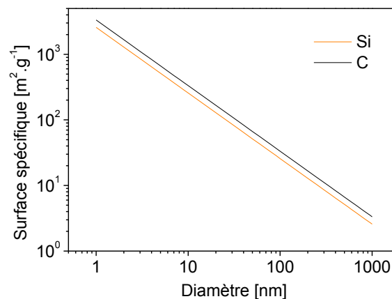
Figure III.2. Relation logarithmique entre le diamètre des nanoparticules et la surface spécifique
