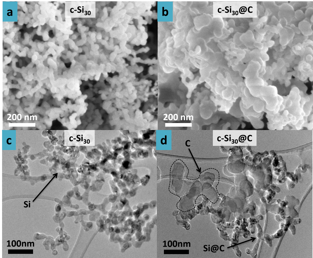
Figure IV.11. Clichés MEB (a,b) et MET (c,d) des matériaux c\text{-Si}_{30} et c\text{-Si}_{30}\text{@C}
