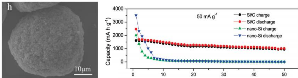
Figure I.22. Cliché MET et performance électrochimique (tracés rouge et noir) de nanoparticules de silicium contenues dans un composite microporeux carboné, d'après Yin 139
