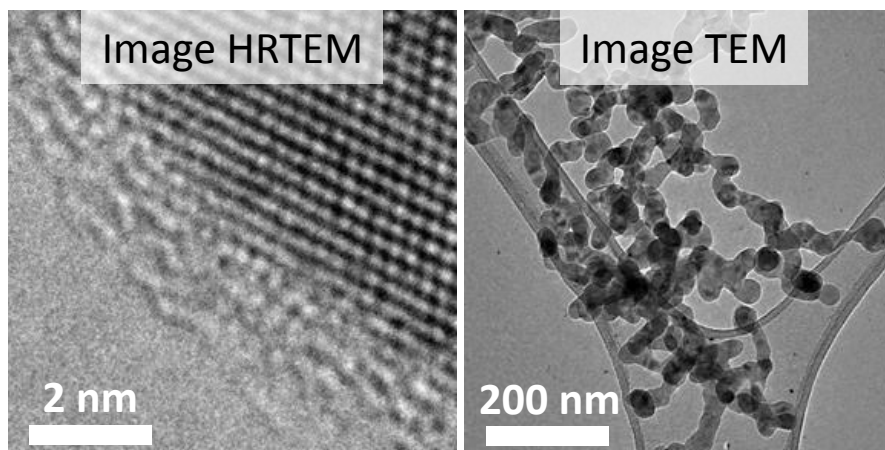
Figure III.14. Comparaison d'un cliché METHR et d'un cliché MET
