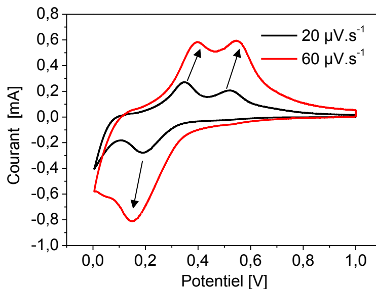
Figure V.1. Exemple de voltamogrammes obtenus sur c-Si 30 à 20 et 60 µV.s -1 (soit 72 et 216 mV.h -1 )
