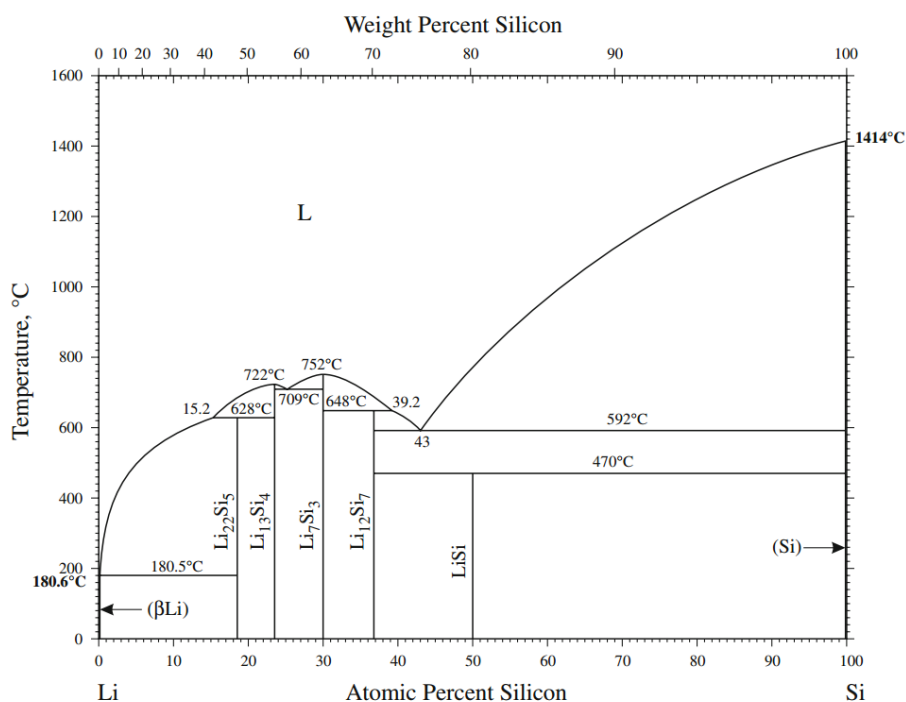
Figure 1.6. Diagramme de phase Li-Si, d'après Okamoto 74
