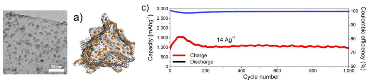
Figure I.25. Nanoparticules de silicium, synthétisées par CVD, enveloppées dans des feuillets de graphène, d'après J. Cho 142
