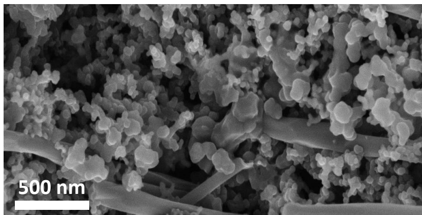
Figure III.13. Image MEB de la tranche d'une électrode non cyclée
