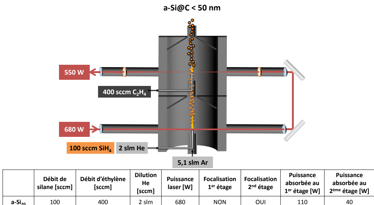
Figure IV.38. Schéma représentant les conditions de synthèse de nanoparticules de silicium amorphes a\text{-Si}_{20}\text{@C}
