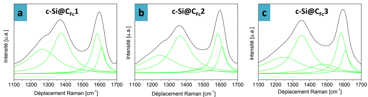
Figure IV.32. Déconvolution des bandes D et G et calcul des rapports L_a et L_c sur les échantillons c\text{-Si@C}_{F_c}
