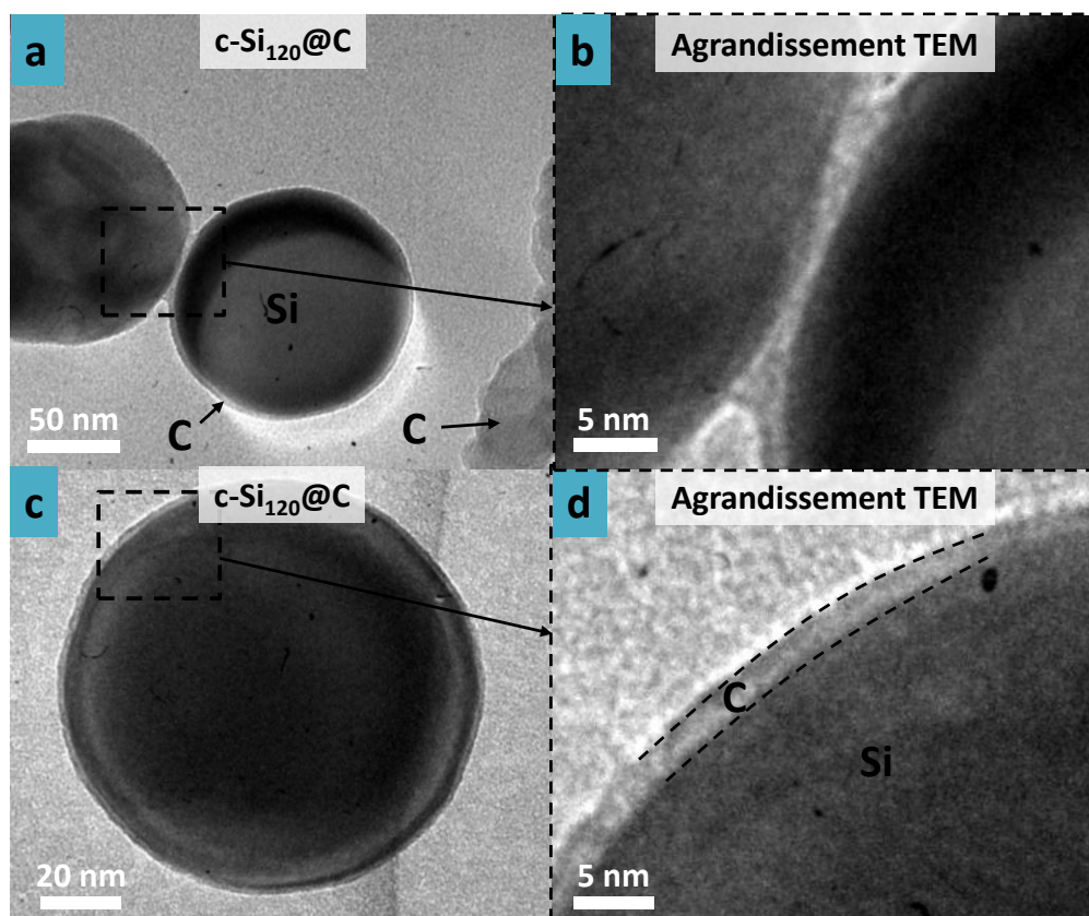
Figure IV.20. Cliché MET de c-Si 120 @C (a,c) et agrandissement respectif (b,d).
