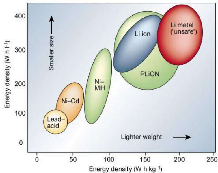
Figure 2. Principales technologies pour le stockage électrochimique d'énergie dans le diagramme de Ragone, d'après Tarascon et Armand 5
